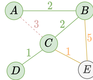
(d) Už nám zbývá pouze vrchol E . Máme na výběr mezi vahami 1 a 5. Vybereme nejlehčí 1 a dostaneme výslednou minimální kostru.
