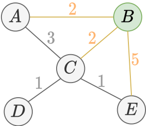
(a) Začneme v B , máme tři možnosti: A, C, E s vahami 2, 2, 5. Vybereme libovolnou nejlehčí, například 2 do A .
