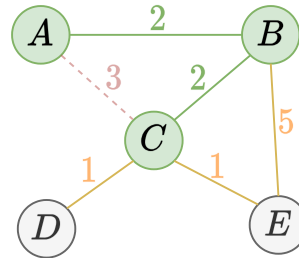
(b) Nyní se můžeme vydat do C/E s vahami 3, 2, 5. Vybereme nejlehčí, tedy 2.
