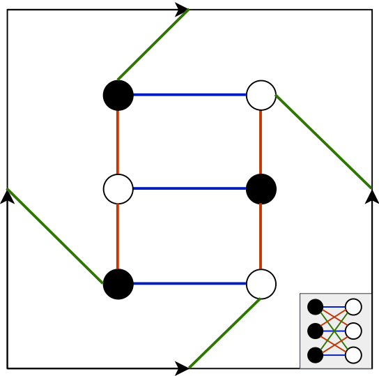
K_{3,3} na torus
