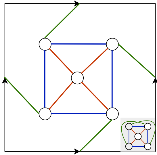
K_5 na torus
