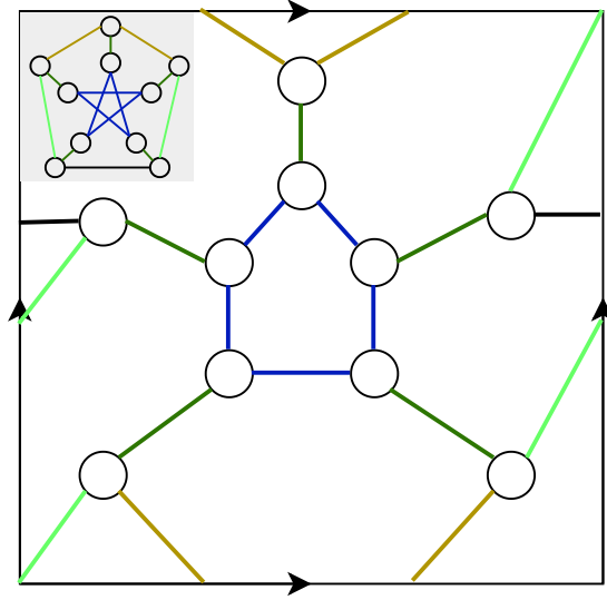
Peterson na torus
