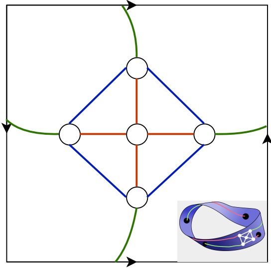
K_5 v projektivní rovině
