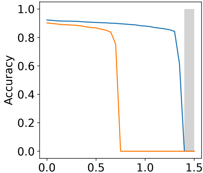
CIFAR-2
