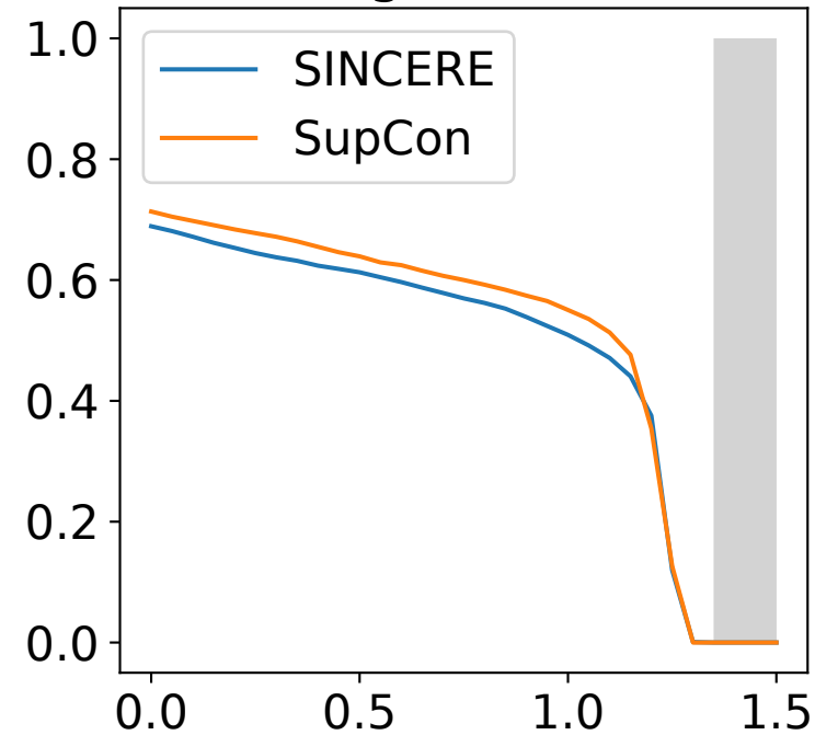
ImageNet-100
