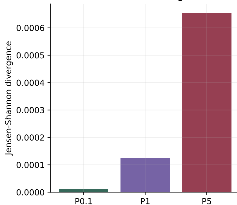
SMILES-token divergence
