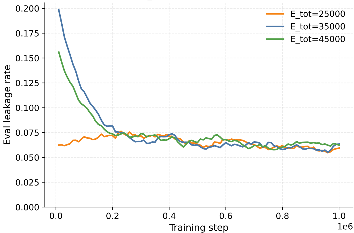
E_tot: Eval Leakage Rate
