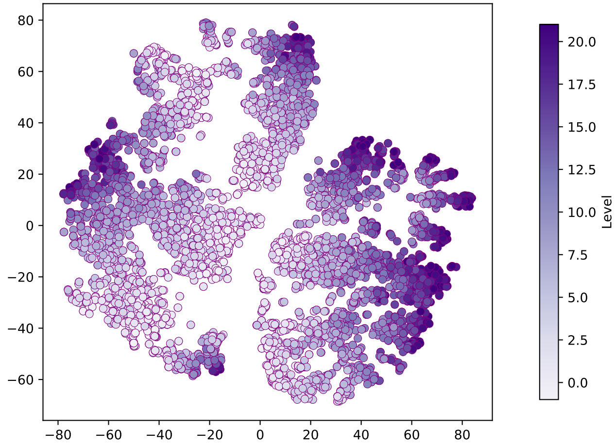
TSNE
