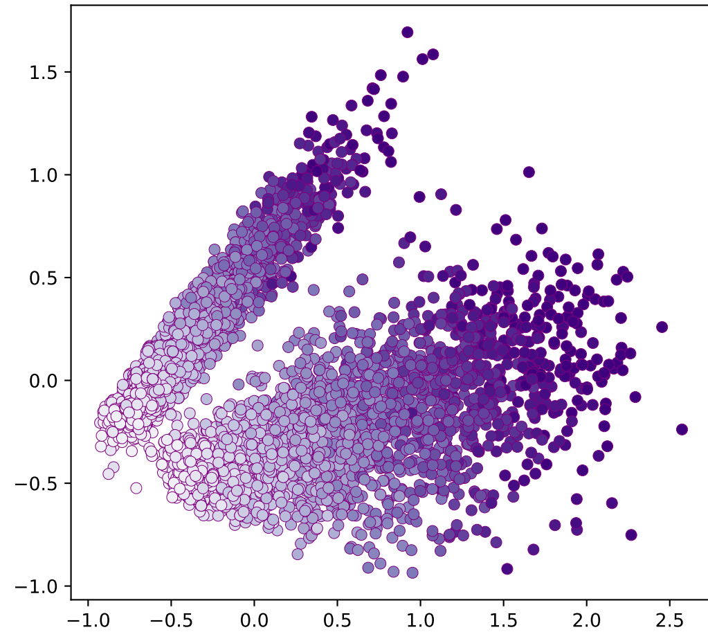
PCA
