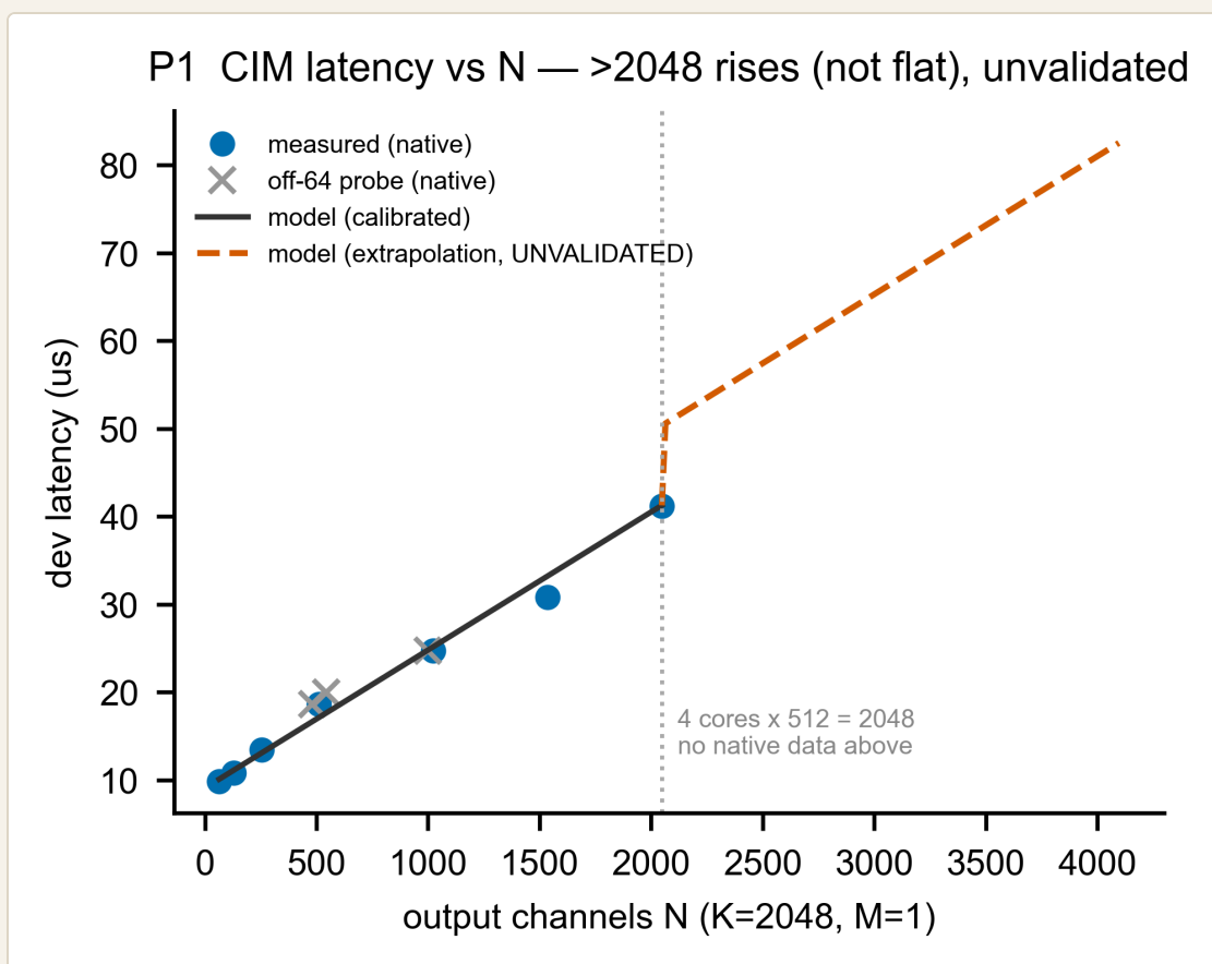
圖 A1-1（P1）— 延遲 vs N（K=2048）：原生 + 外推
