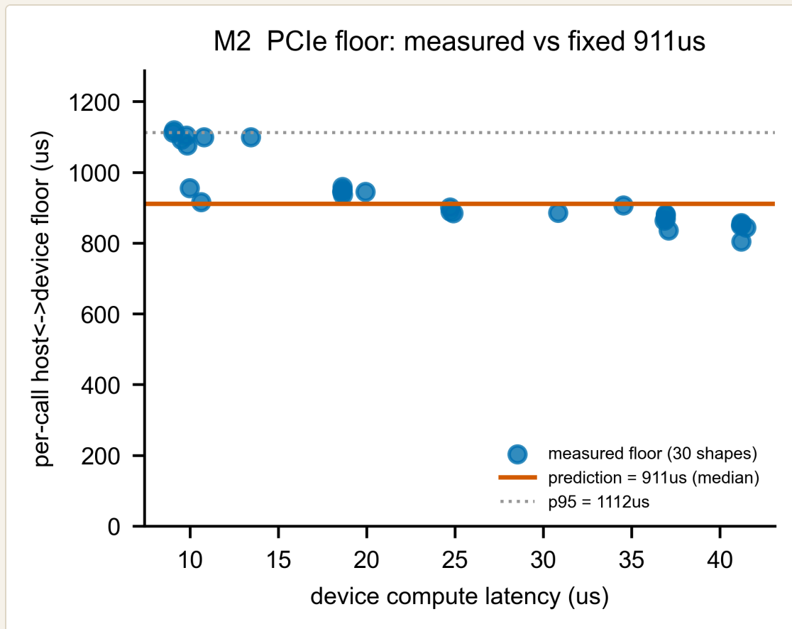
圖 A2-1 (M2 PCIe floor) — 量測的 floor vs 固定 911\mu\text{s} 預測
