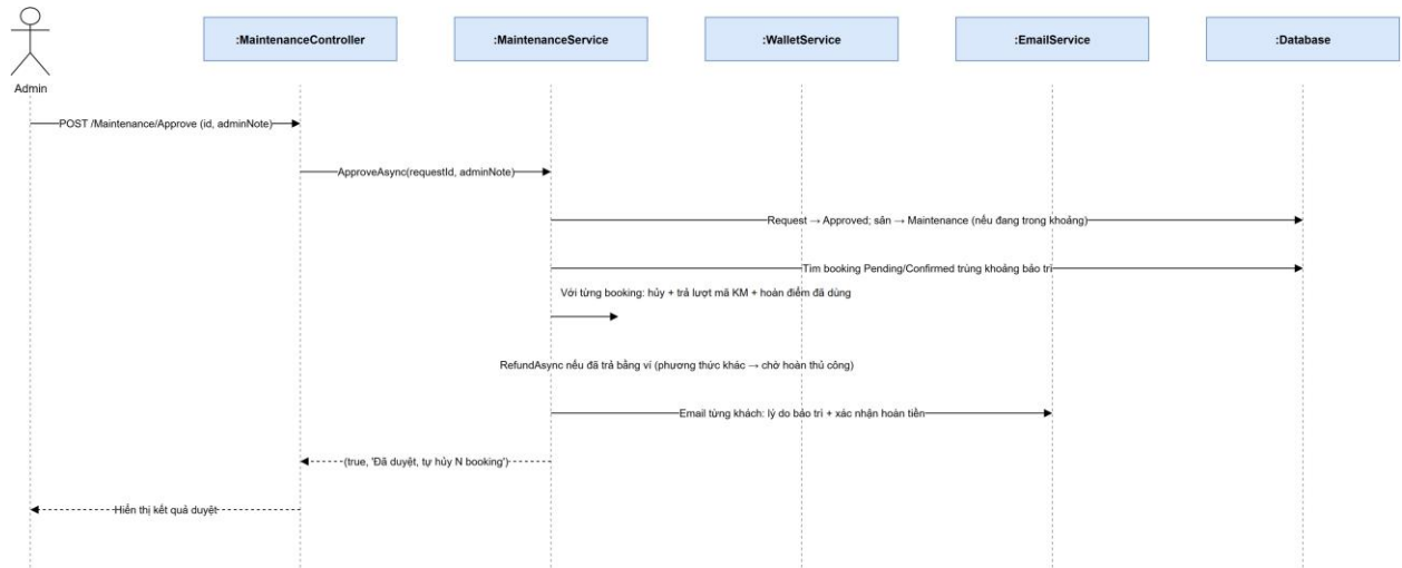
Hình 3.5 - Sequence Diagram: Duyệt bảo trì
