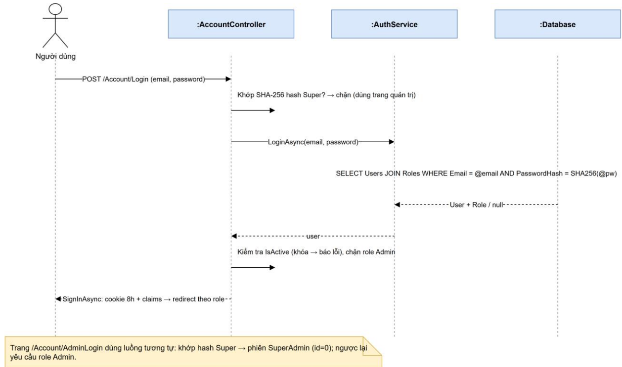
Hình 3.1 - Sequence Diagram: Đăng nhập
