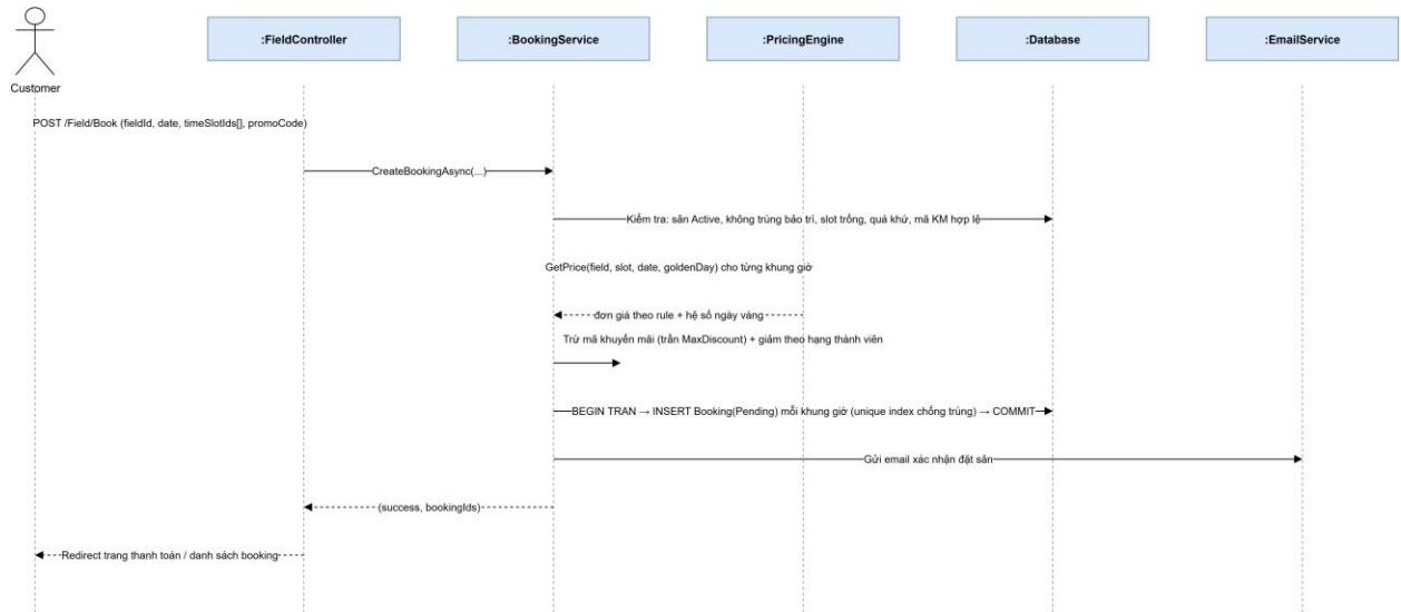
Hình 3.2 - Sequence Diagram: Đặt sân
