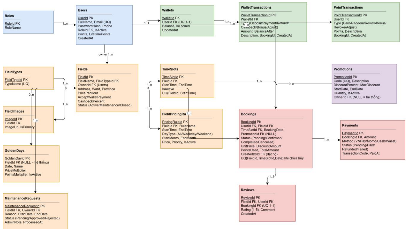
Hình 1.3.1 - ERD
