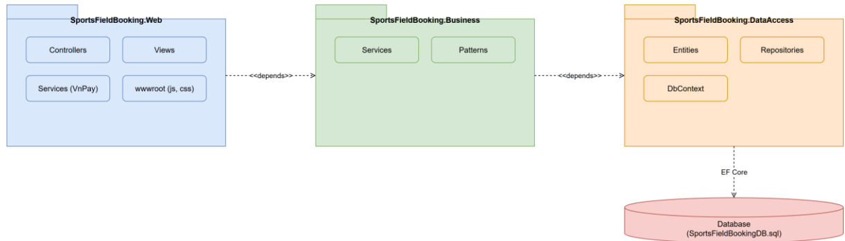
Hình 1.2 - Package Diagram
