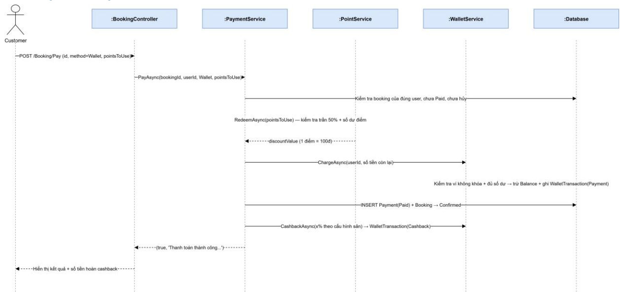
Hình 3.3 - Sequence Diagram: Thanh toán bằng ví
