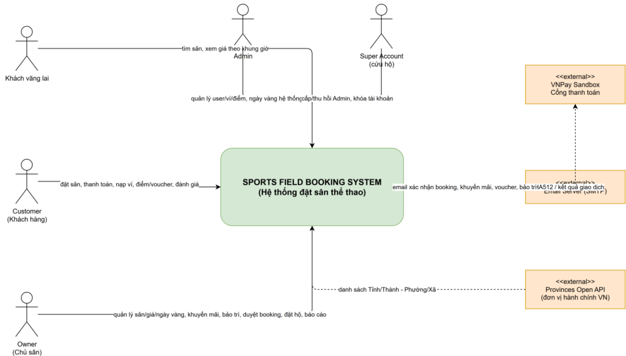
Hình 1.1 - Context Diagram
