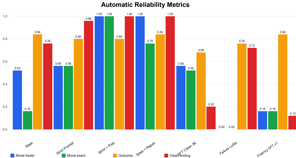
Hình 23: E4: độ tin cậy tự động của bảy cấu hình trên cùng 25 đề bài nội bộ. Các chỉ số phản ánh hợp đồng đầu ra và độ phủ, không thay thế đánh giá ngữ nghĩa của con người.
