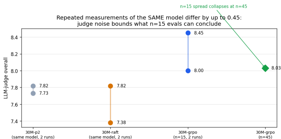
Hình 10: Độ biến thiên khi chấm lặp cùng checkpoint và ảnh hưởng của cỡ mẫu.
