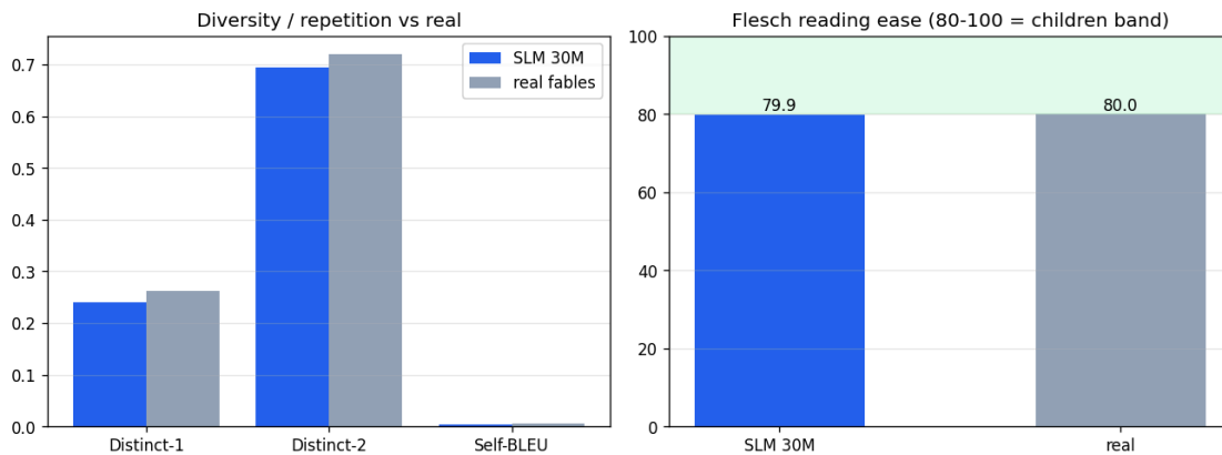
Hình 7: Đa dạng, mức lặp và độ dễ đọc của truyện sinh so với truyện thật.
