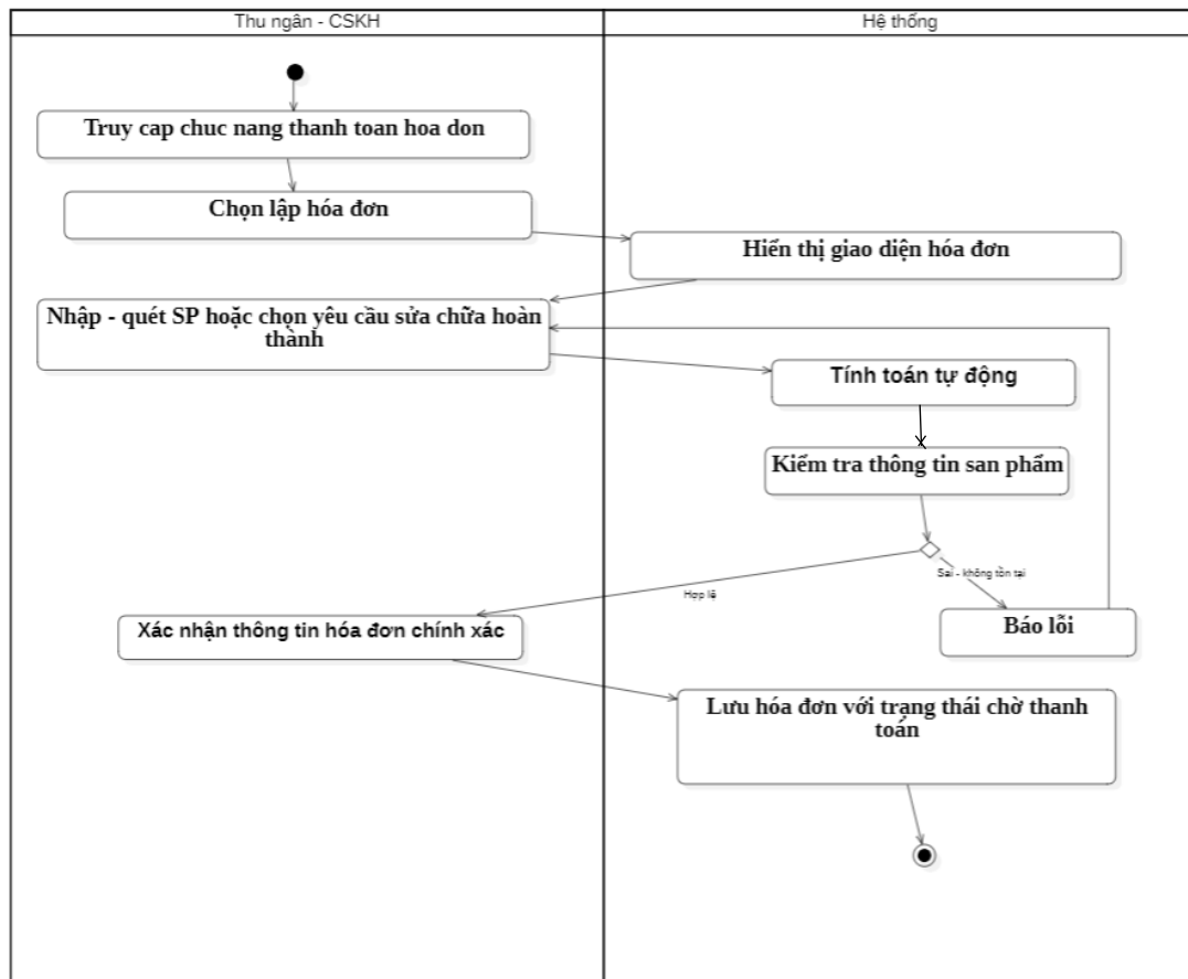
Biểu đồ hoạt động của Usecase “Lập hóa đơn”
