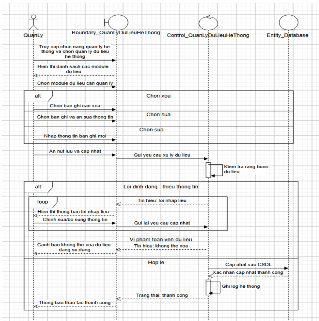
Biểu đồ tuần tự của Usecase “Quản lý dữ liệu hệ thống”
