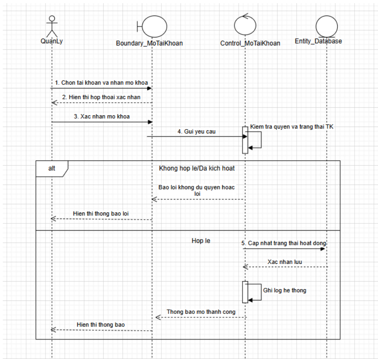
Biểu đồ tuần tự của Usecase “Mở tài khoản”
