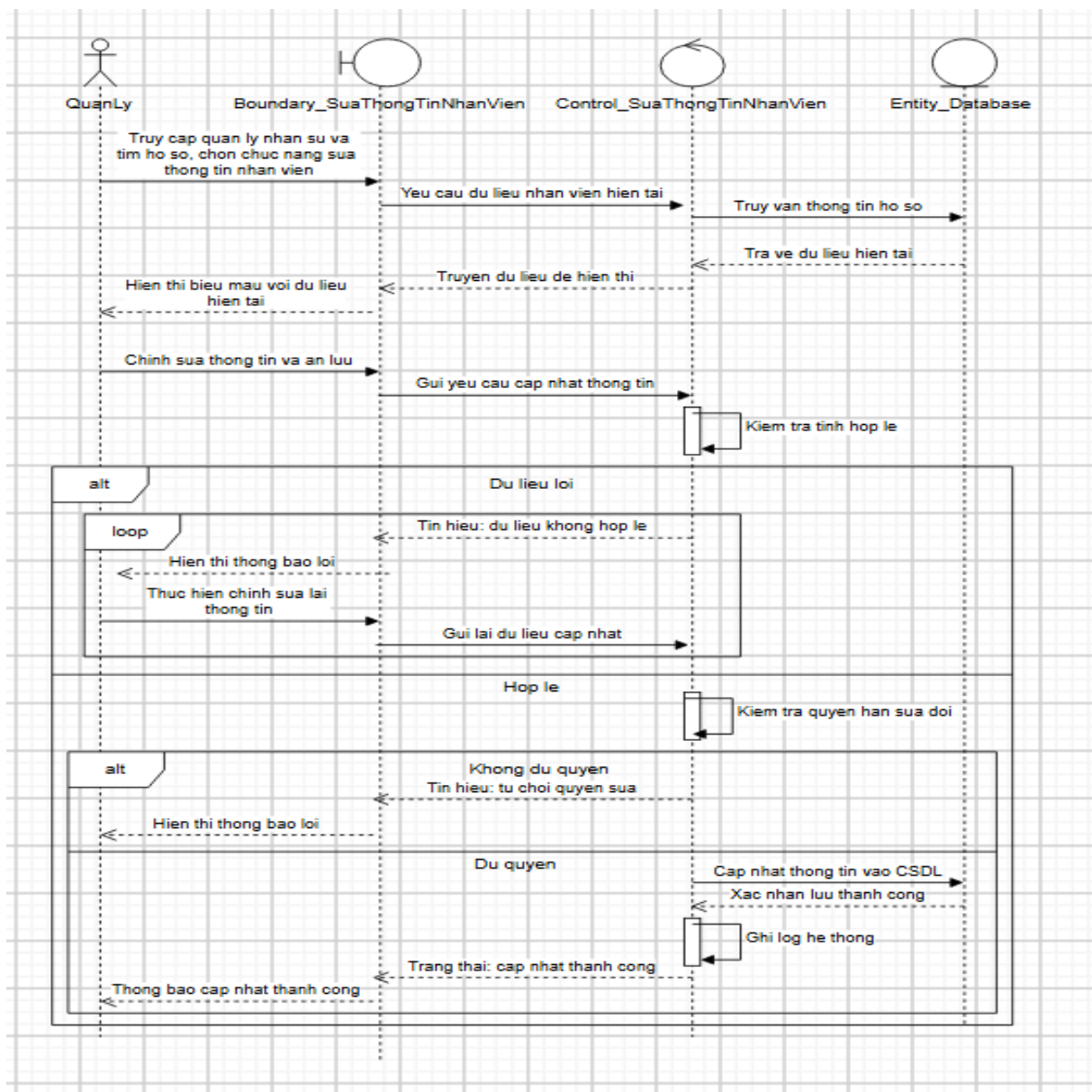
Biểu đồ tuần tự của Usecase “Sửa thông tin nhân viên”
