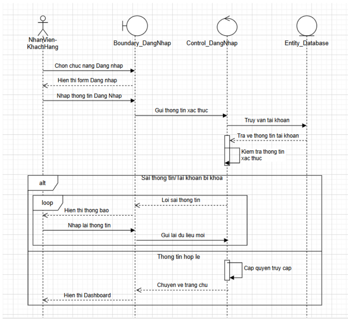
Biểu đồ tuần tự của Usecase “Đăng nhập”
