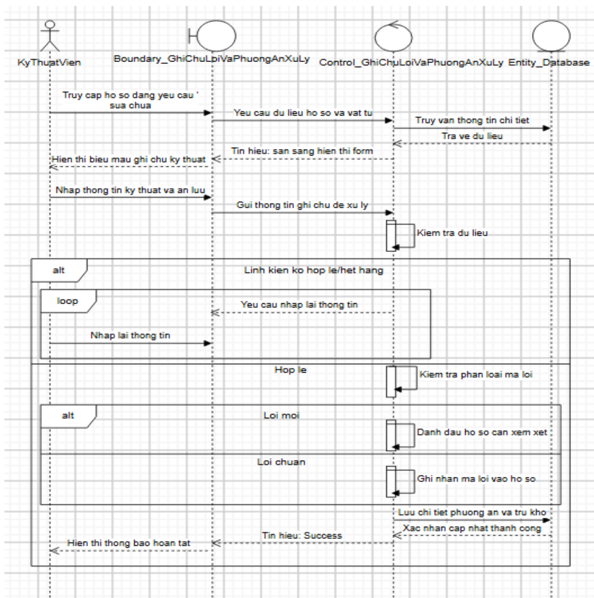
Biểu đồ tuần tự của Usecase “Ghi chú lỗi và phương án xử lý”
