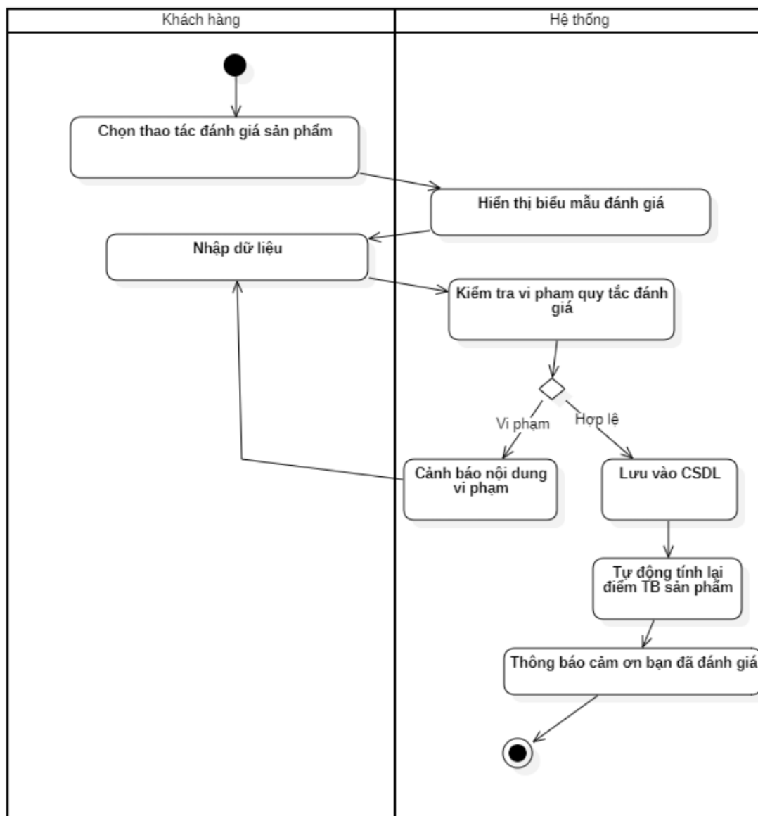
Biểu đồ hoạt động của Usecase “Đánh giá sản phẩm”
