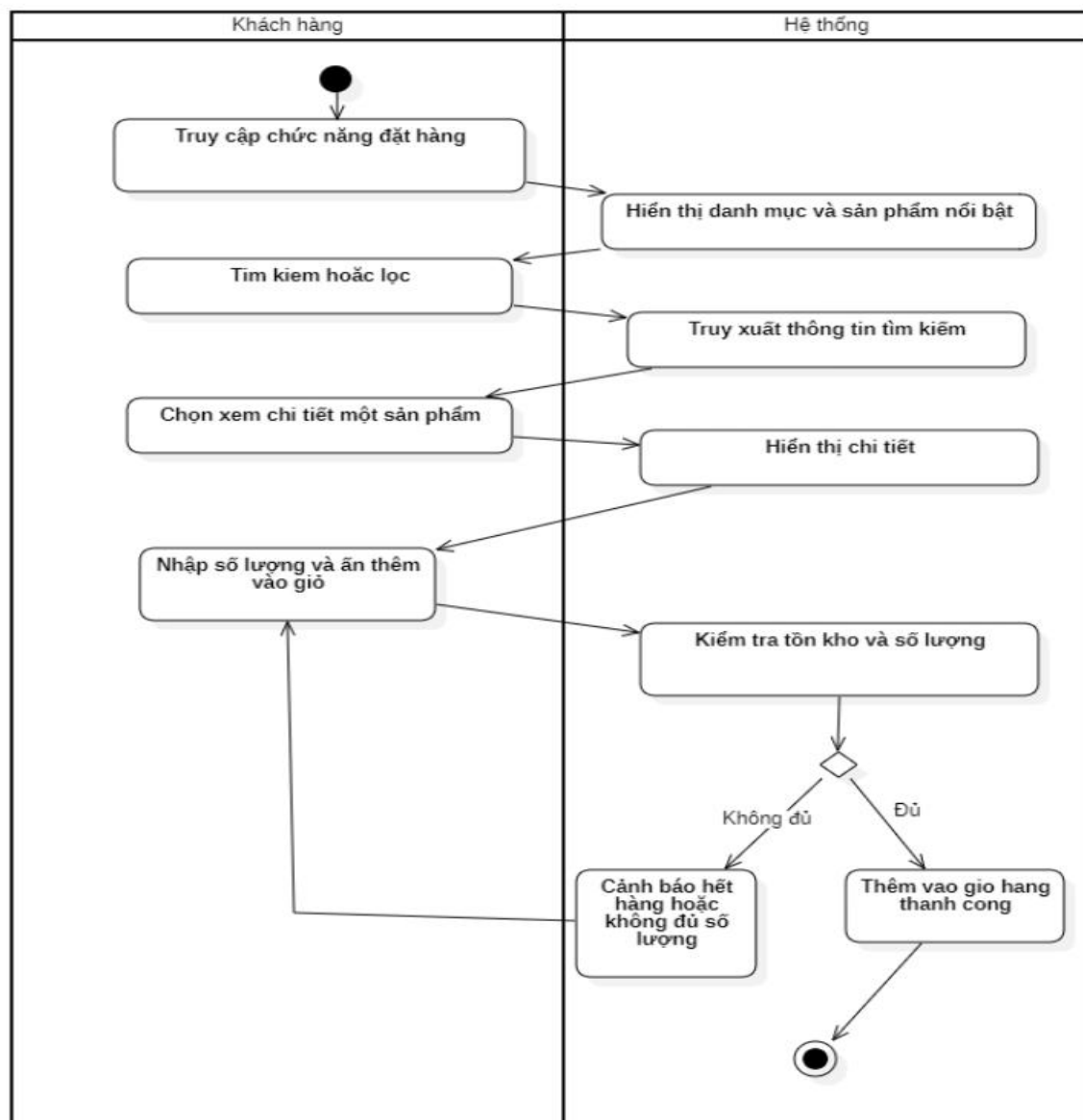
Biểu đồ hoạt động của Usecase “Chọn sản phẩm”
