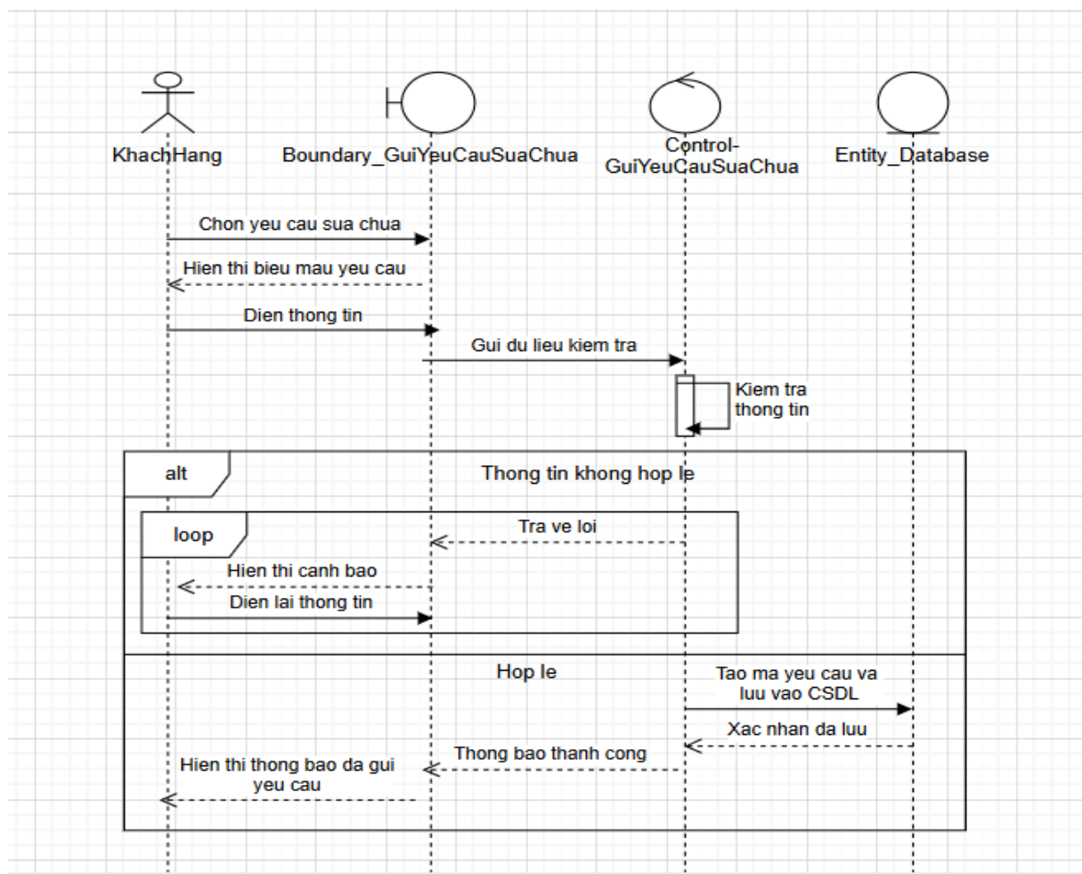
Biểu đồ tuần tự của Usecase “Gửi yêu cầu sửa chữa”
