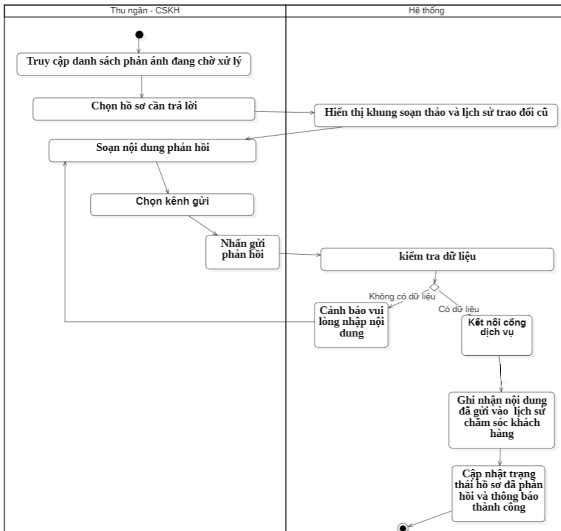
Biểu đồ hoạt động của Usecase “Gửi phản hồi cho khách”
