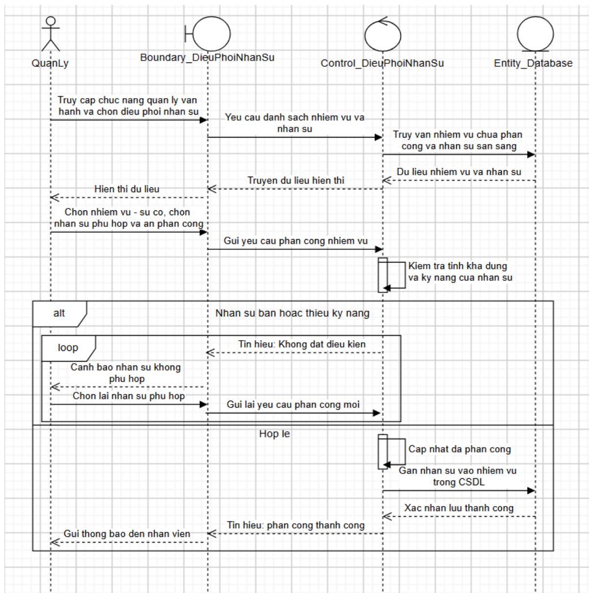
Biểu đồ tuần tự của Usecase “Điều phối nhân sự”
