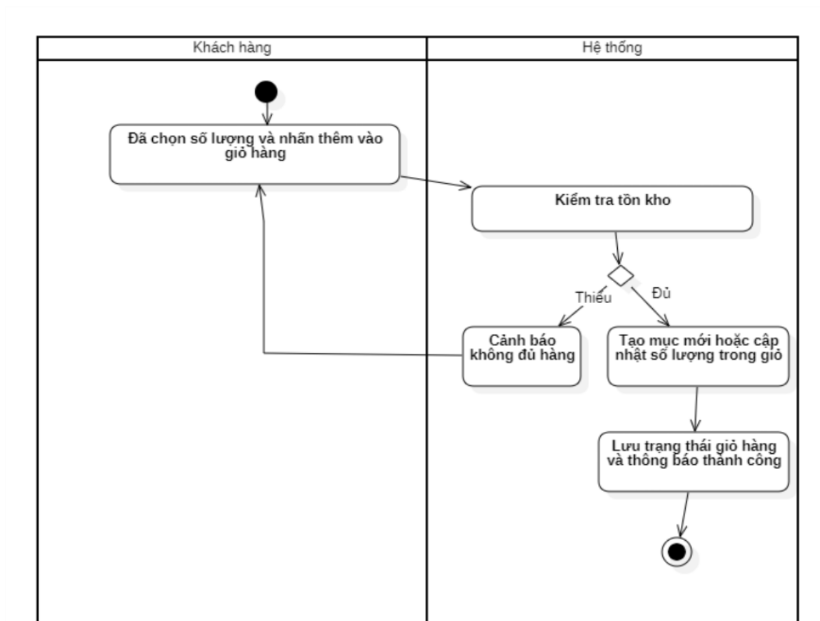
Usecase “Thêm vào giỏ hàng”
