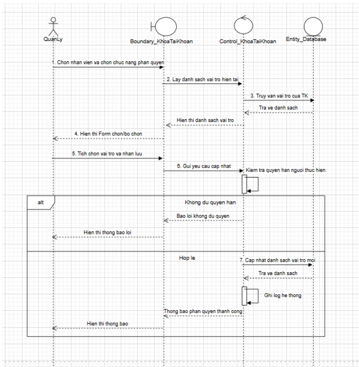
Biểu đồ tuần tự của Usecase “Phân quyền tài khoản”
