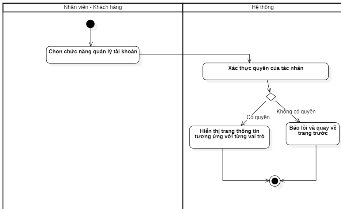
Biểu đồ hoạt động của Usecase “Quản lý tài khoản”
