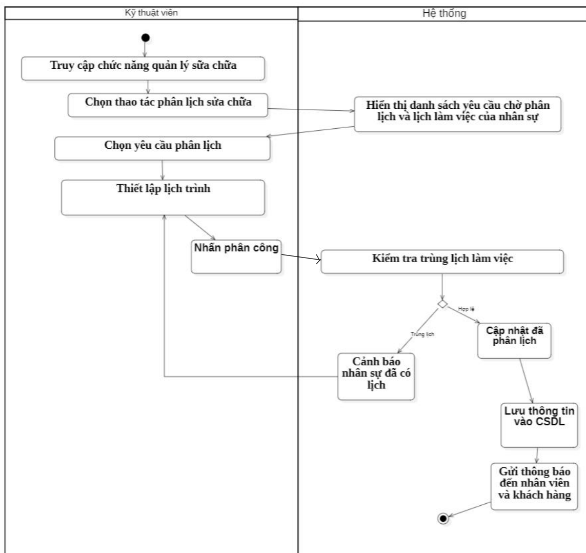
Biểu đồ hoạt động của Usecase “Phân lịch sửa chữa”
