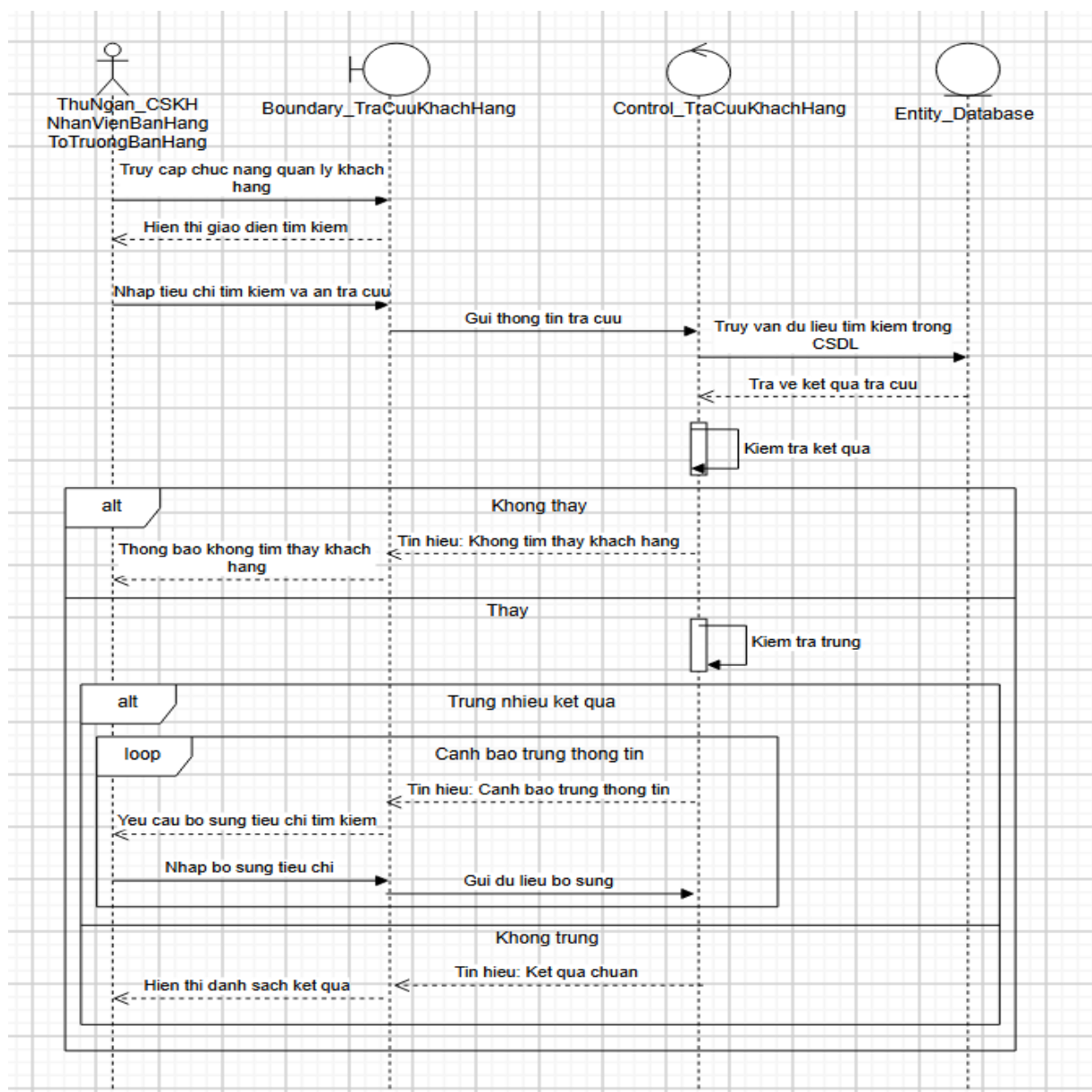
Biểu đồ tuần tự của Usecase “Tra cứu khách hàng”
