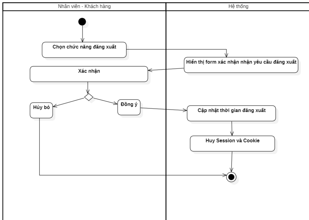
Biểu đồ hoạt động của Usecase “Đăng xuất”
