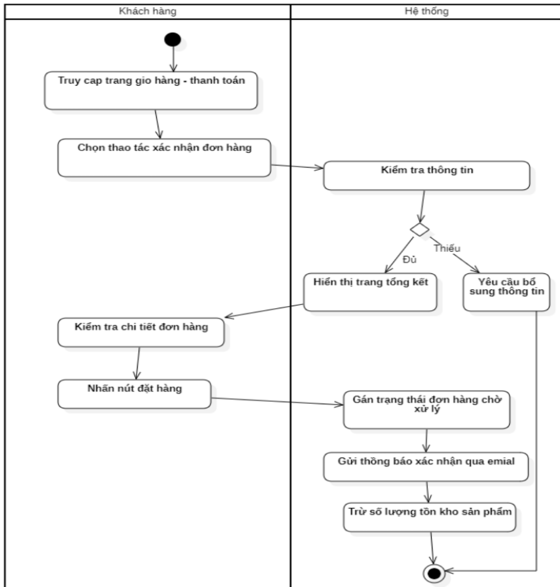
Biểu đồ hoạt động của Usecase “Xác nhận đơn hàng”
