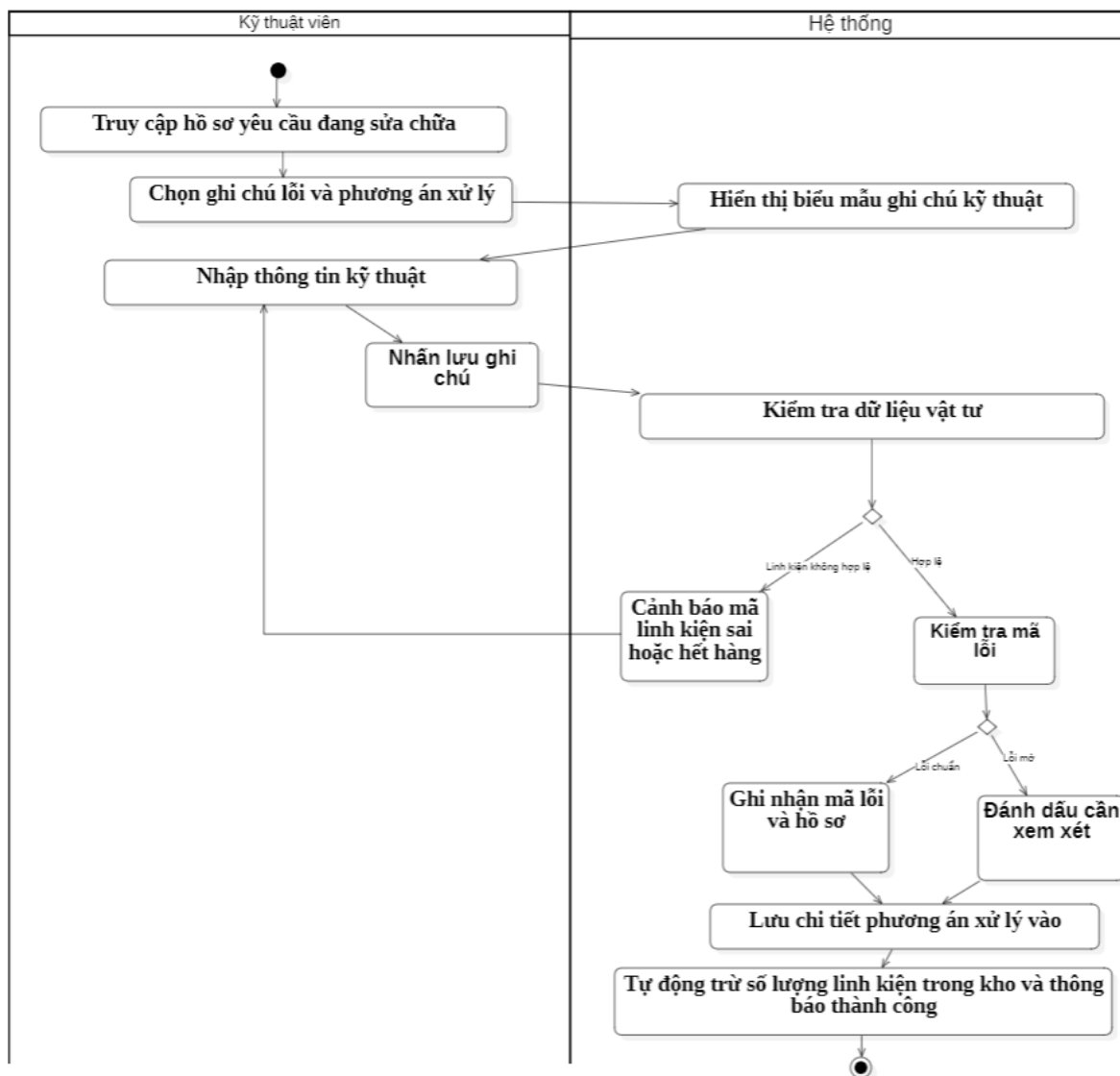
Biểu đồ hoạt động của Usecase “Ghi chú lỗi và phương án xử lý”
