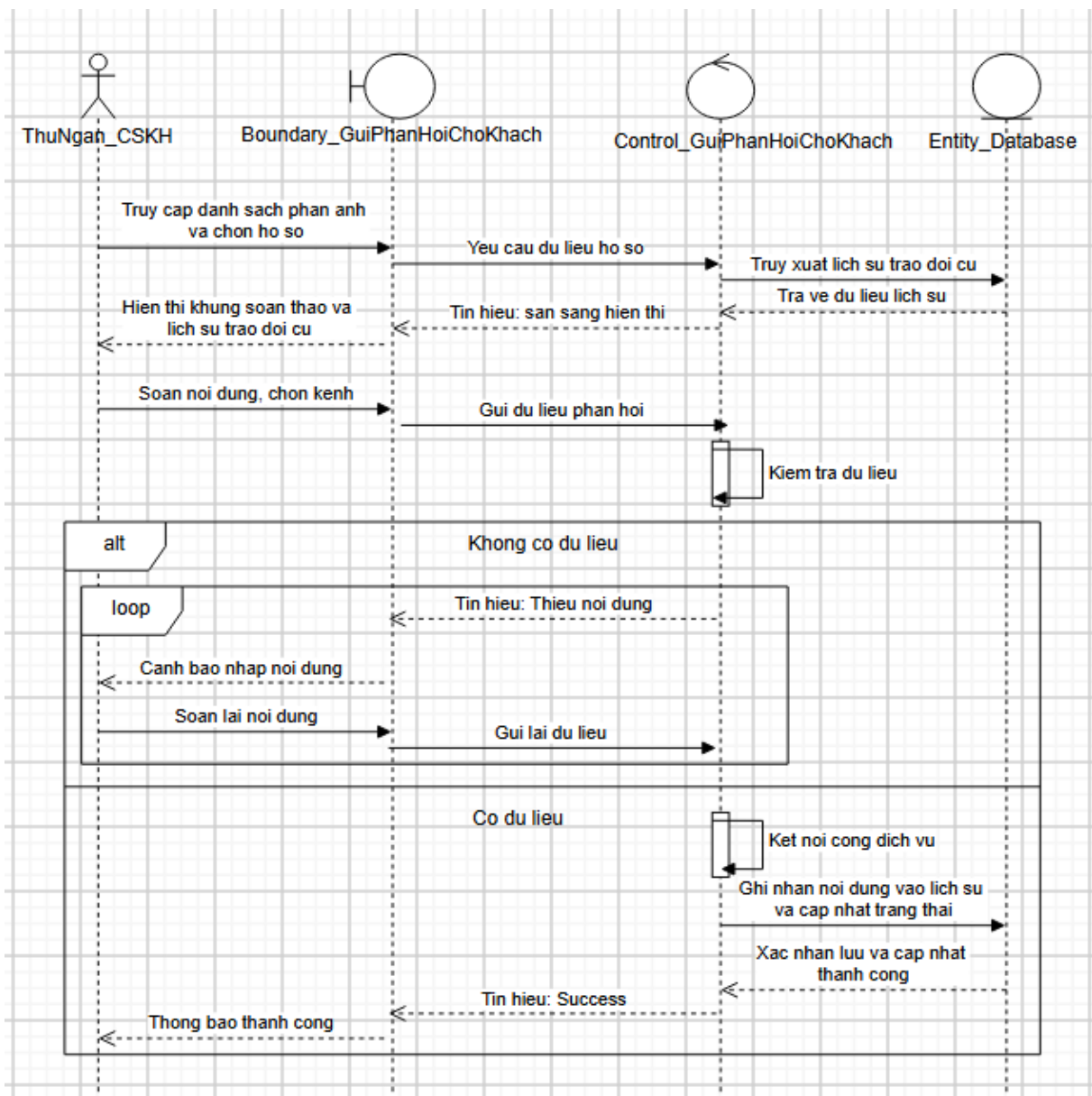
Biểu đồ tuần tự của Usecase “Gửi phản hồi cho khách”
