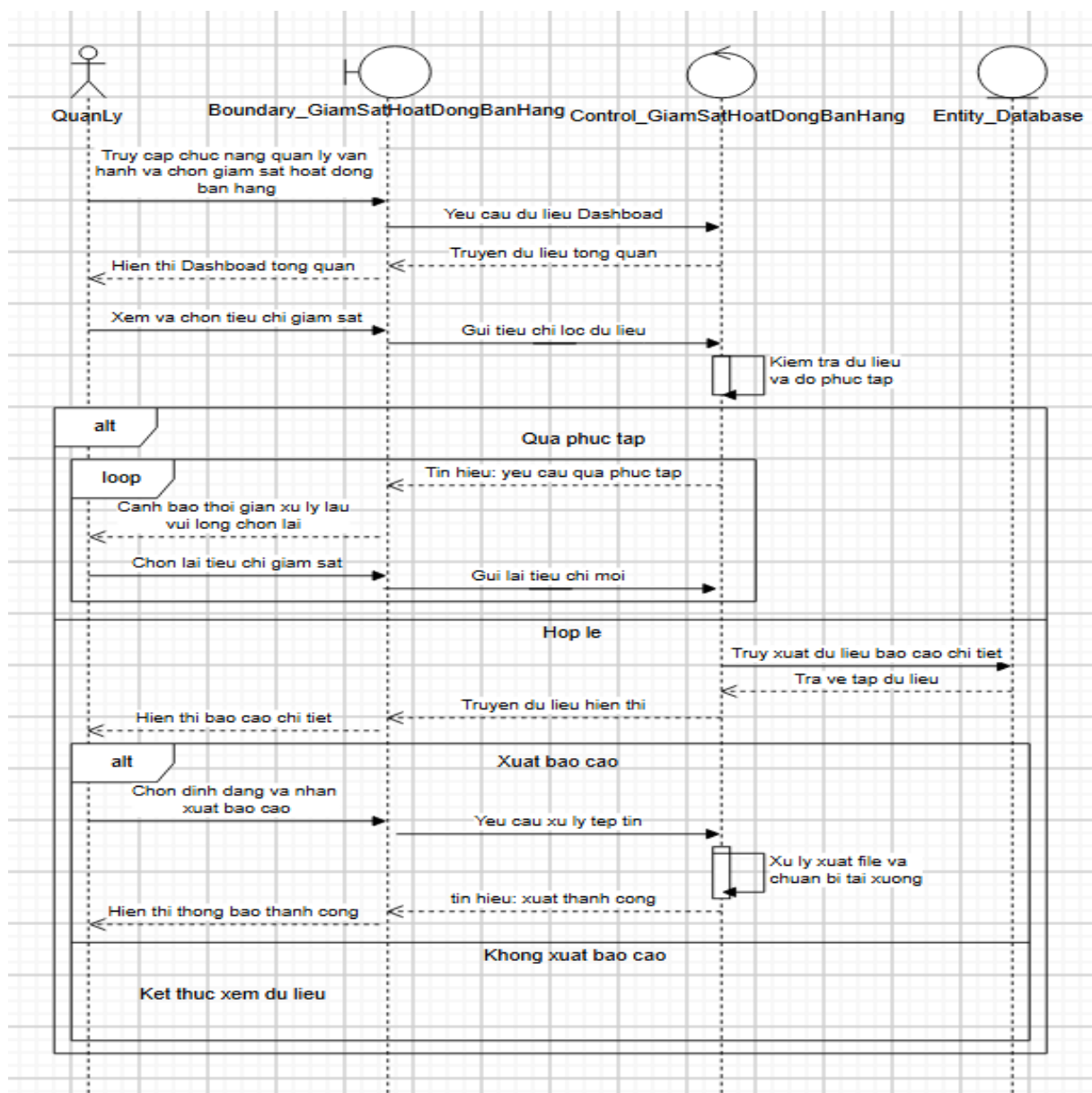
Biểu đồ tuần tự của Usecase “Giám sát hoạt động bán hàng”
