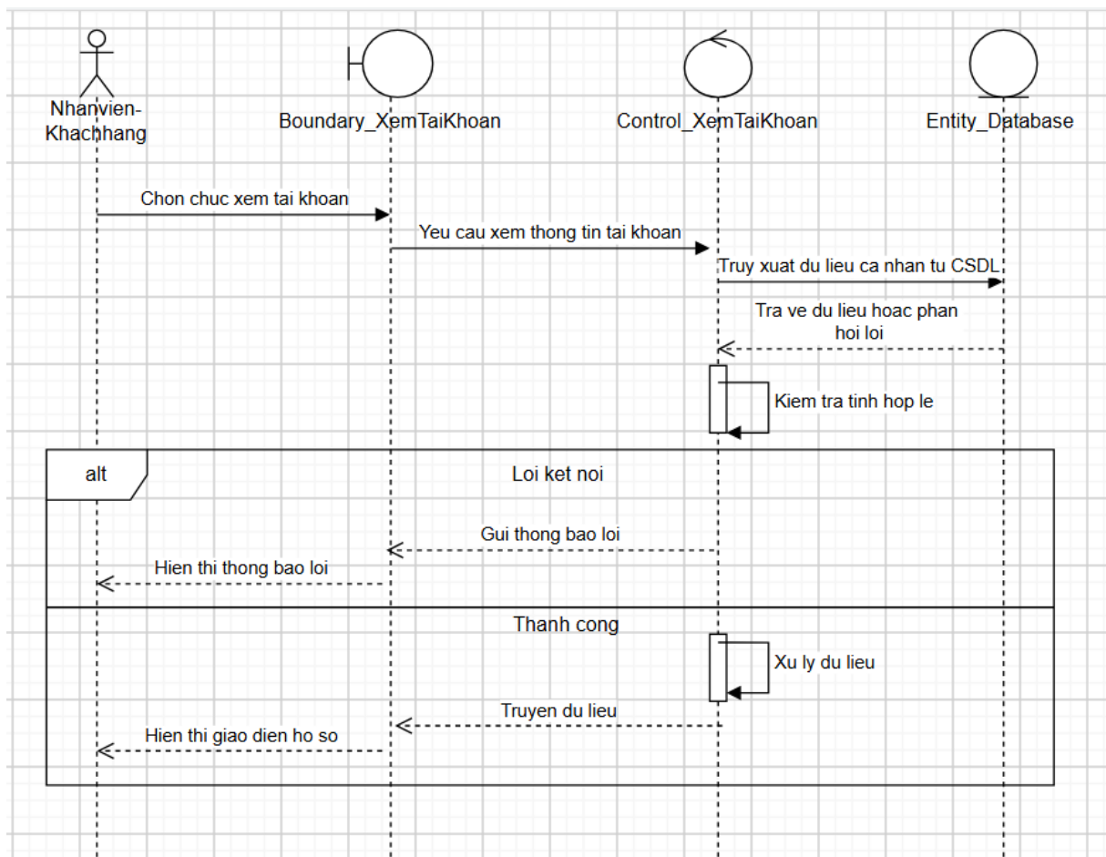
Biểu đồ tuần tự của Usecase “Xem tài khoản
