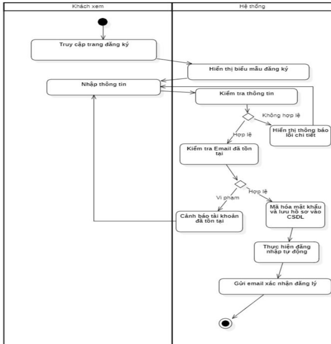
Biểu đồ hoạt động của Usecase “Đăng ký”
