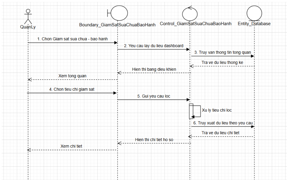
Biểu đồ tuần tự của Usecase “Giám sát sửa chữa - bảo hành”
