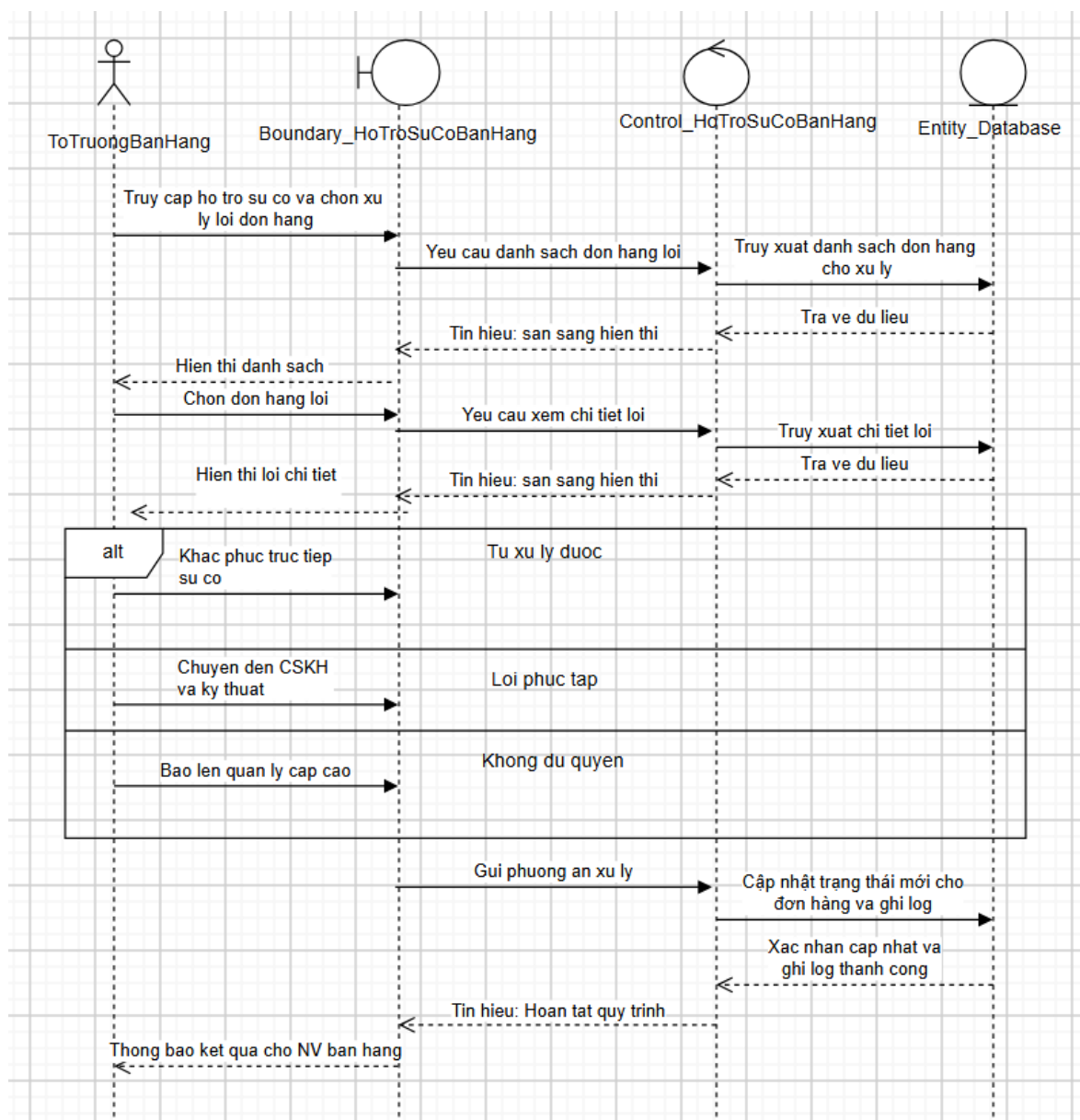
Biểu đồ tuần tự của Usecase “Xử lý lỗi đơn hàng”
