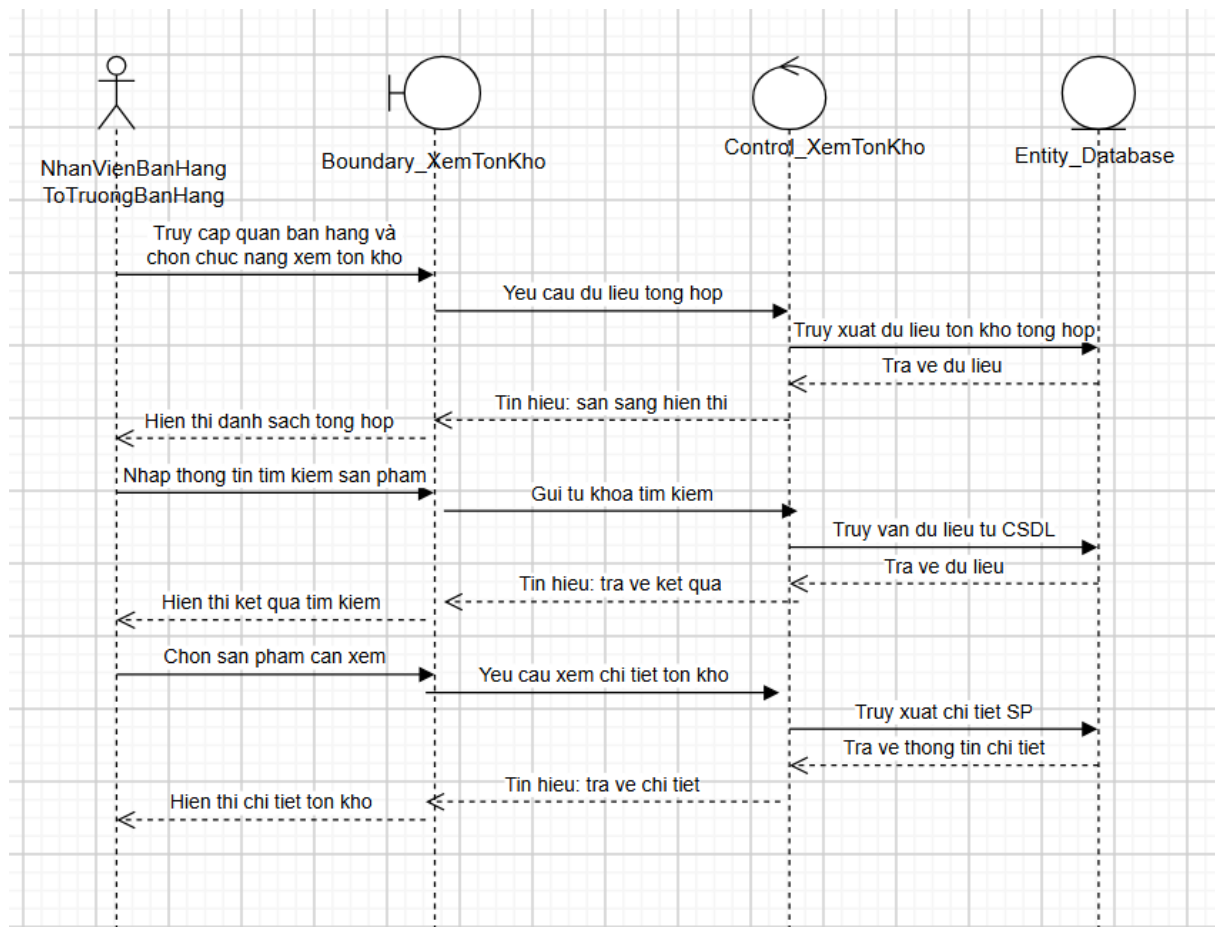
Biểu đồ tuần tự của Usecase “Xem tồn kho”
