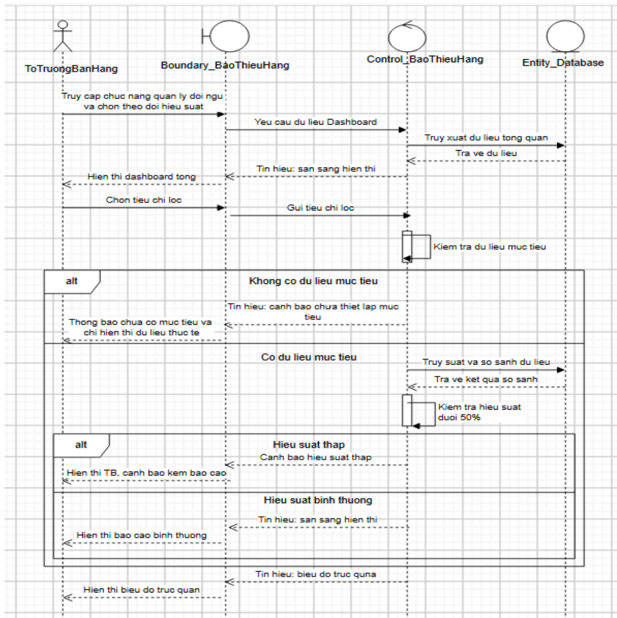
Biểu đồ tuần tự của Usecase “Theo dõi hiệu suất bán hàng”
