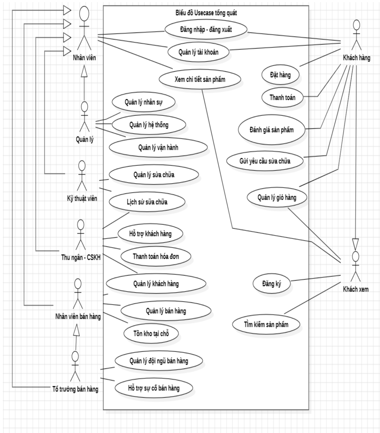
Hình 3: Biểu đồ Usecase tổng quát
