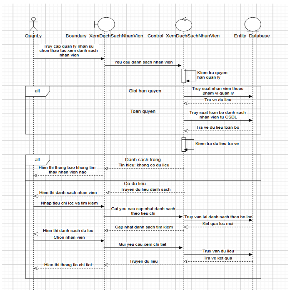
Biểu đồ tuần tự của Usecase “Xem danh sách nhân viên”
