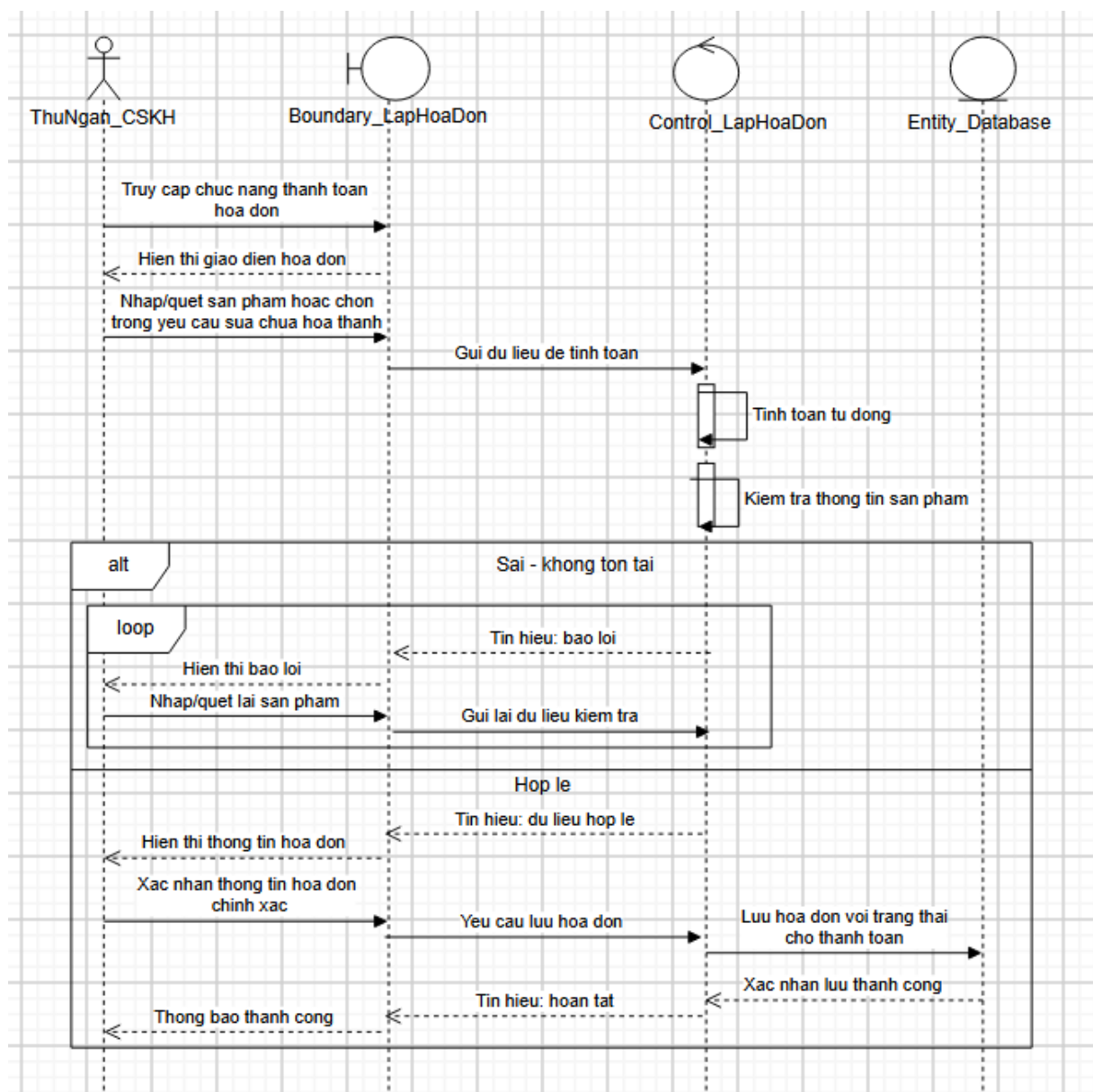
Biểu đồ tuần tự của Usecase “Lập hóa đơn”
