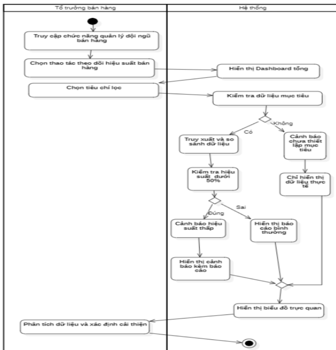
Biểu đồ hoạt động của Usecase “Theo dõi hiệu suất bán hàng”
