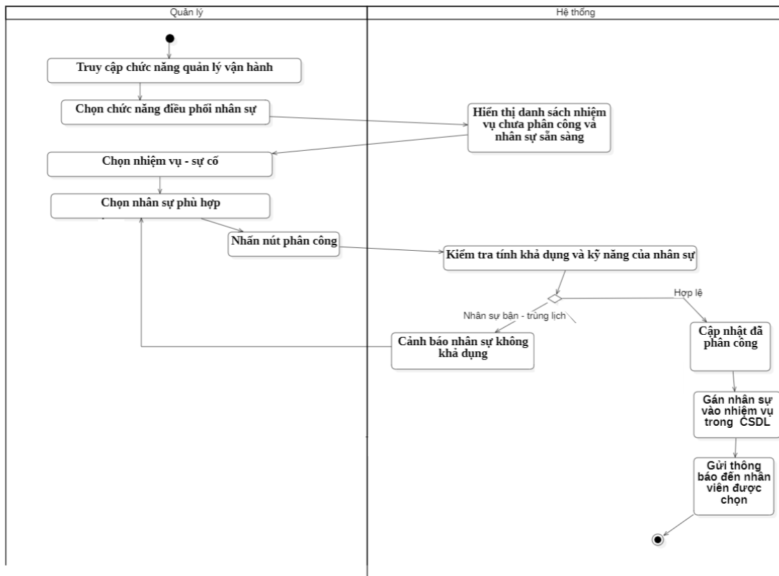
Biểu đồ hoạt động của Usecase “Điều phối nhân sự”
