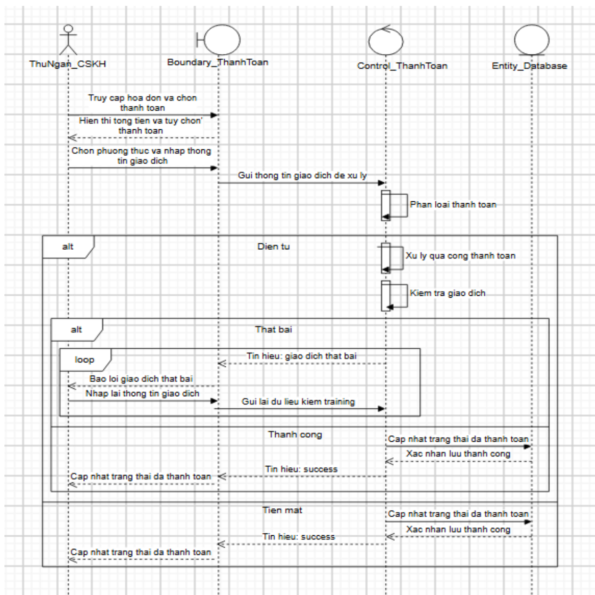
Biểu đồ tuần tự của Usecase “Thanh toán”
