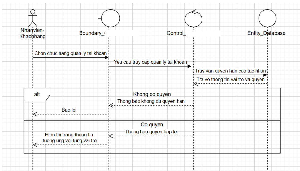
Biểu đồ tuần tự của Usecase “Quản lý tài khoản”
