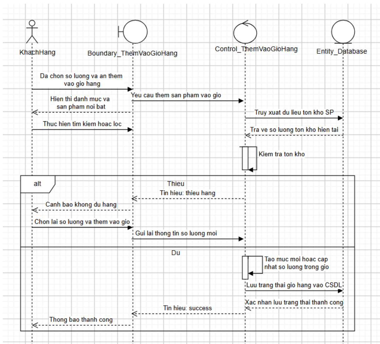
Biểu đồ tuần tự của Usecase “Thêm vào giỏ hàng”
