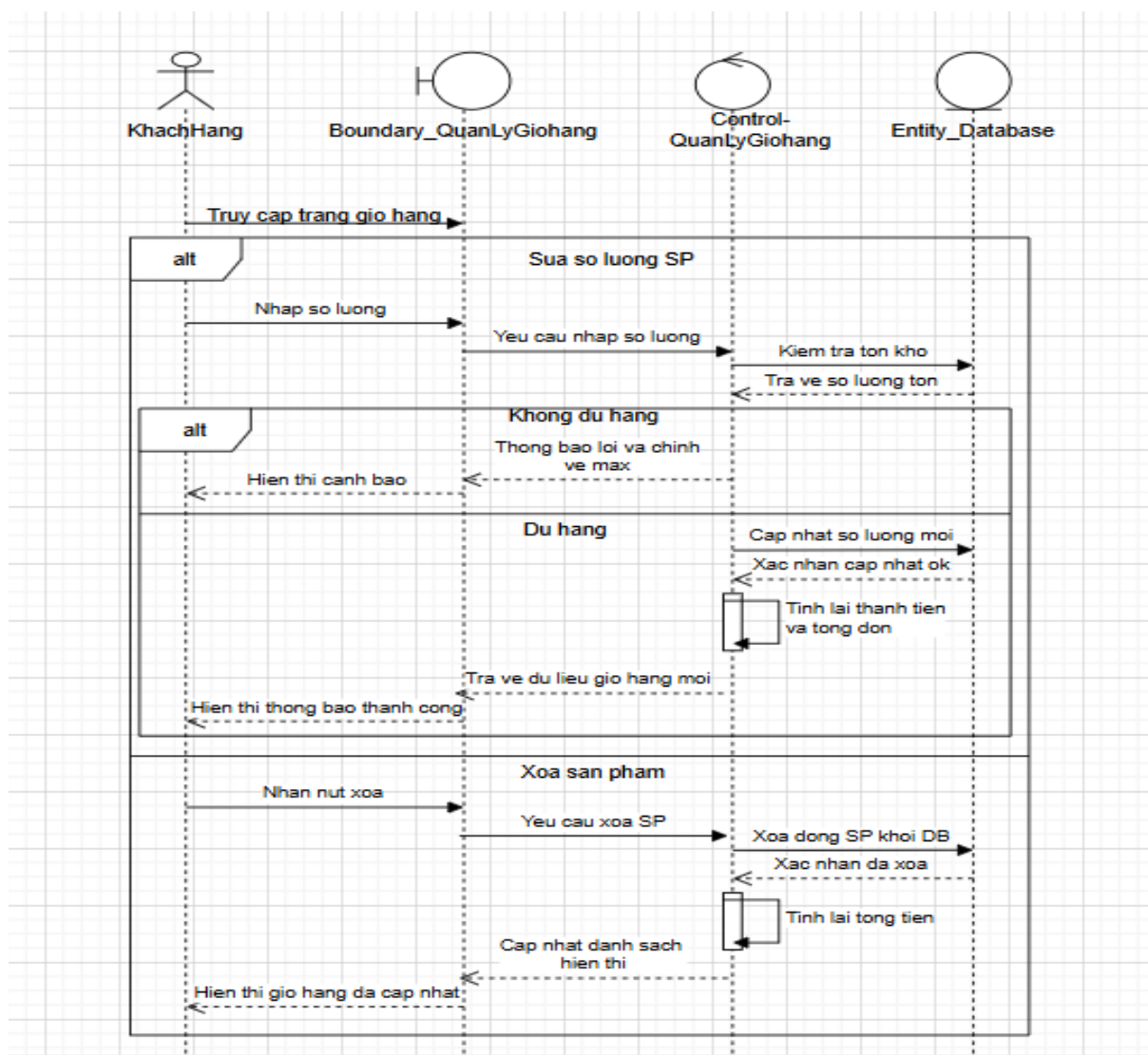
Biểu đồ tuần tự của Usecase “Quản lý giỏ hàng”
