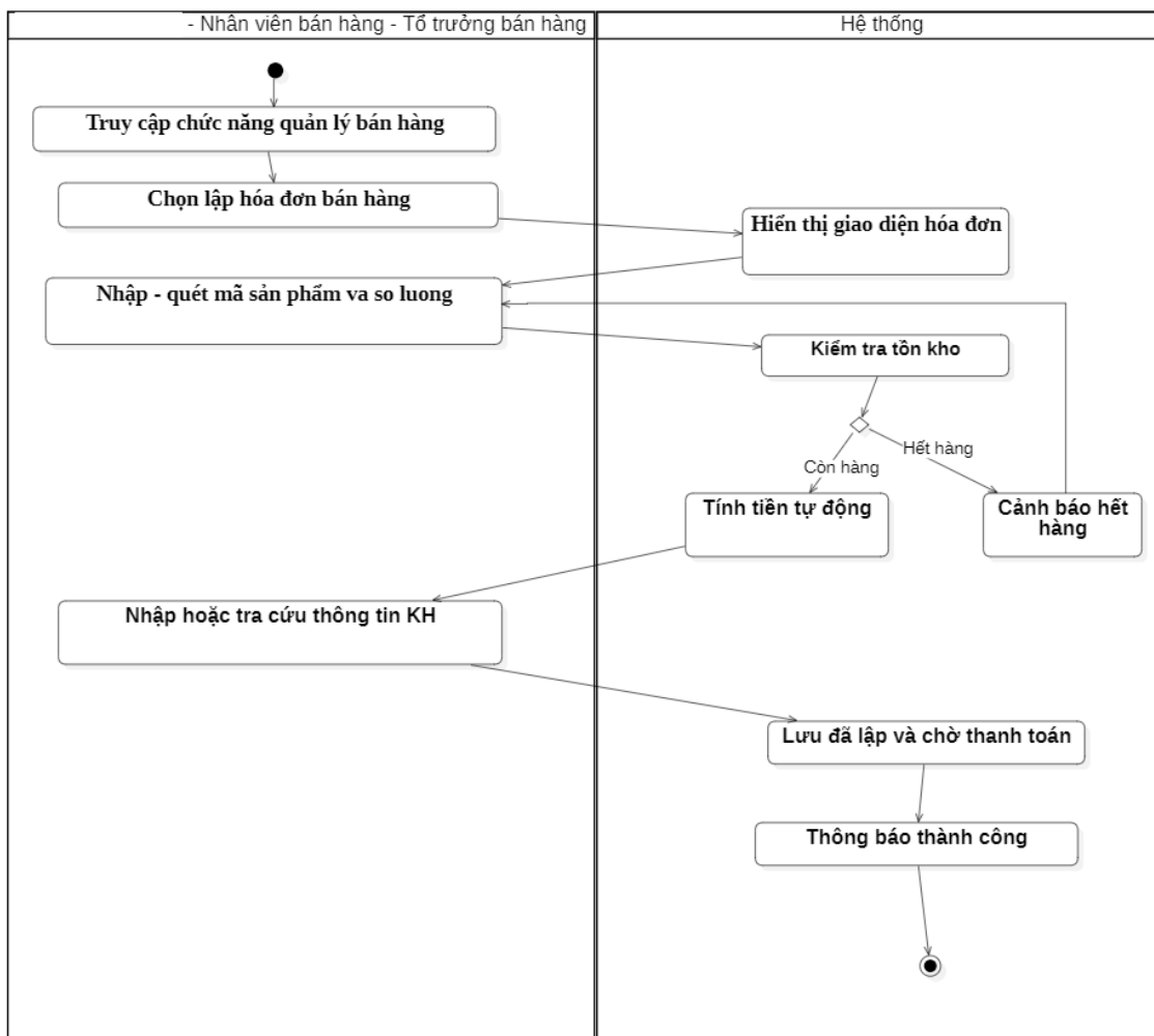
Biểu đồ hoạt động của Usecase “Lập hóa đơn bán hàng”
