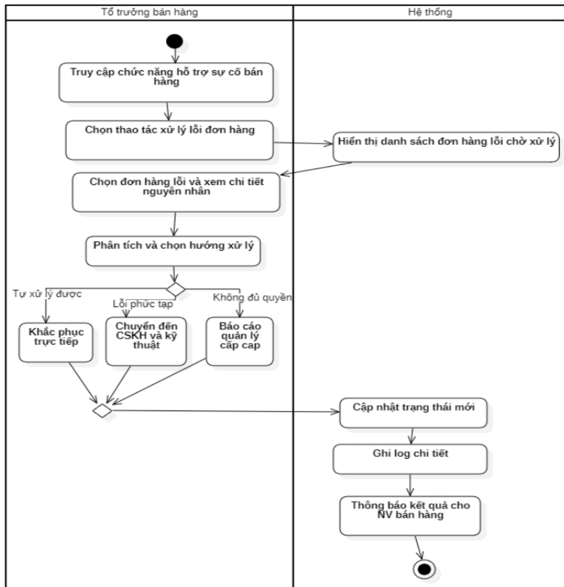
Biểu đồ hoạt động của Usecase “Xử lý lỗi đơn hàng”
