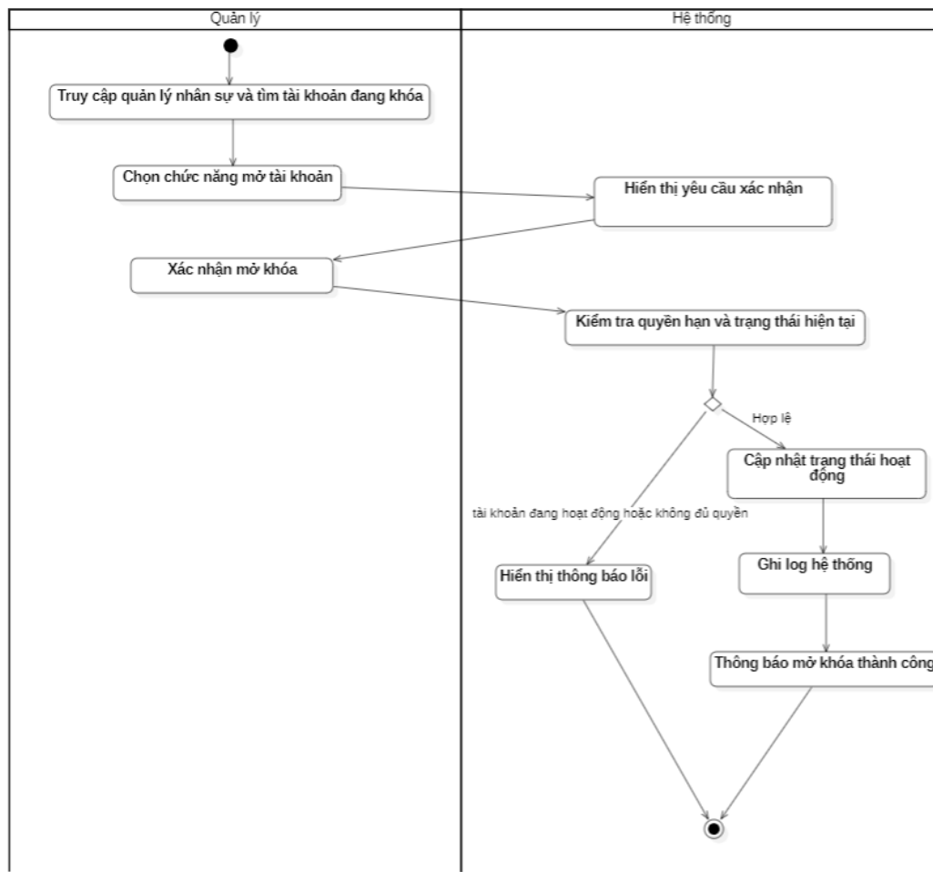
Biểu đồ hoạt động của Usecase “Mở tài khoản”
