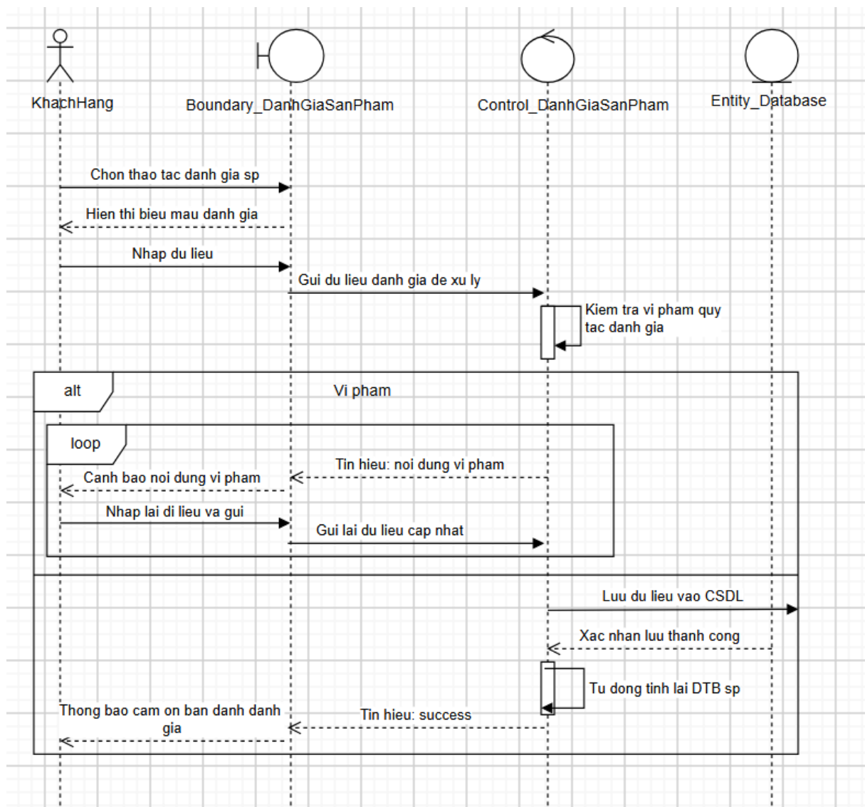
Biểu đồ tuần tự của Usecase “Đánh giá sản phẩm”
