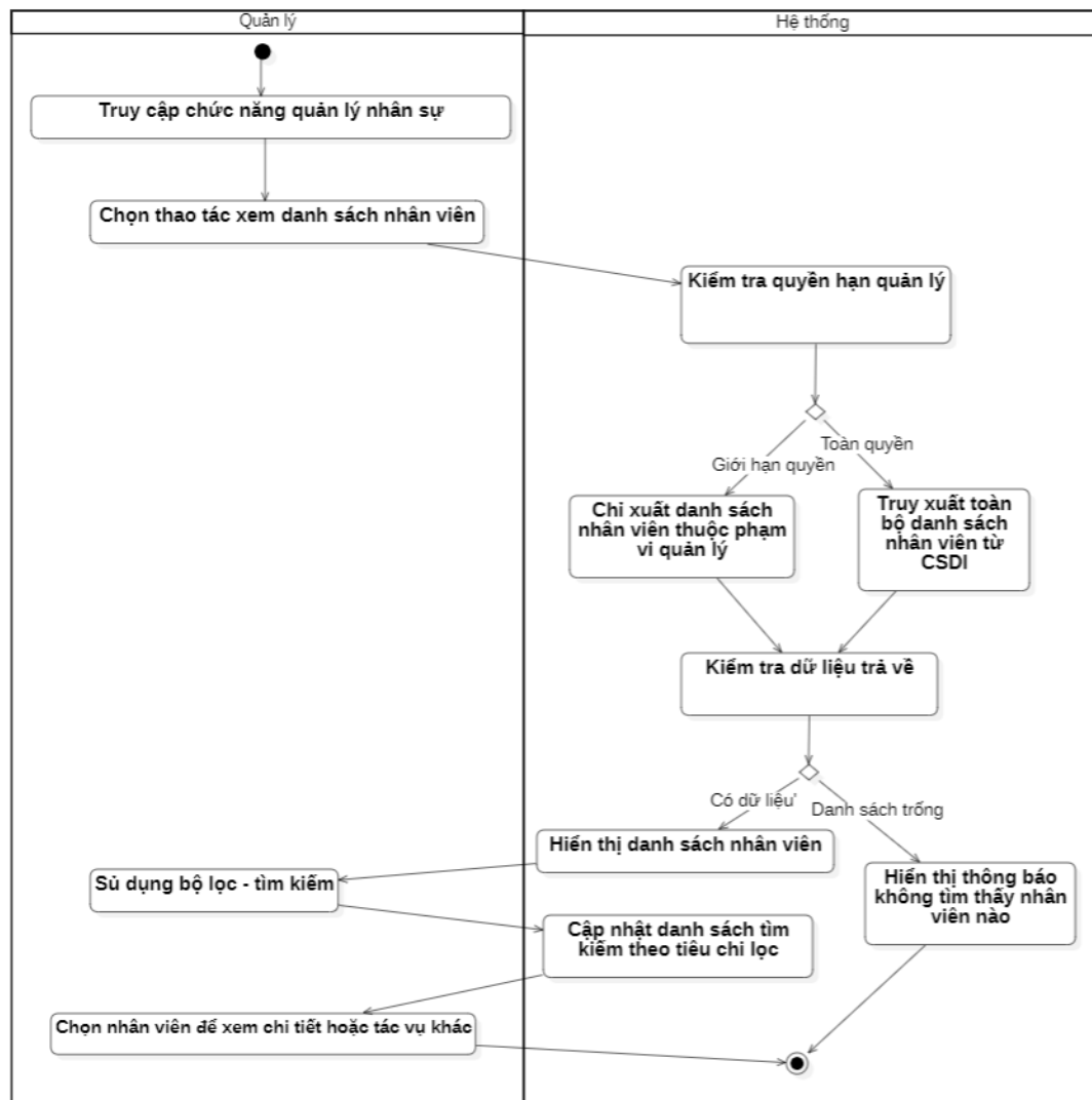
Biểu đồ hoạt động của Usecase “Xem danh sách nhân viên”
