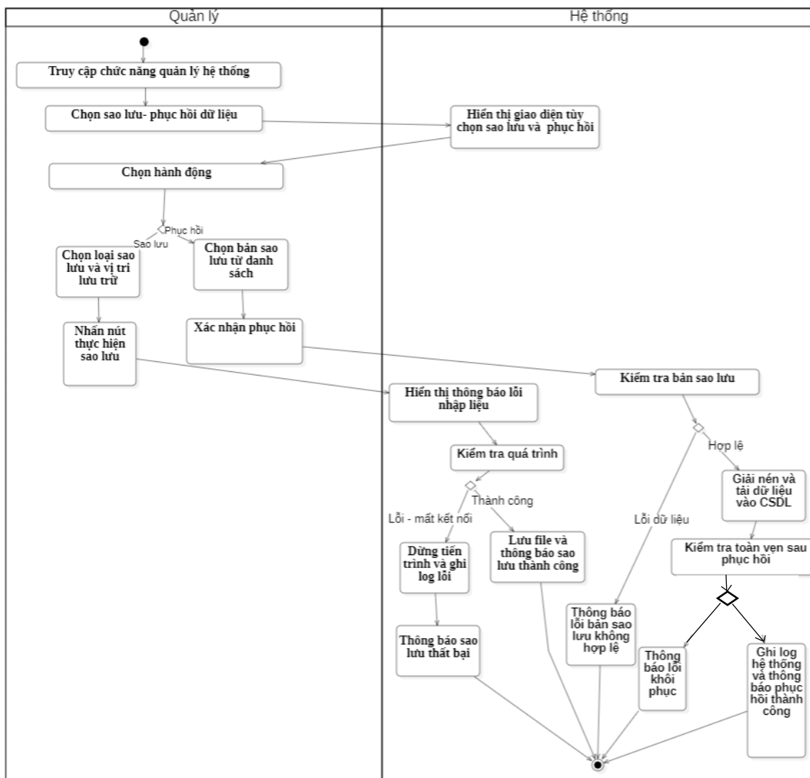
Biểu đồ hoạt động của Usecase “Sao lưu - phục hồi dữ liệu”
