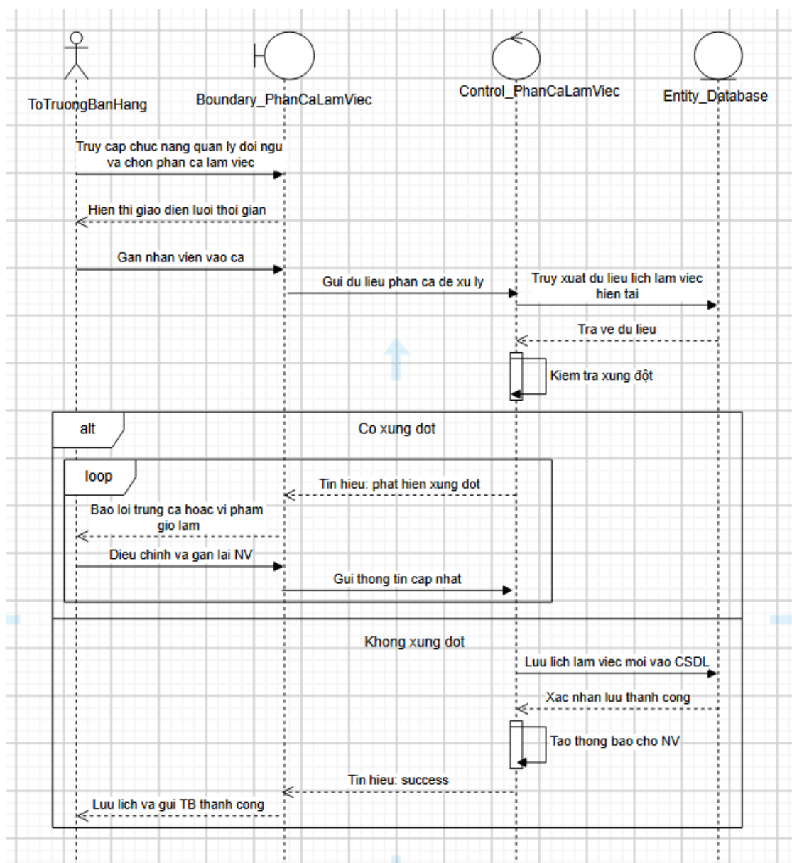
Biểu đồ tuần tự của Usecase “Phân ca làm việc”
