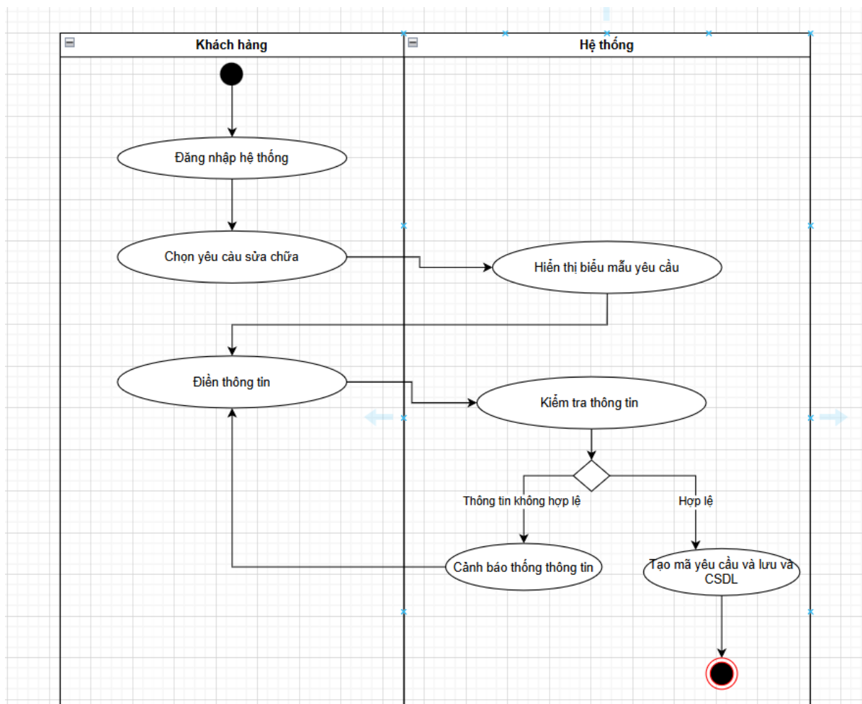
Biểu đồ hoạt động của Usecase “Gửi yêu cầu sửa chữa”
