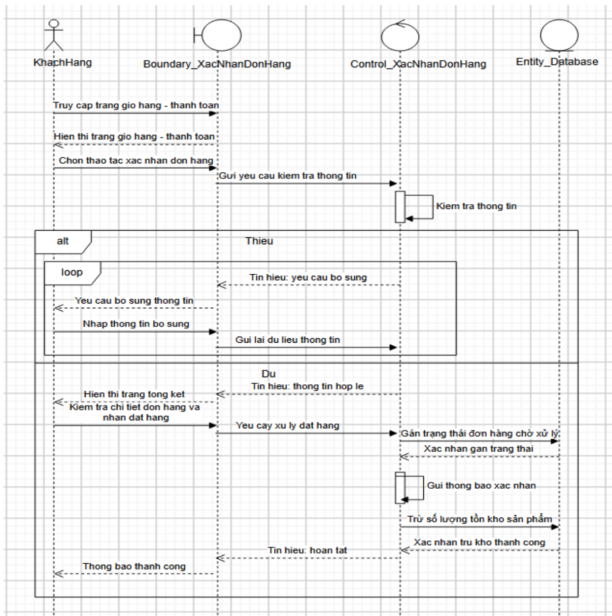
Biểu đồ tuần tự của Usecase “Xác nhận đơn hàng”
