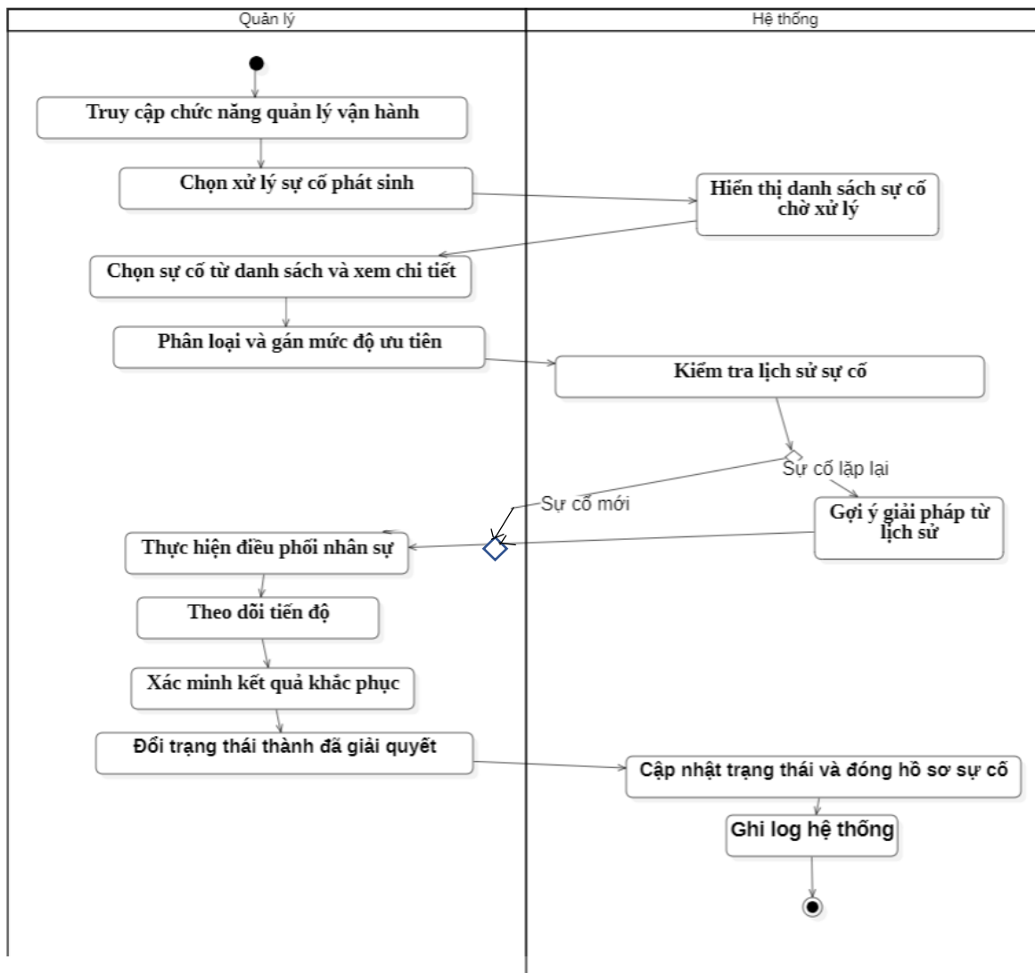
Biểu đồ hoạt động của Usecase “Xử lý sự cố phát sinh”
