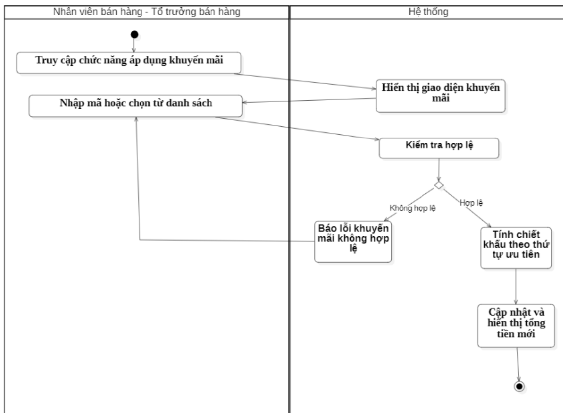
Biểu đồ hoạt động của Usecase “Áp dụng khuyến mãi”
