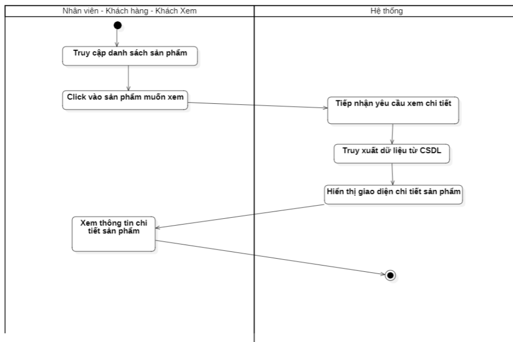
Biểu đồ hoạt động của Usecase “Xem chi tiết sản phẩm”
