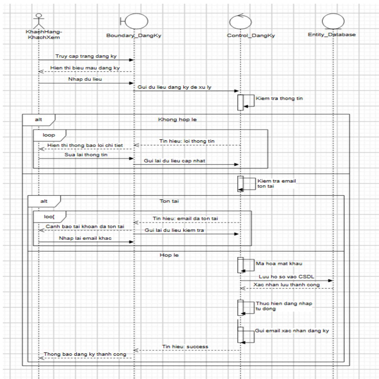
Biểu đồ tuần tự của Usecase “Đăng ký”
