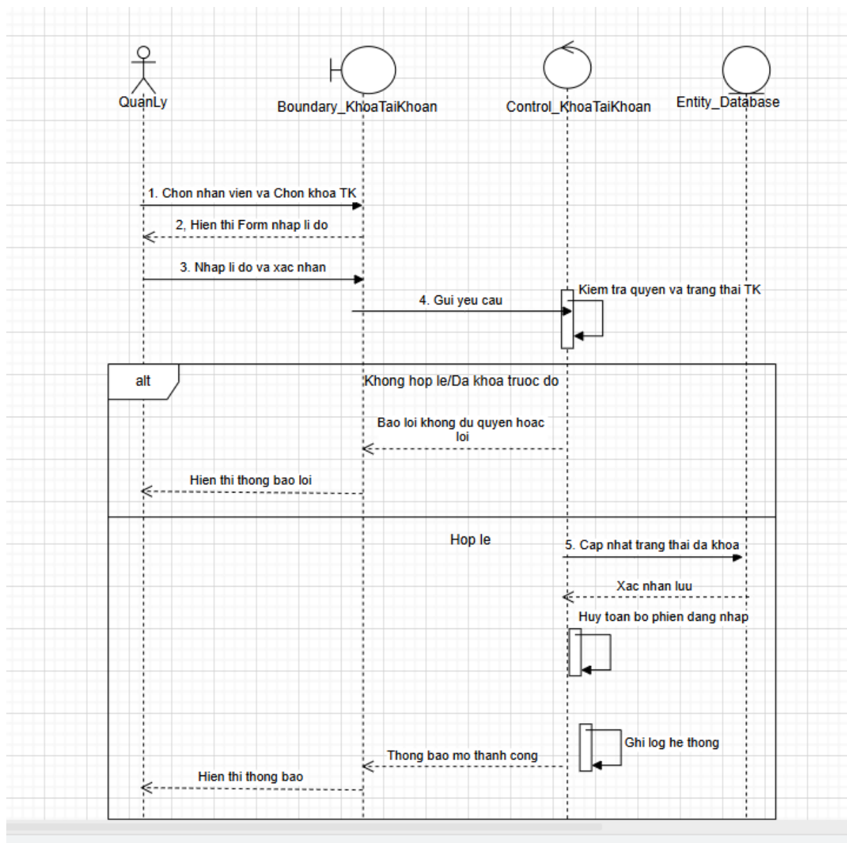
Biểu đồ tuần tự của Usecase “Khóa tài khoản”
