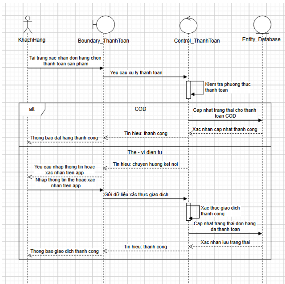
Biểu đồ tuần tự của Usecase “Thanh toán sản phẩm”
