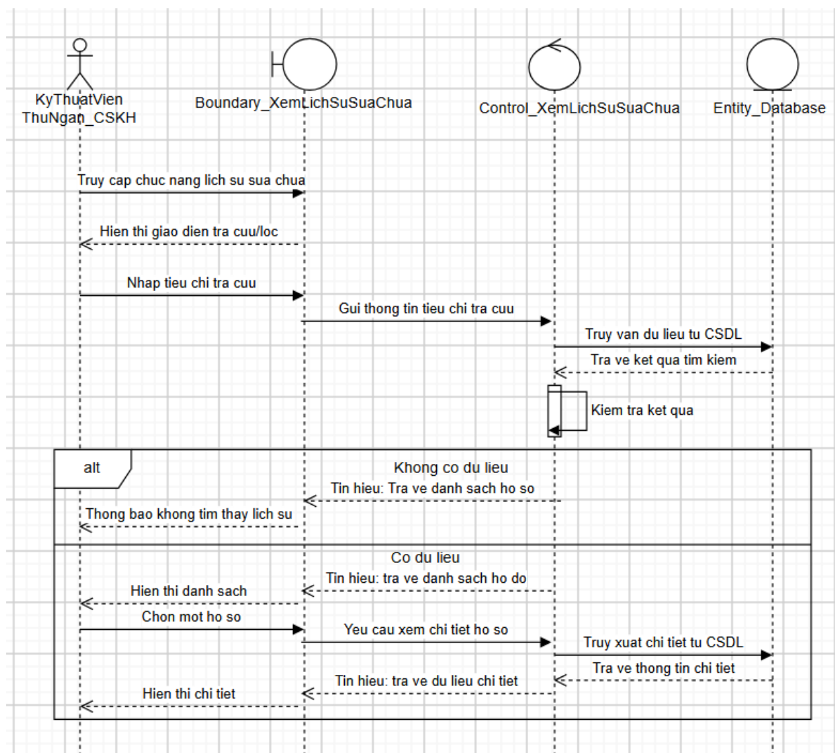
Biểu đồ tuần tự của Usecase “Xem lịch sử sửa chữa”
