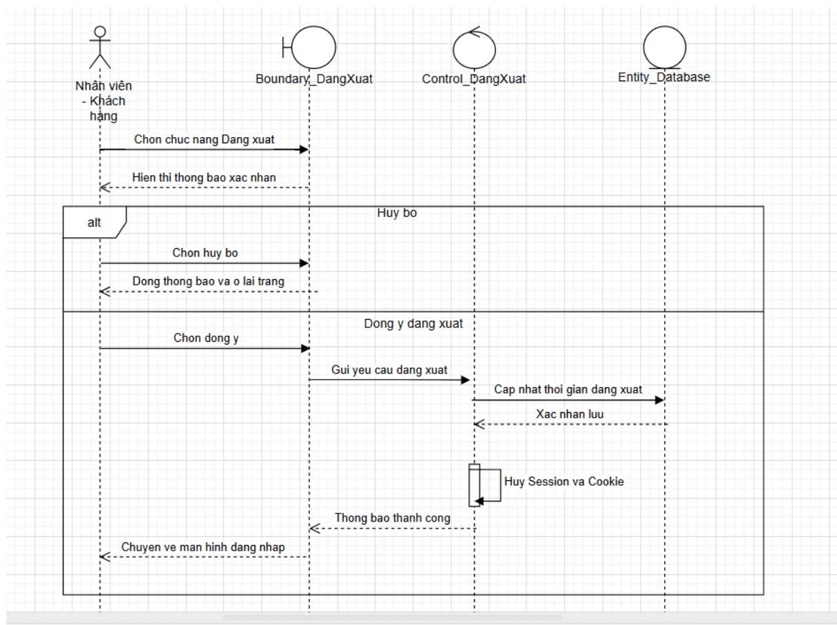
Biểu đồ tuần tự của Usecase “Đăng xuất”
