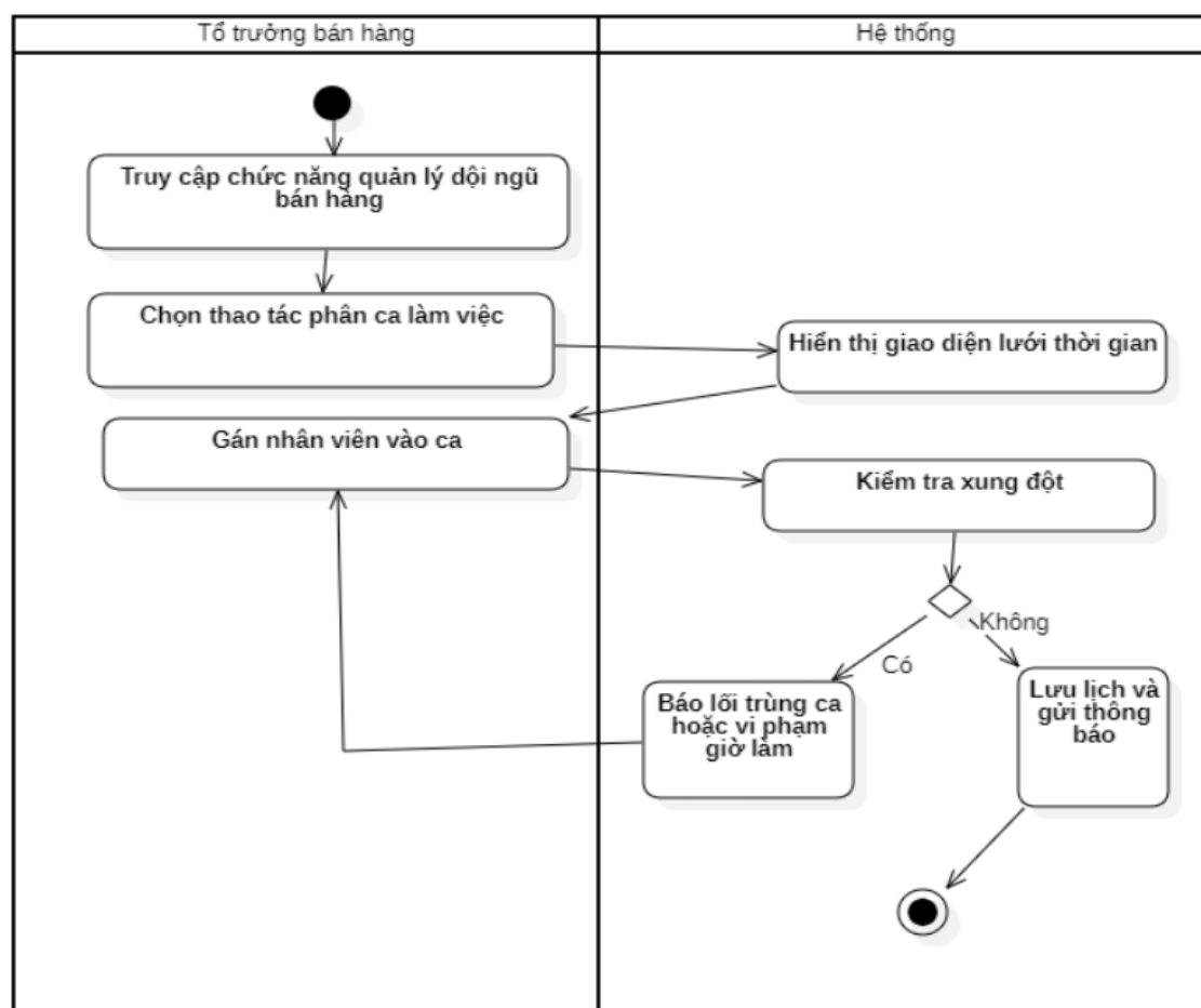
Biểu đồ hoạt động của Usecase “Phân ca làm việc”
