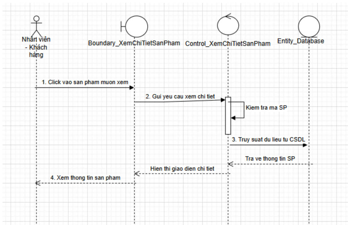
Biểu đồ tuần tự của Usecase “Xem chi tiết sản phẩm”
