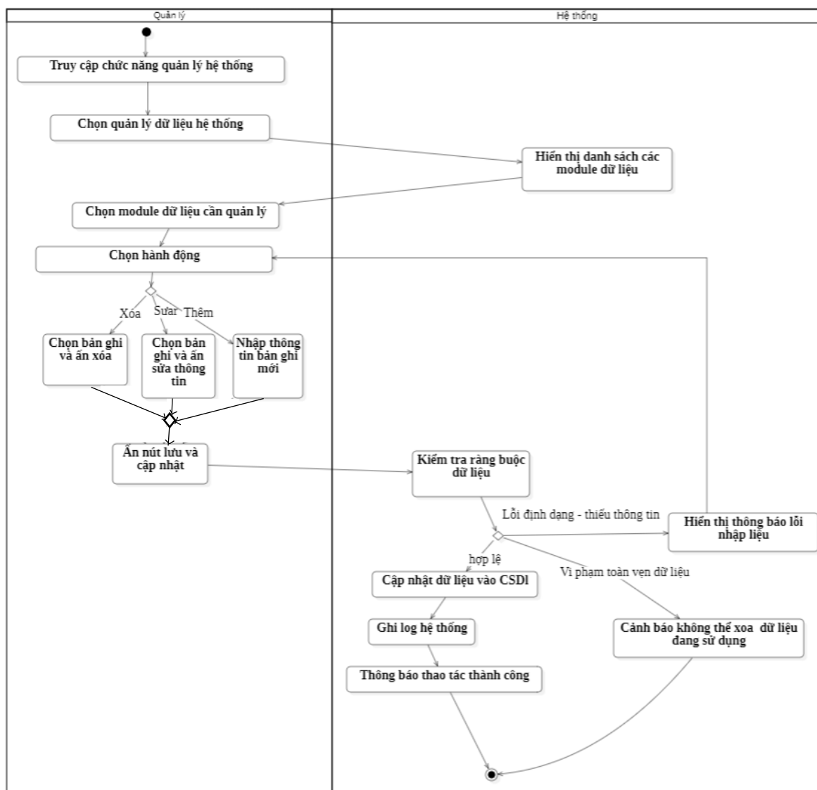
Biểu đồ hoạt động của Usecase “Quản lý dữ liệu hệ thống”
