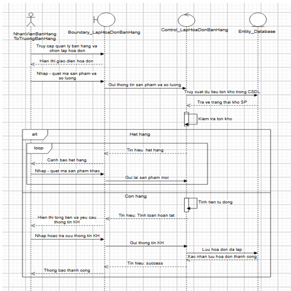
Biểu đồ tuần tự của Usecase “Lập hóa đơn bán hàng”
