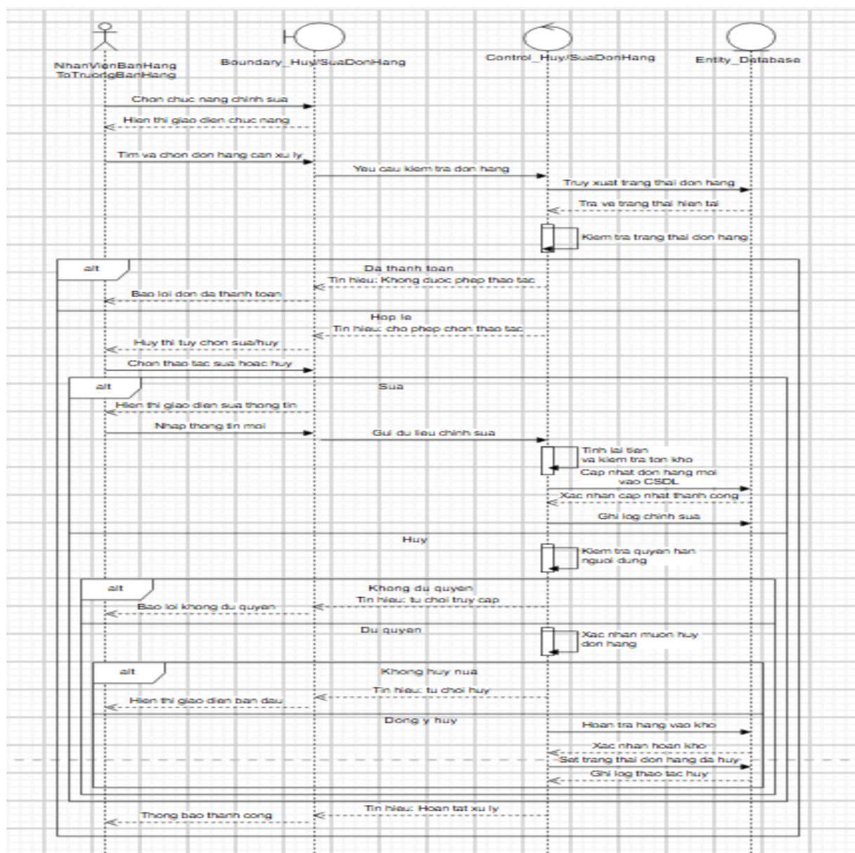
Biểu đồ tuần tự của Usecase “Hủy/chỉnh sửa đơn hàng”
