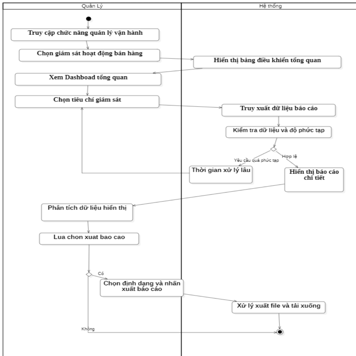
Biểu đồ hoạt động của Usecase “Giám sát hoạt động bán hàng”
