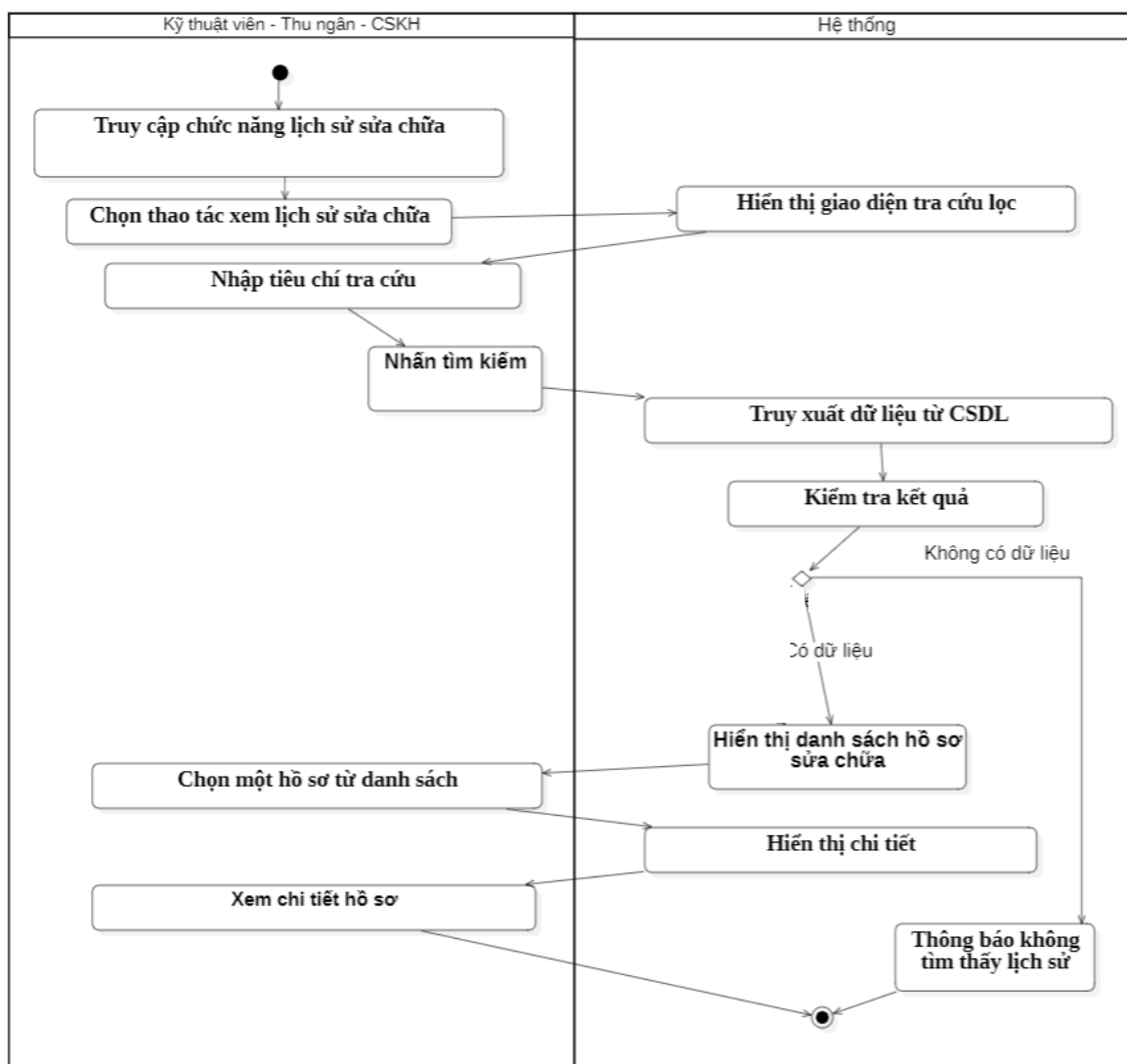
Biểu đồ hoạt động của Usecase “Xem lịch sử sửa chữa”
