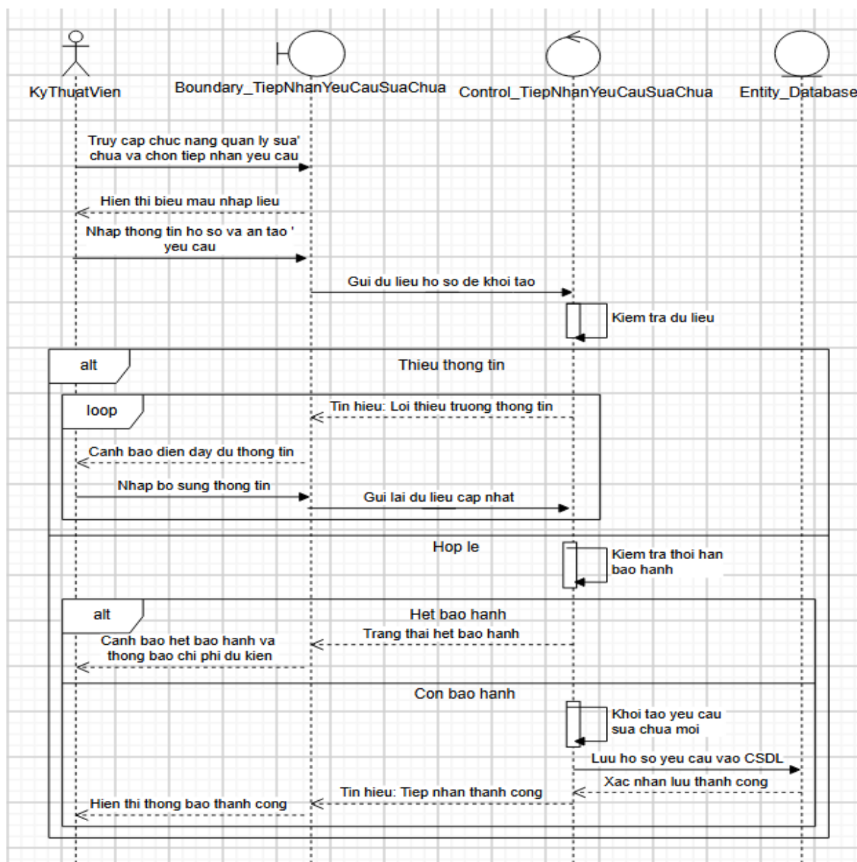
Biểu đồ tuần tự của Usecase “Tiếp nhận yêu cầu sửa chữa”
