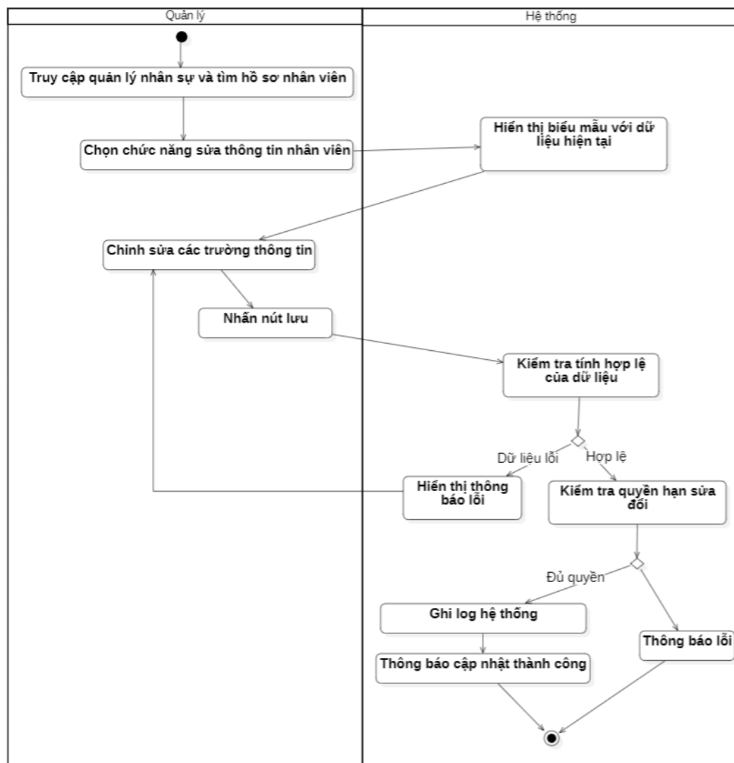
Biểu đồ hoạt động của Usecase “Sửa thông tin nhân viên”
