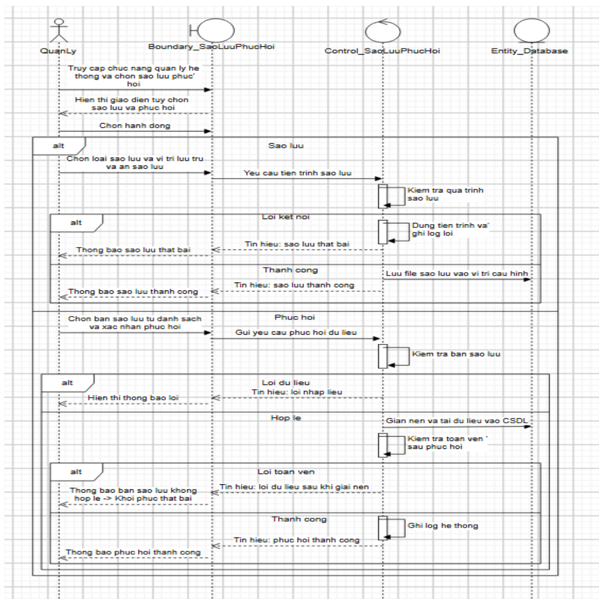
Biểu đồ tuần tự của Usecase “Sao lưu - phục hồi dữ liệu”
