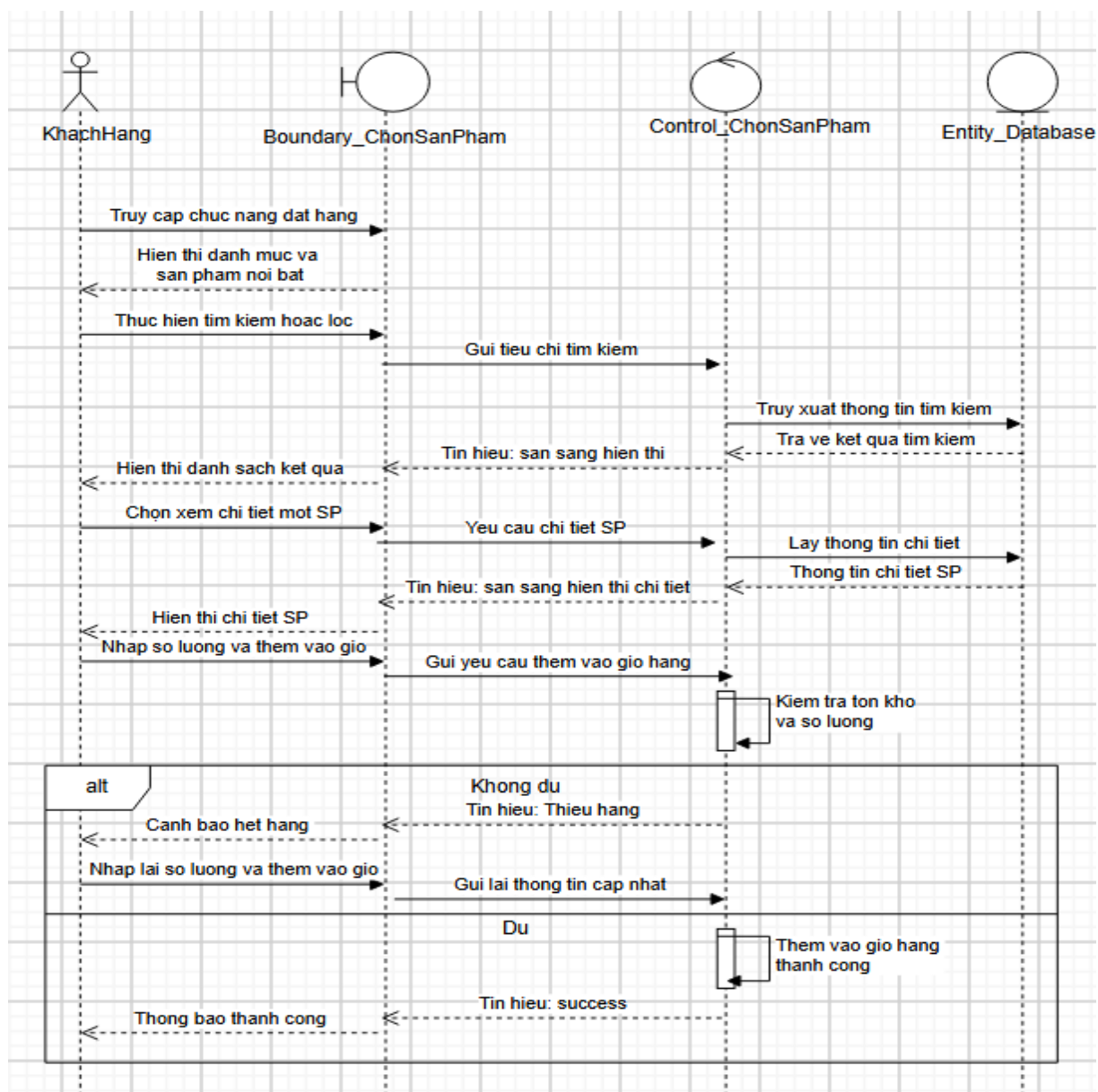
Biểu đồ tuần tự của Usecase “Chọn sản phẩm ”
