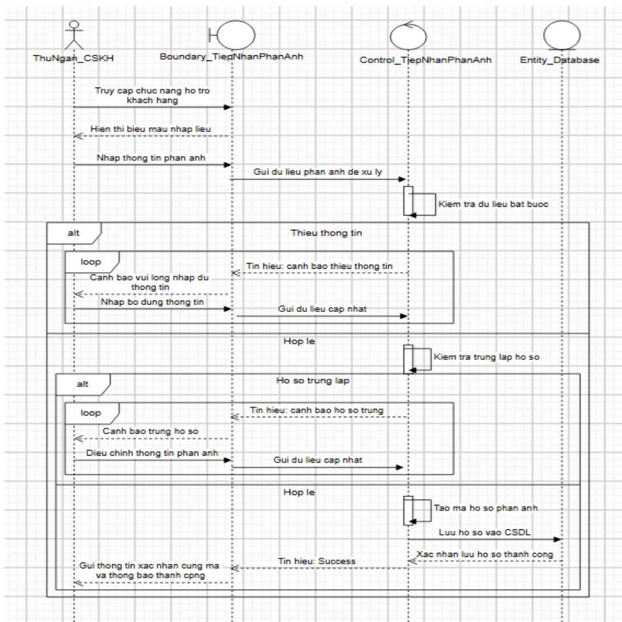
Biểu đồ tuần tự của Usecase “Tiếp nhận phản ánh”
