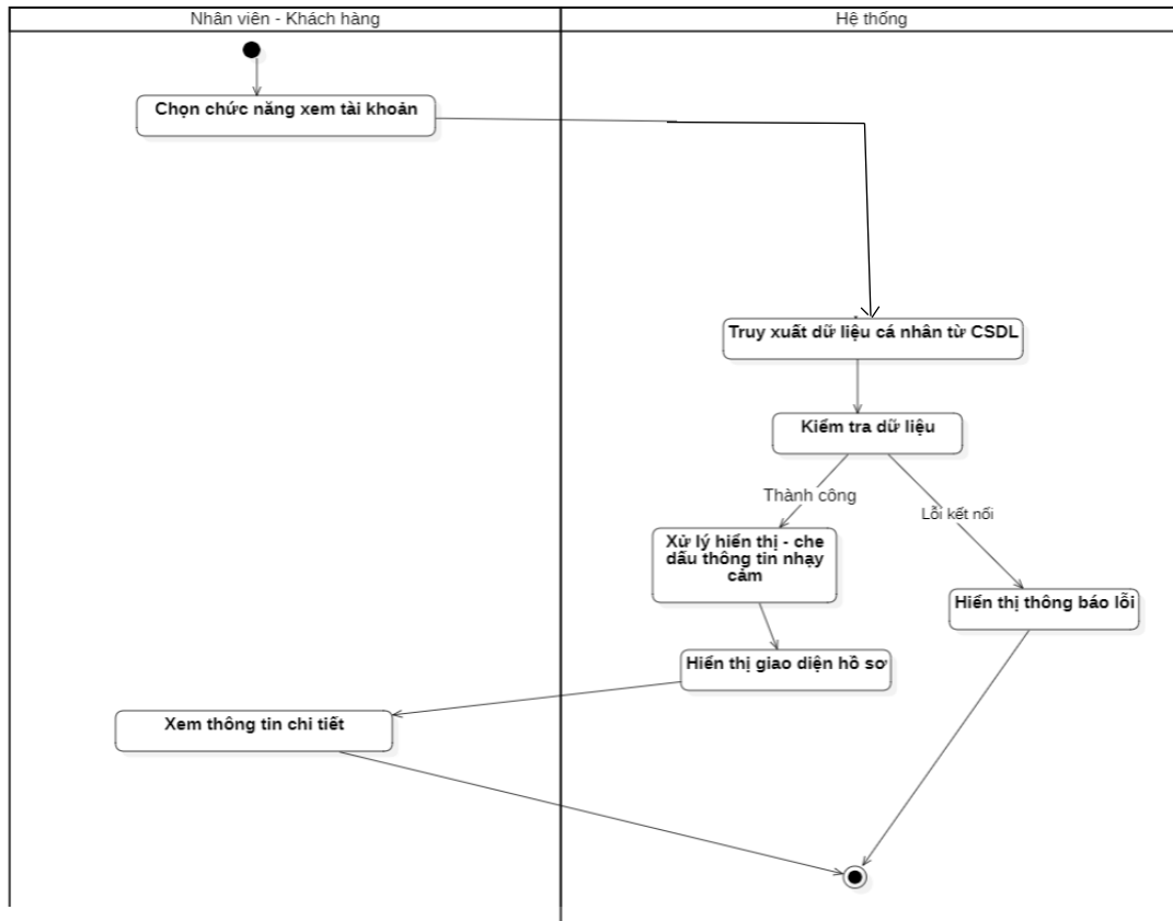
Biểu đồ hoạt động của Usecase “Xem tài khoản”
