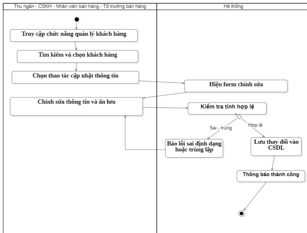
Biểu đồ hoạt động của Usecase “Cập nhật thông tin khách hàng”
