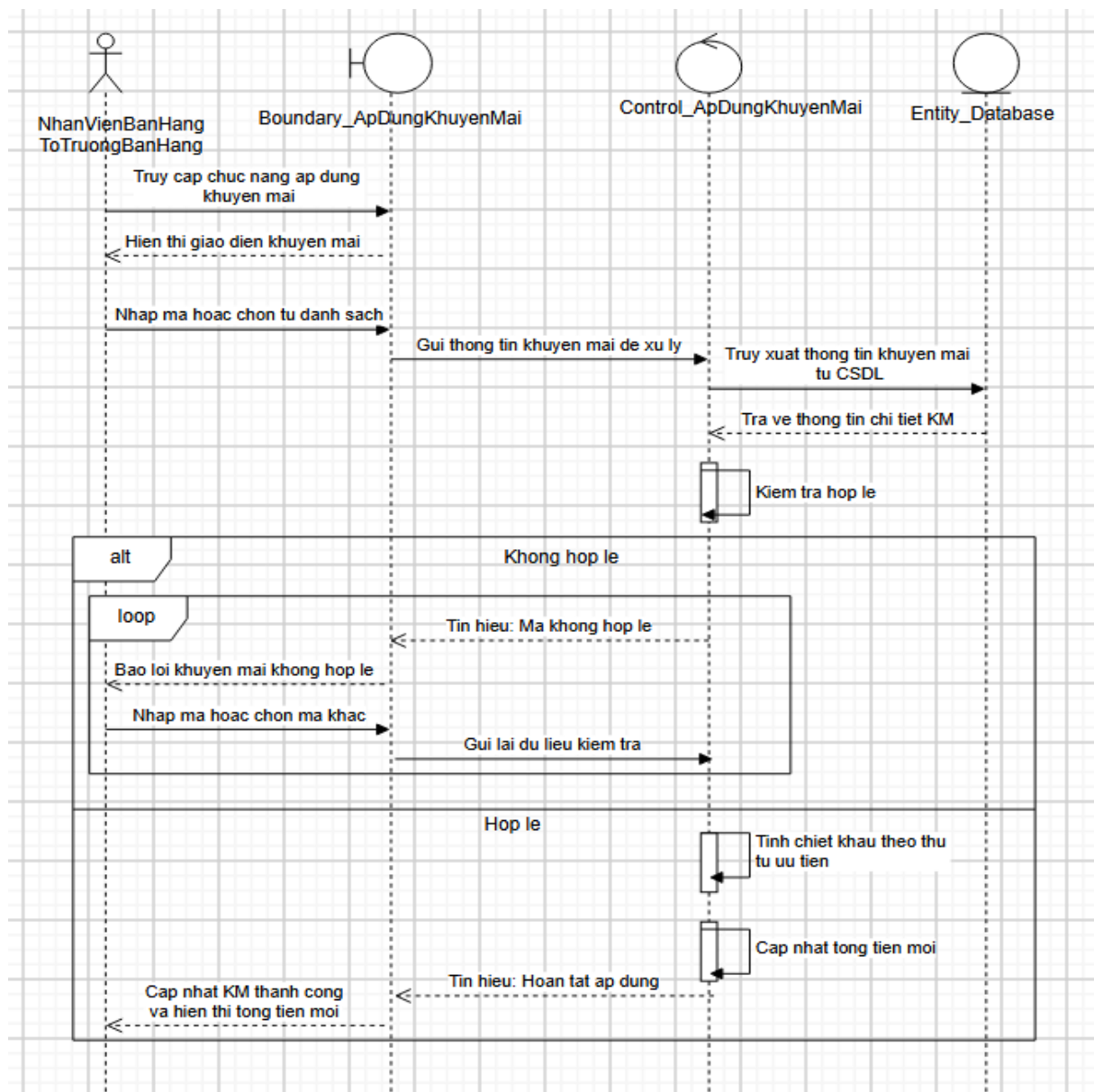
Biểu đồ tuần tự của Usecase “Áp dụng khuyến mãi”
