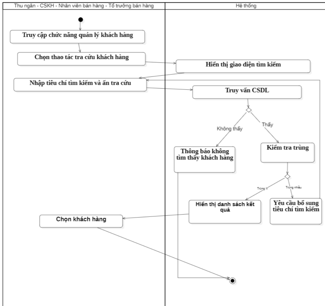
Biểu đồ hoạt động của Usecase “Tra cứu khách hàng”
