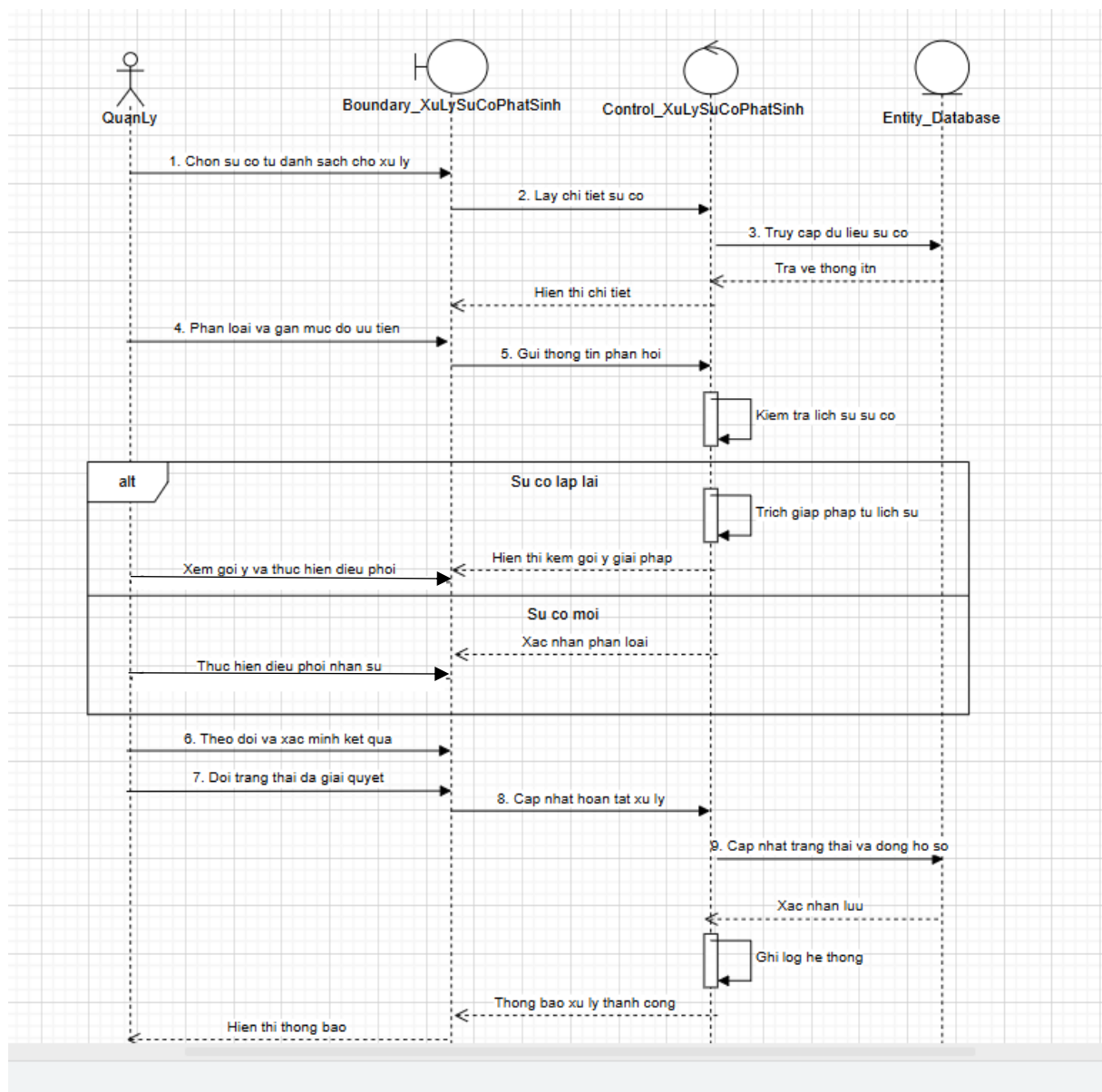
Biểu đồ tuần tự của Usecase “Xử lý sự cố phát sinh”
