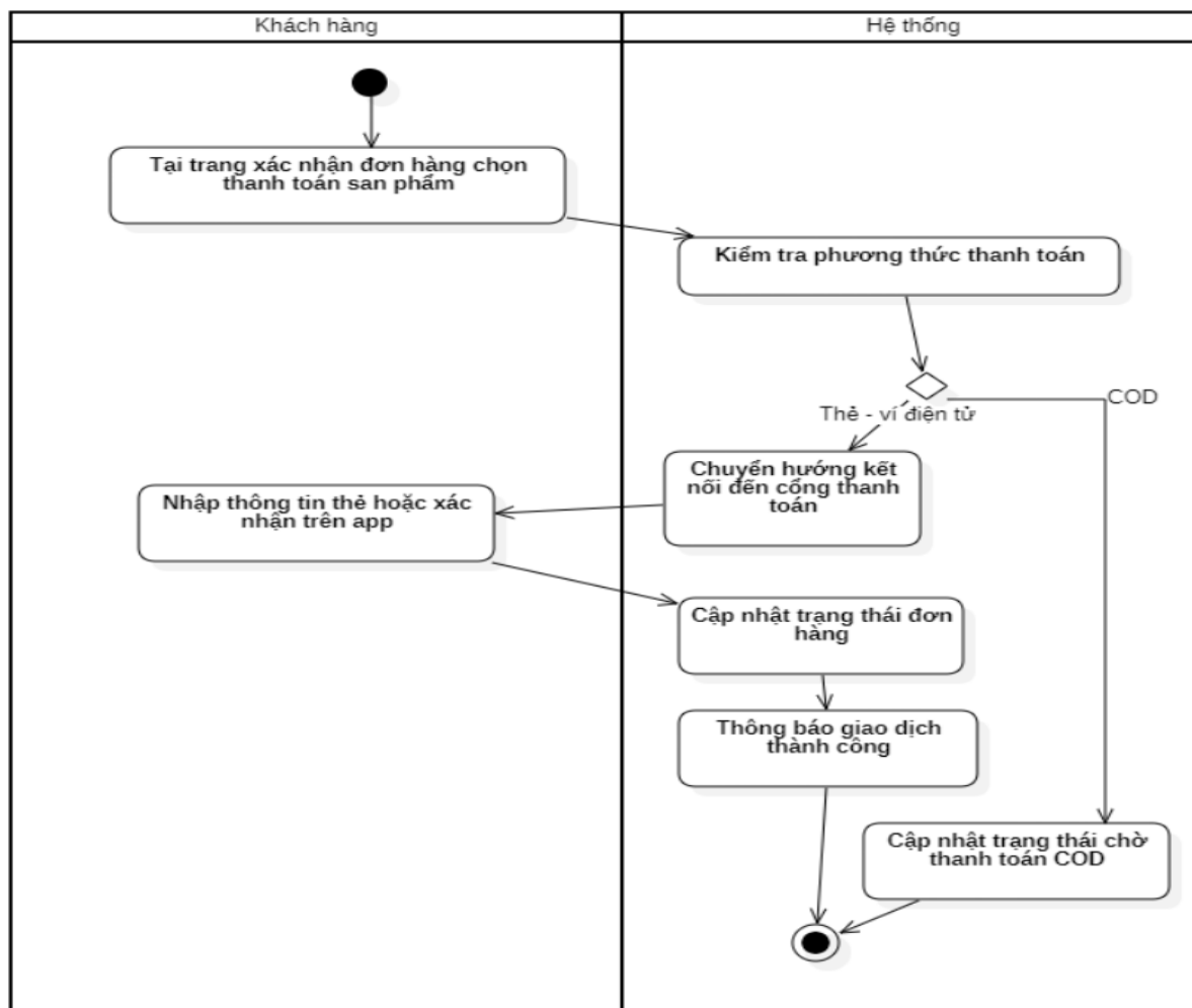
Usecase “Thanh toán sản phẩm”
