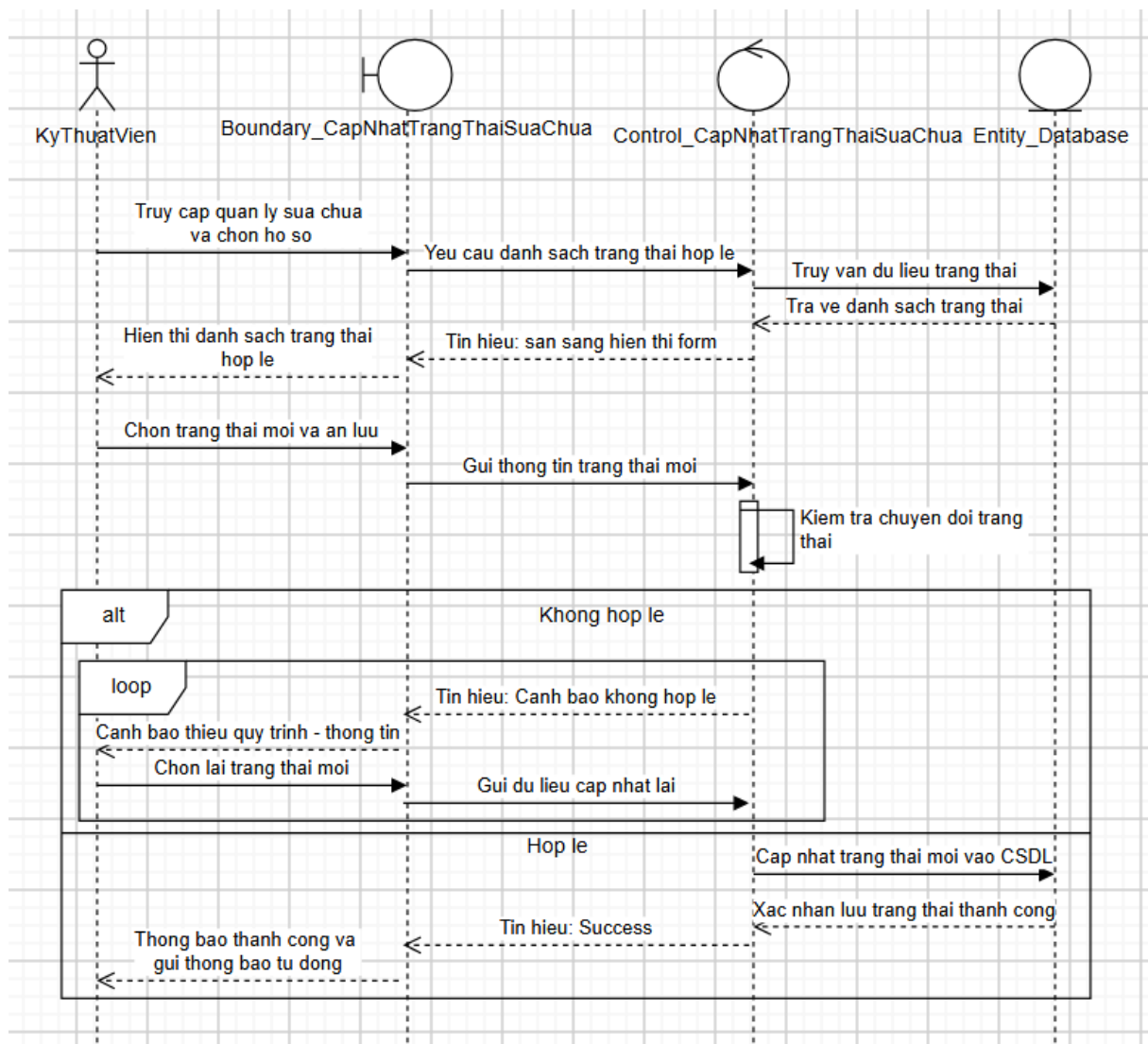
Biểu đồ tuần tự của Usecase “Cập nhật trạng thái sửa chữa”
