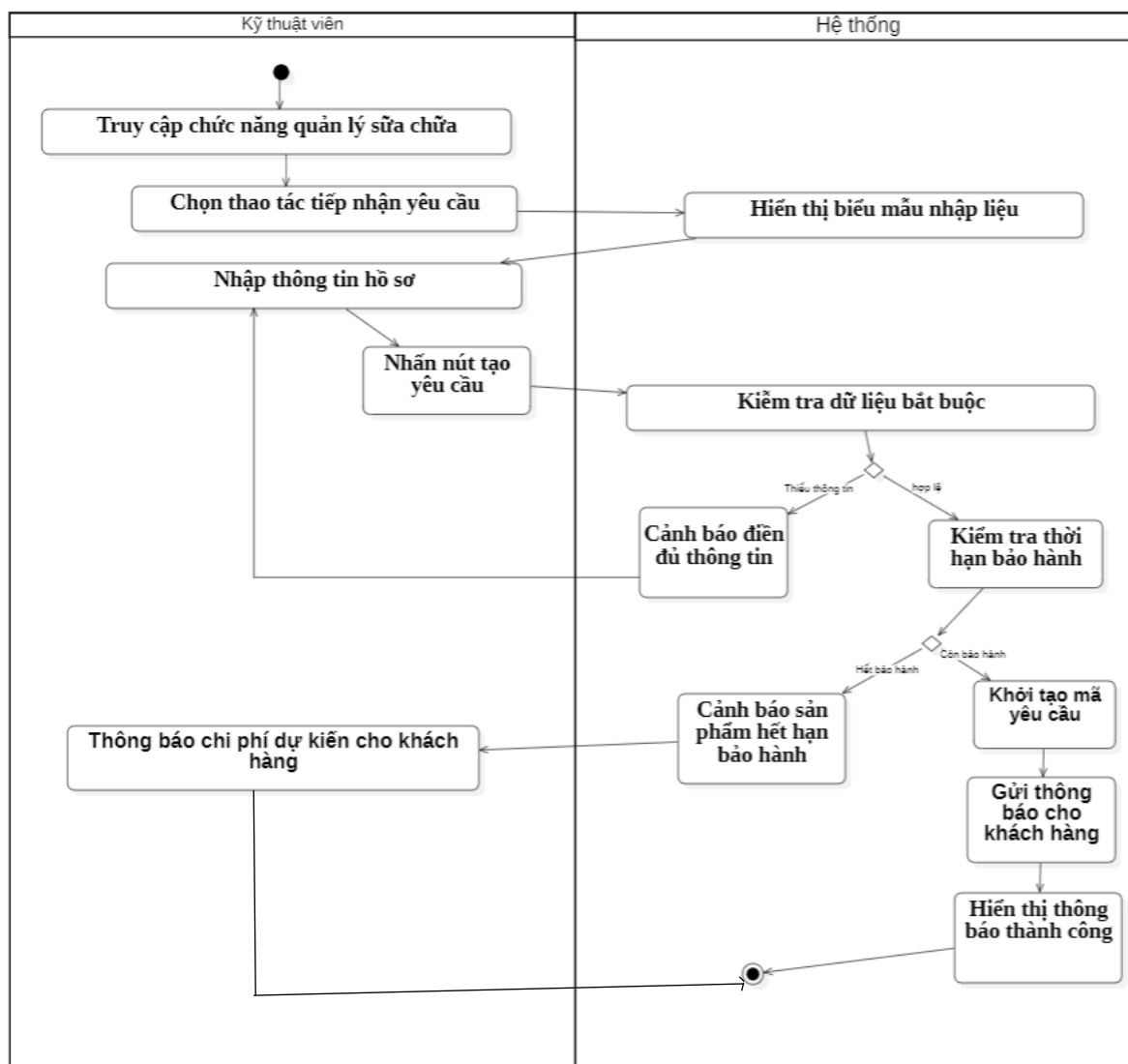
Biểu đồ hoạt động của Usecase “Tiếp nhận yêu cầu sửa chữa”
