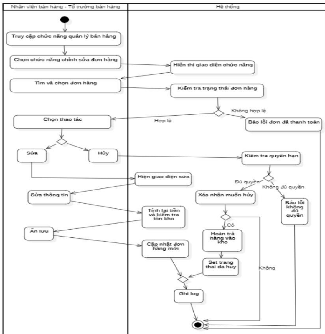
Biểu đồ hoạt động của Usecase “Hủy/chỉnh sửa đơn hàng”
