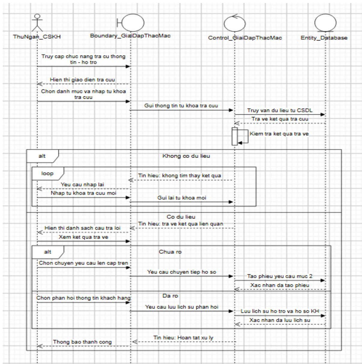
Biểu đồ tuần tự của Usecase “Giải đáp thắc mắc”
