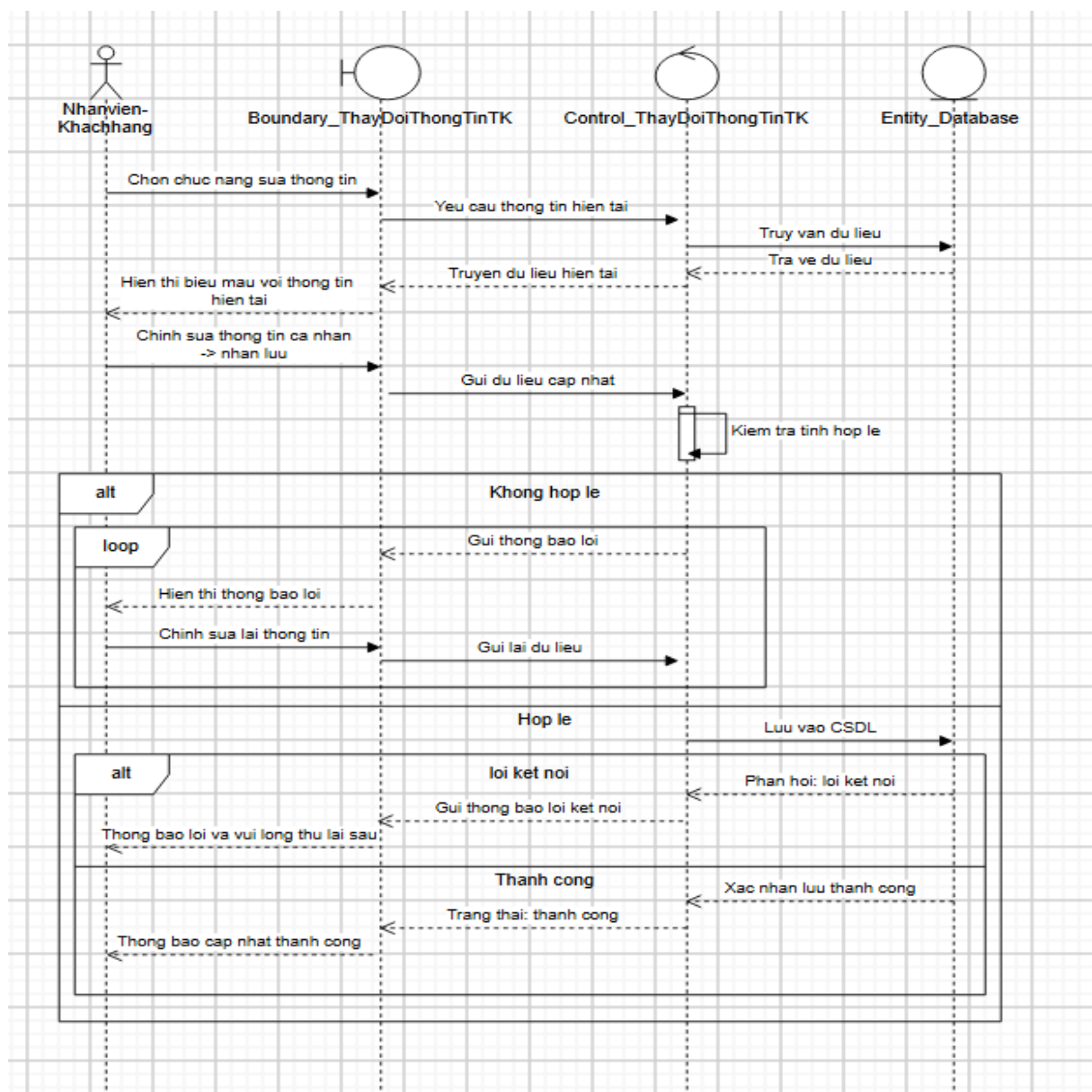
Biểu đồ tuần tự của Usecase “Thay đổi thông tin tài khoản”
