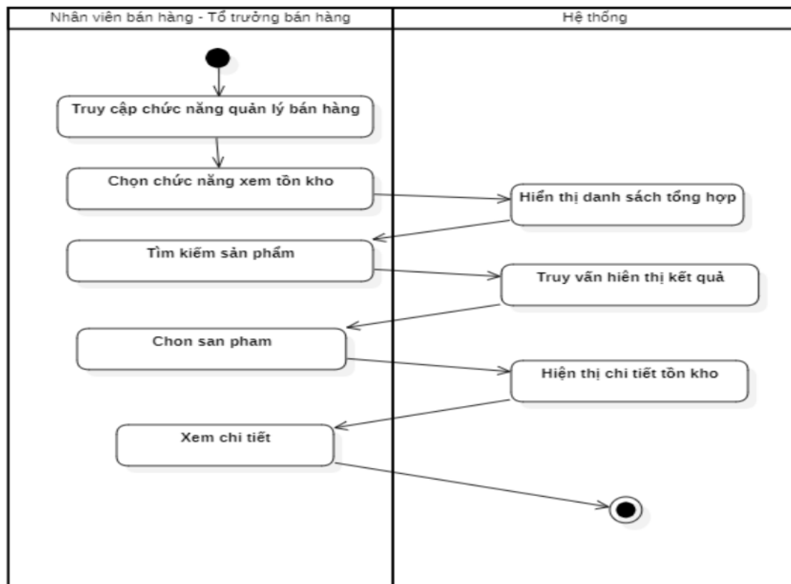
Biểu đồ hoạt động của Usecase “Xem tồn kho”
