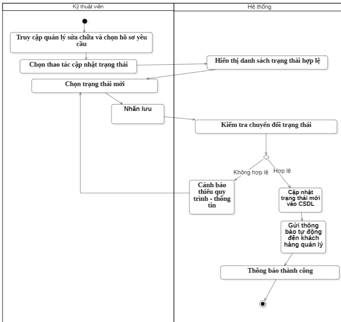
Biểu đồ hoạt động của Usecase “Cập nhật trạng thái sửa chữa”
