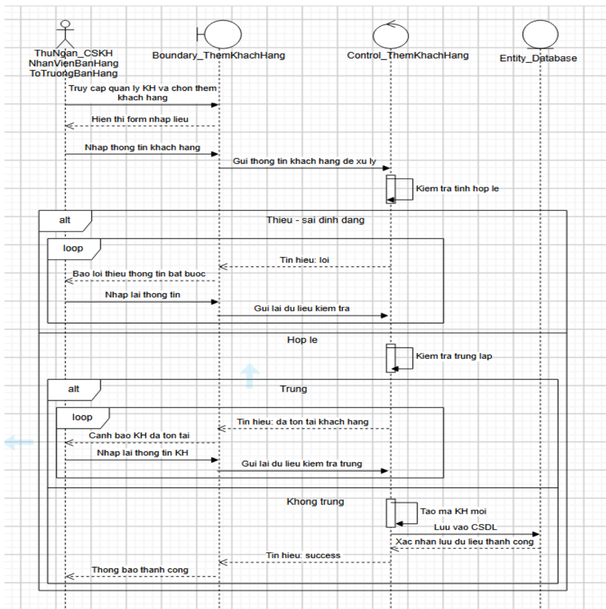
Biểu đồ tuần tự của Usecase “Thêm khách hàng”
