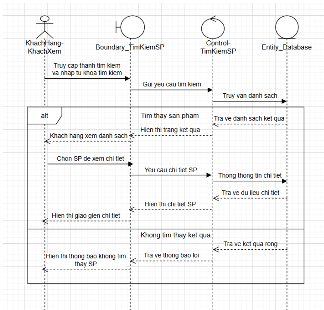
Biểu đồ tuần tự của Usecase “Tìm kiếm sản phẩm”
