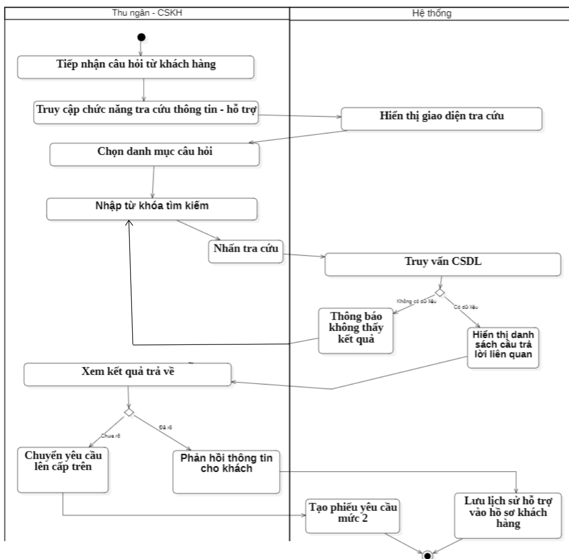
Biểu đồ hoạt động của Usecase “Giải đáp thắc mắc”
