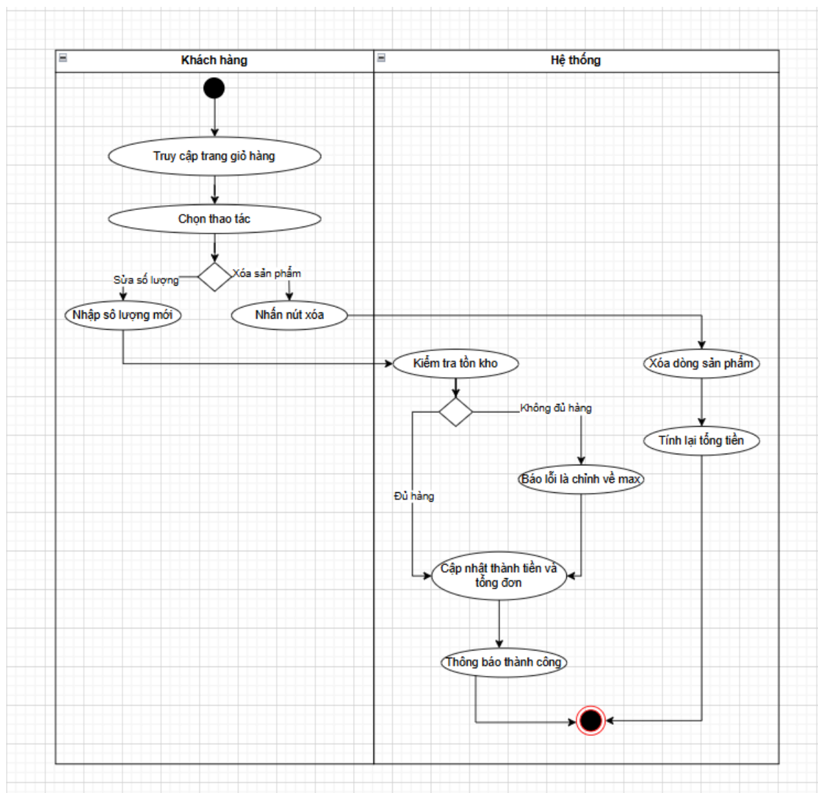
Biểu đồ hoạt động của Usecase “Quản lý giỏ hàng”
