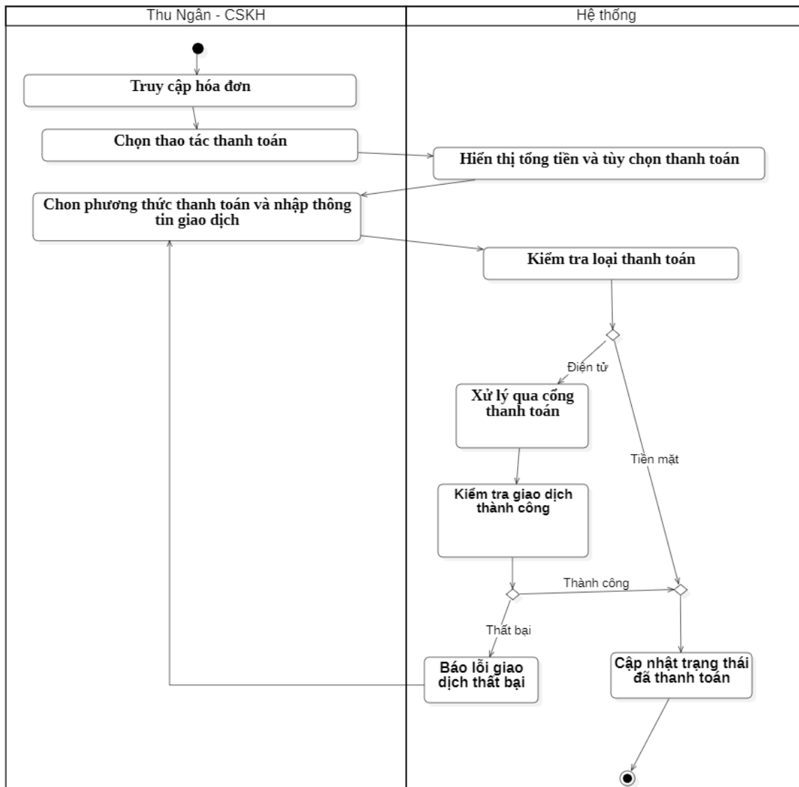
Biểu đồ hoạt động của Usecase “Thanh toán”
