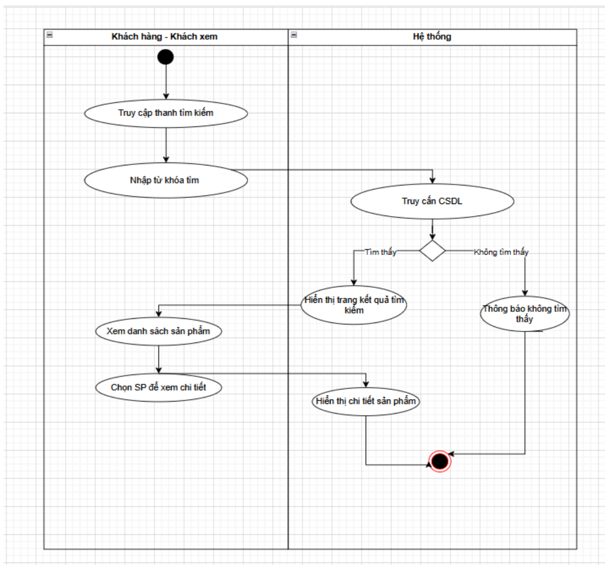
Biểu đồ hoạt động của Usecase “Tìm kiếm sản phẩm”
