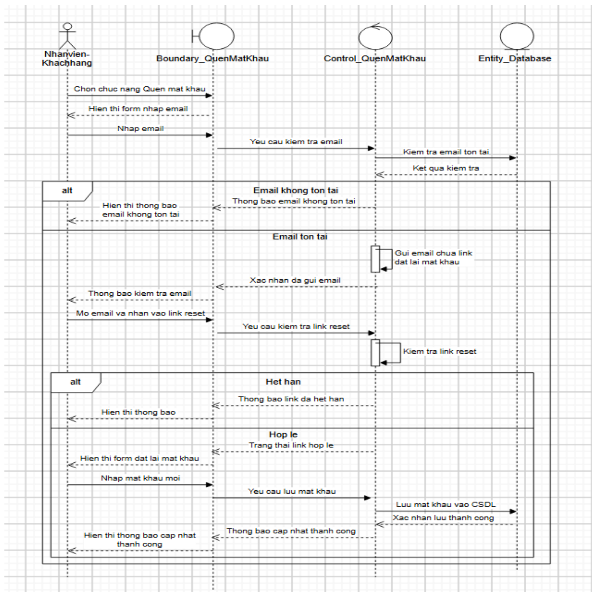
Biểu đồ tuần tự của Usecase “Quên mật khẩu”
