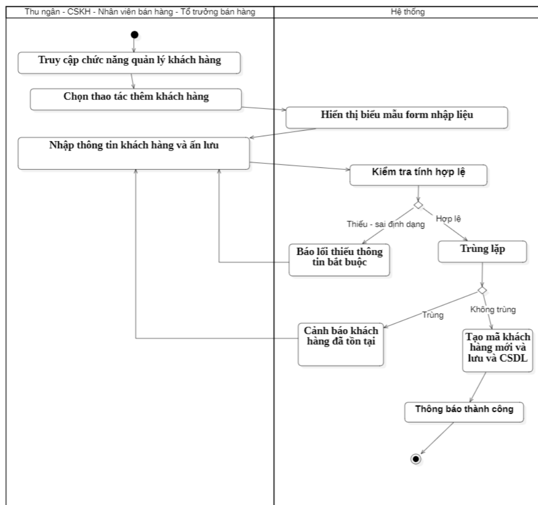
Biểu đồ hoạt động của Usecase “Thêm khách hàng”
