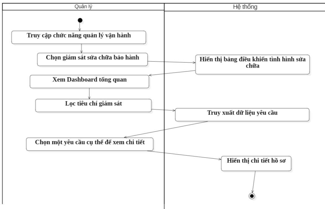
Biểu đồ hoạt động của Usecase “Giám sát sửa chữa - bảo hành”
