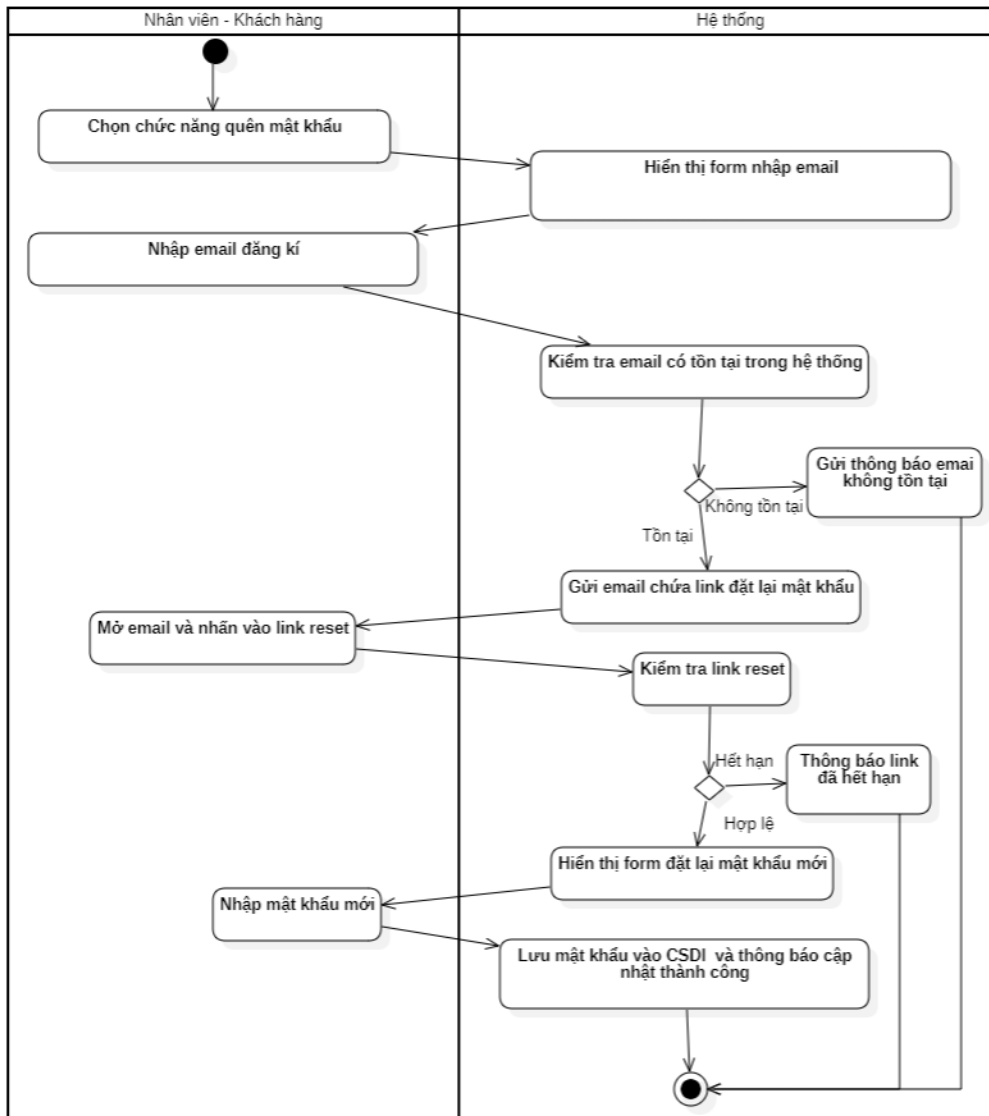
Biểu đồ hoạt động của Usecase “Quên mật khẩu”
