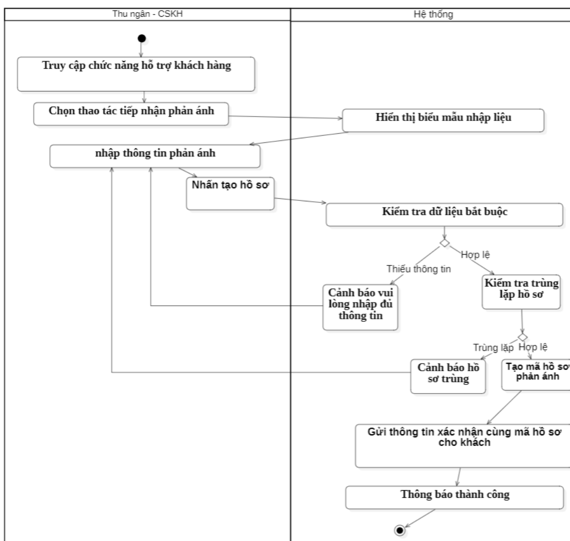
Biểu đồ hoạt động của Usecase “Tiếp nhận phản ánh”
