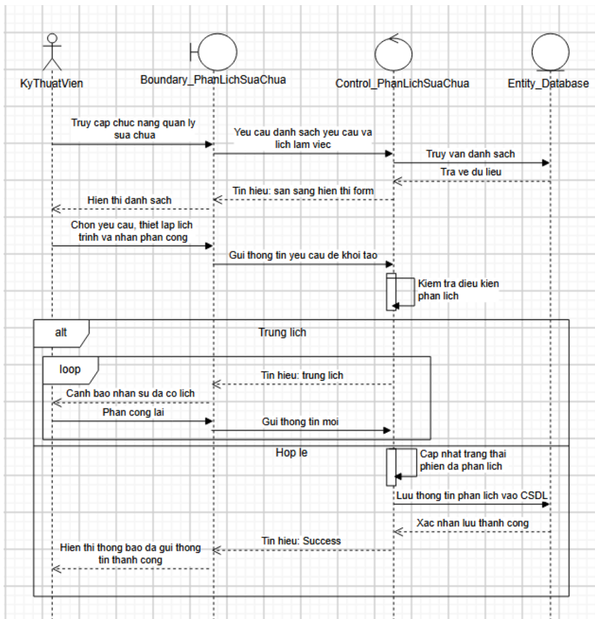
Biểu đồ tuần tự của Usecase “Phân lịch sửa chữa”
