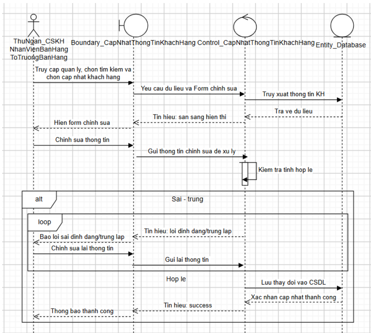
Biểu đồ tuần tự của Usecase “Cập nhật thông tin khách hàng”
