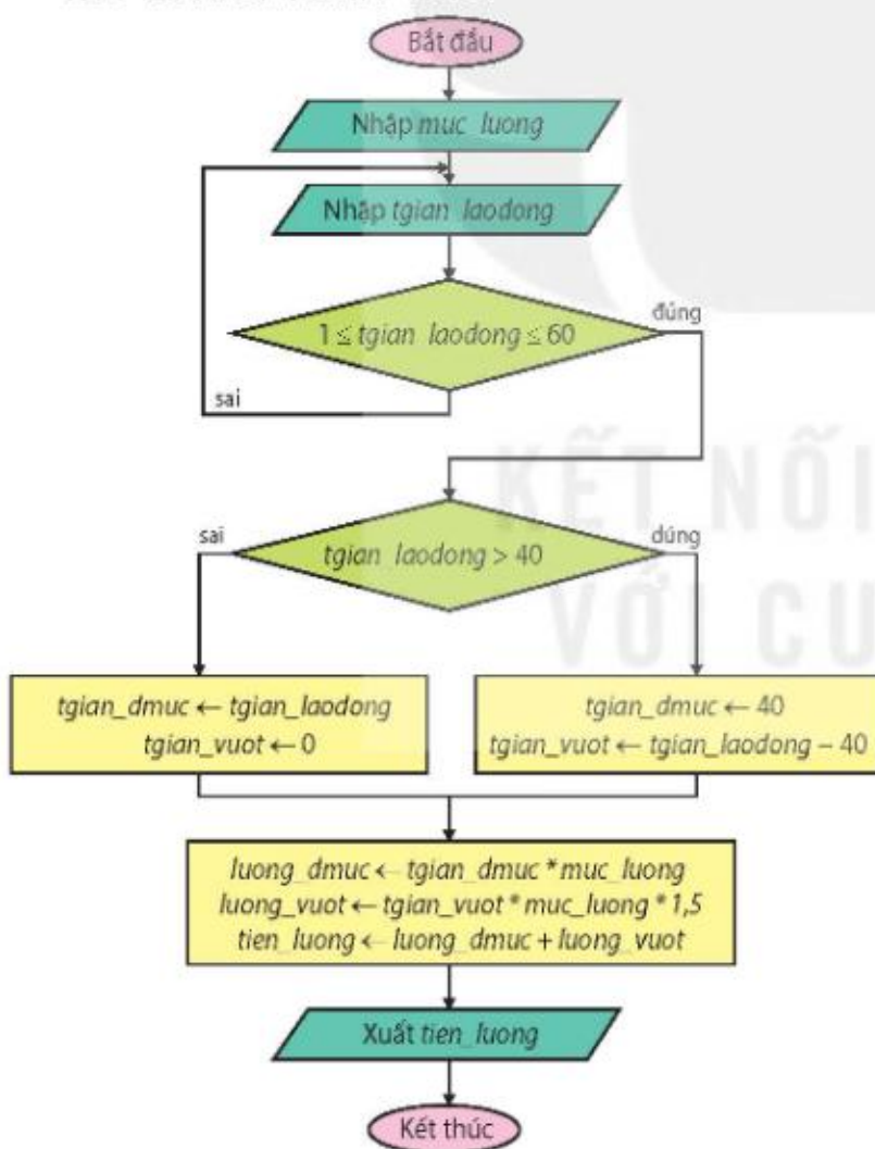
Hình 15.3. Thuật toán tính lương
