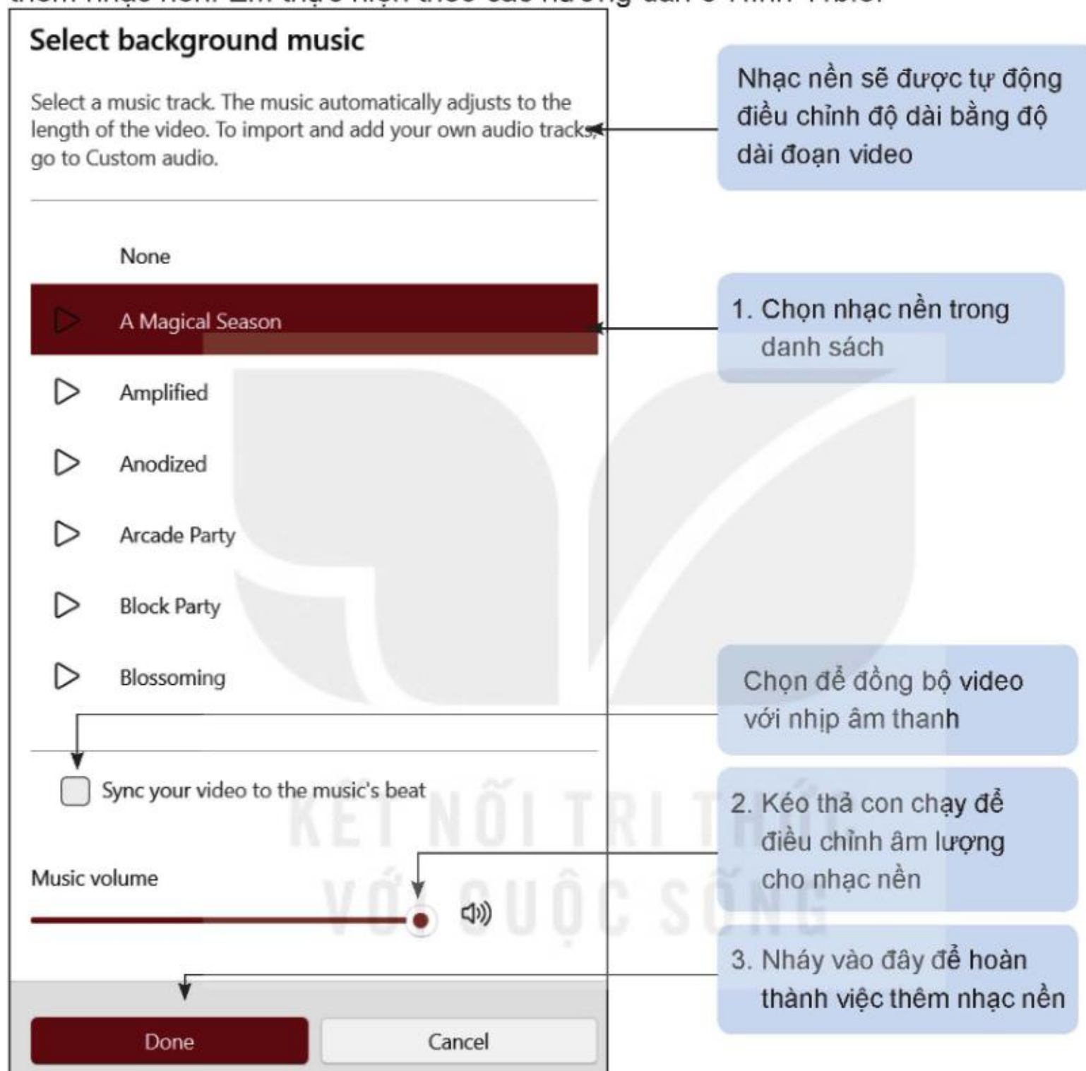
Hình 11b.5. Các thao tác chọn nhạc nền
