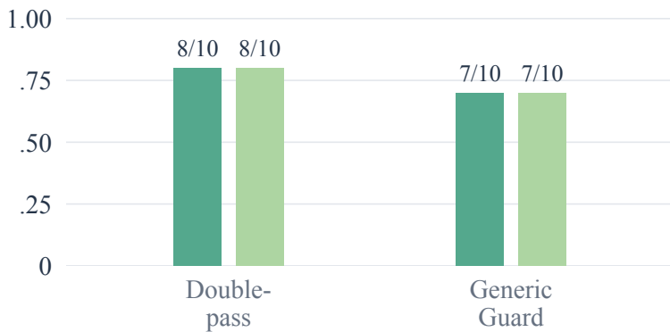
Repeated poisoning · p=1 · n=10
