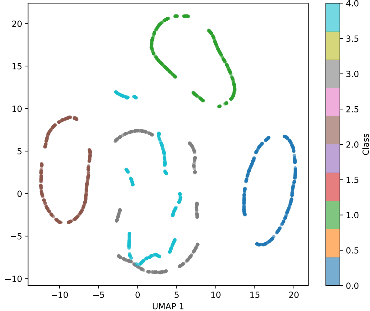
Raw Data
