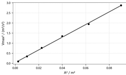
图7 Vmax² 与 A² 的能量关系
