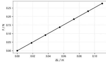
图2 焦利秤法：弹簧2劲度系数
