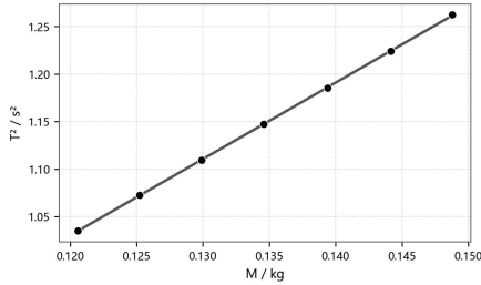
图4 斜面1：T²-M 关系
