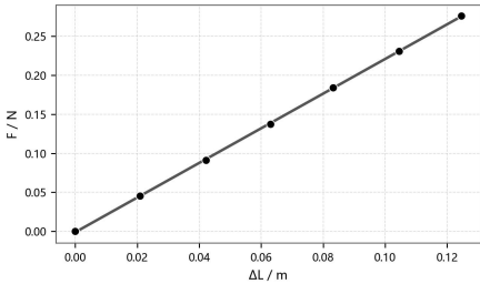
图1 焦利秤法：弹簧1劲度系数
