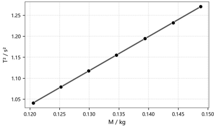
图3 水平状态：T²-M 关系
