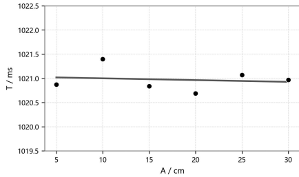
图6 振幅 A 与周期 T 的关系
