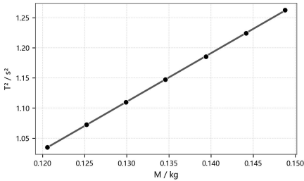
图5 斜面2：T²-M 关系
