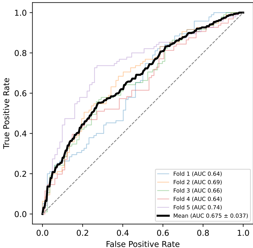
ROC — AAL (v2)
