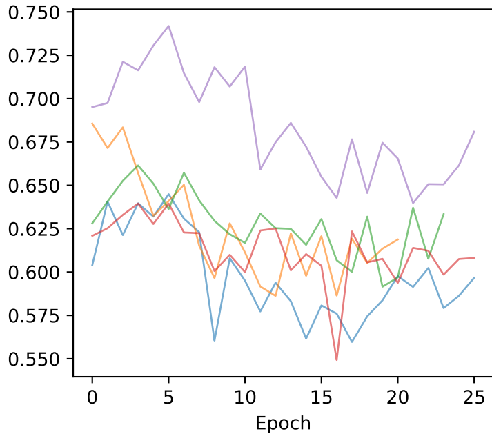
Validation AUC
