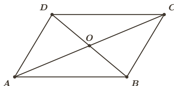
Parallelogram: AO = OC and BO = OD
