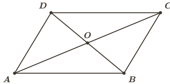
Parallelogram ABCD: AO = OC and BO = OD
