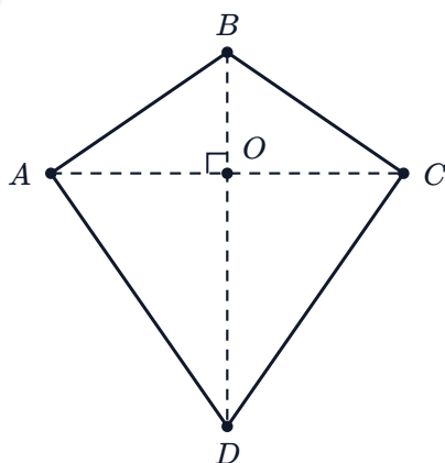
Kite: AB = BC and CD = DA
