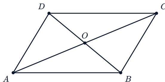
Parallelogram: AO = OC and BO = OD
