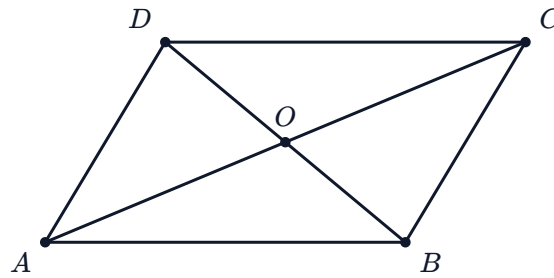
Parallelogram ABCD: AO = OC and BO = OD
