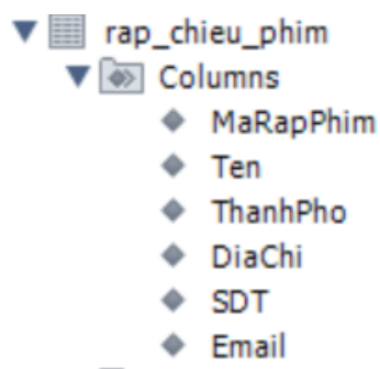
Hình 4: Các cột của bảng RAP_CHIEU_PHIM sau khi chạy lệnh
