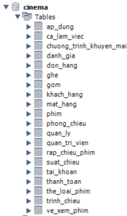
Hình 3: Các bảng được tạo sau khi chạy lệnh
