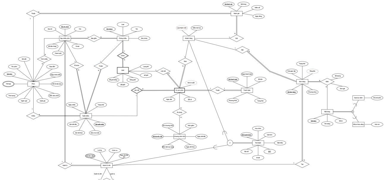
Hình 6: Sơ đồ EERD của hệ thống rạp chiếu phim.
