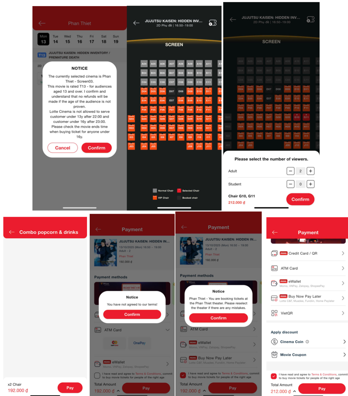
Hình 4: Giao diện chọn ghế và thanh toán – minh họa luồng đặt vé trực tuyến
