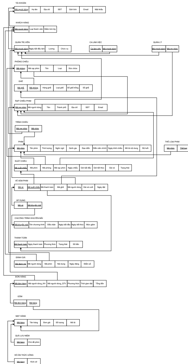
Hình 7: Ảnh xạ sang CSDL cho sơ đồ EERD của hệ thống rạp chiếu phim.
