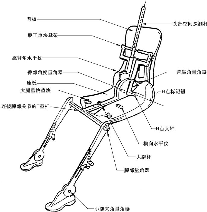
图 A.1 3-D H 装置构件名称
