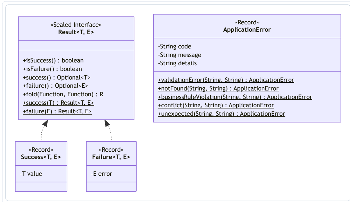
Figura 3: Diagrama de la Capa de Aplicación – Shared Kernel
