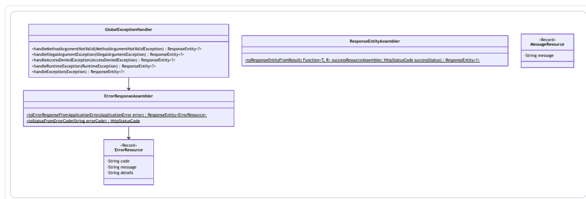
Figura 2: Diagrama de la Capa de Interfaz – Shared Kernel
