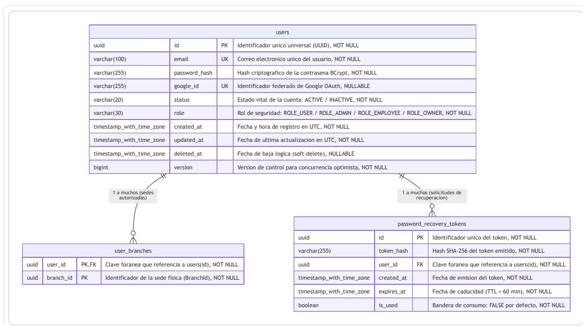
Figura 13: Diagrama de Base de Datos Relacional ER – IAM
