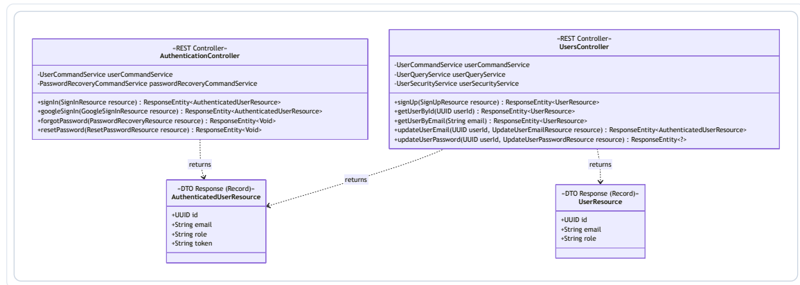
Figura 9: Diagrama de la Capa de Interfaces – IAM
