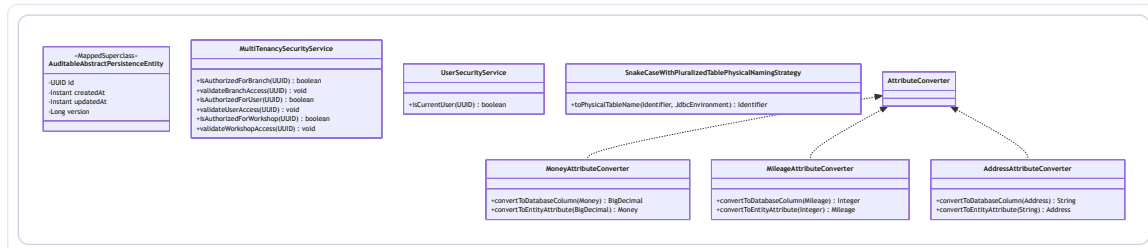
Figura 4: Diagrama de la Capa de Infraestructura – Shared Kernel
