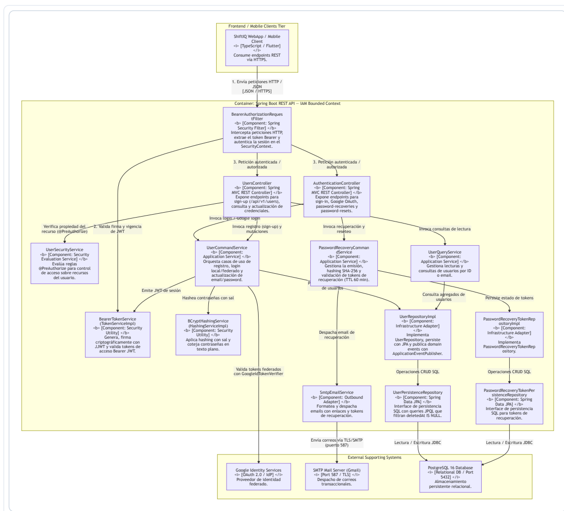
Figura 11: Diagrama de Componentes C4 Nivel 3 – IAM
