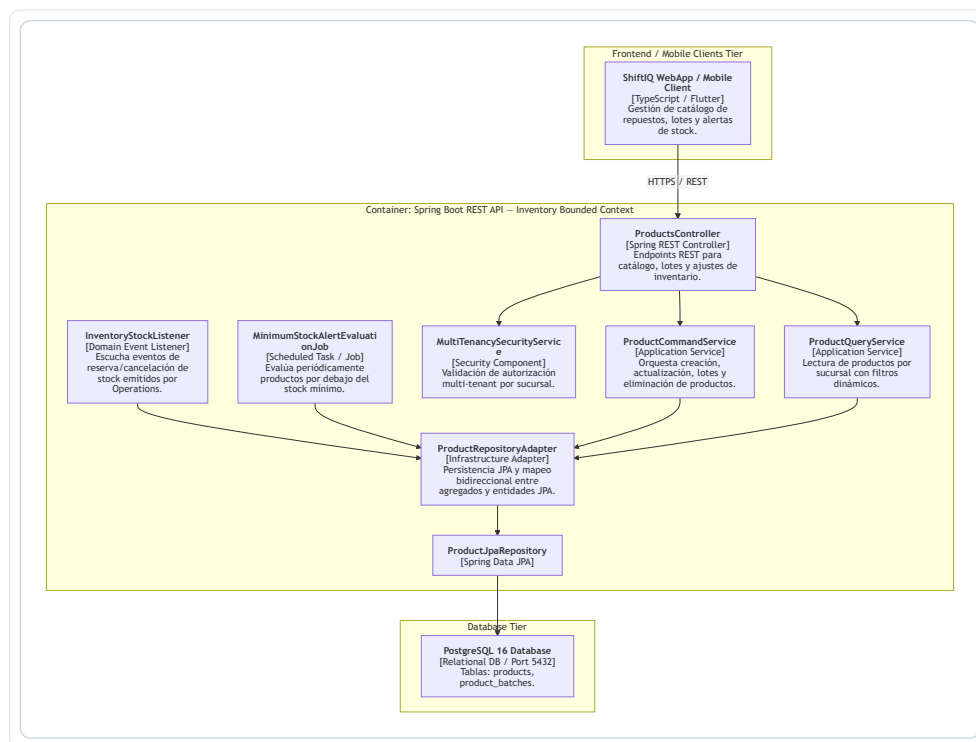
Figura 60: Diagrama de Componentes C4 Nivel 3 – Inventory
