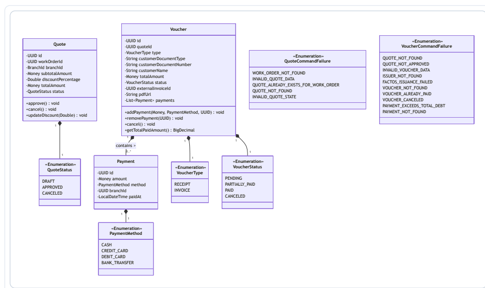
Figura 84: Diagrama de la Capa de Dominio – Billing
