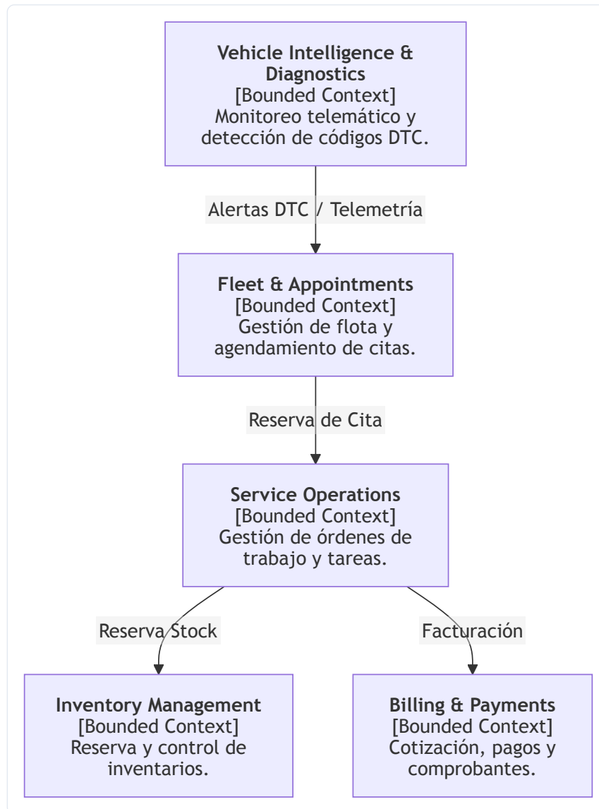
Figura 32: Flujo de interacción entre Bounded Contexts en el proceso de servicio automotriz.
