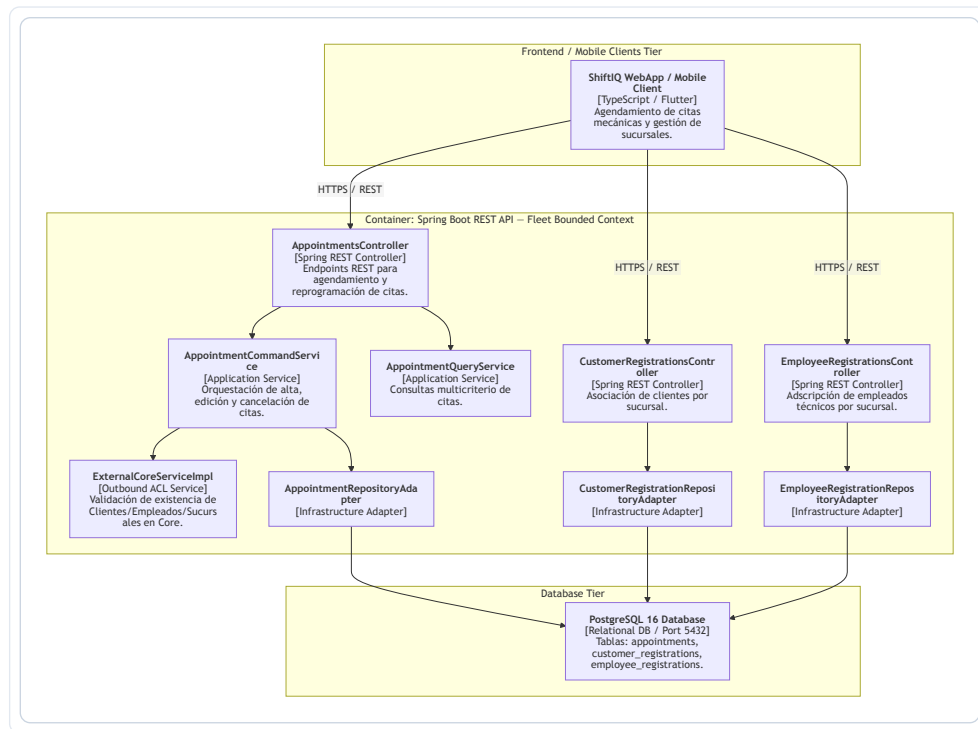
Figura 81: Diagrama de Componentes C4 Nivel 3 – Fleet
