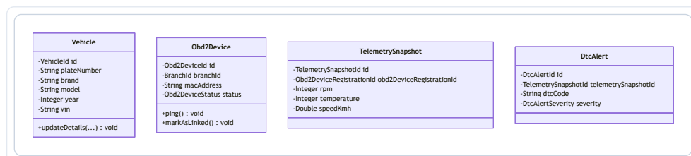
Figura 68: Diagrama de Clases del Dominio UML – IoT
