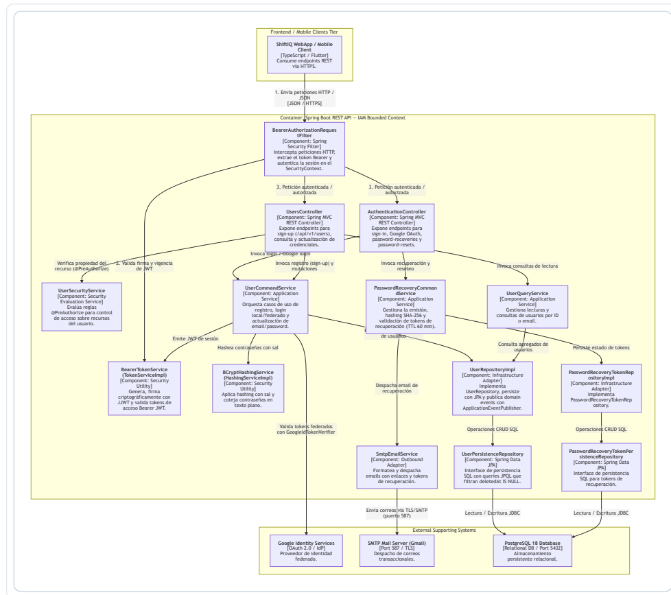
Figura 46: Diagrama de Componentes C4 Nivel 3 – IAM
