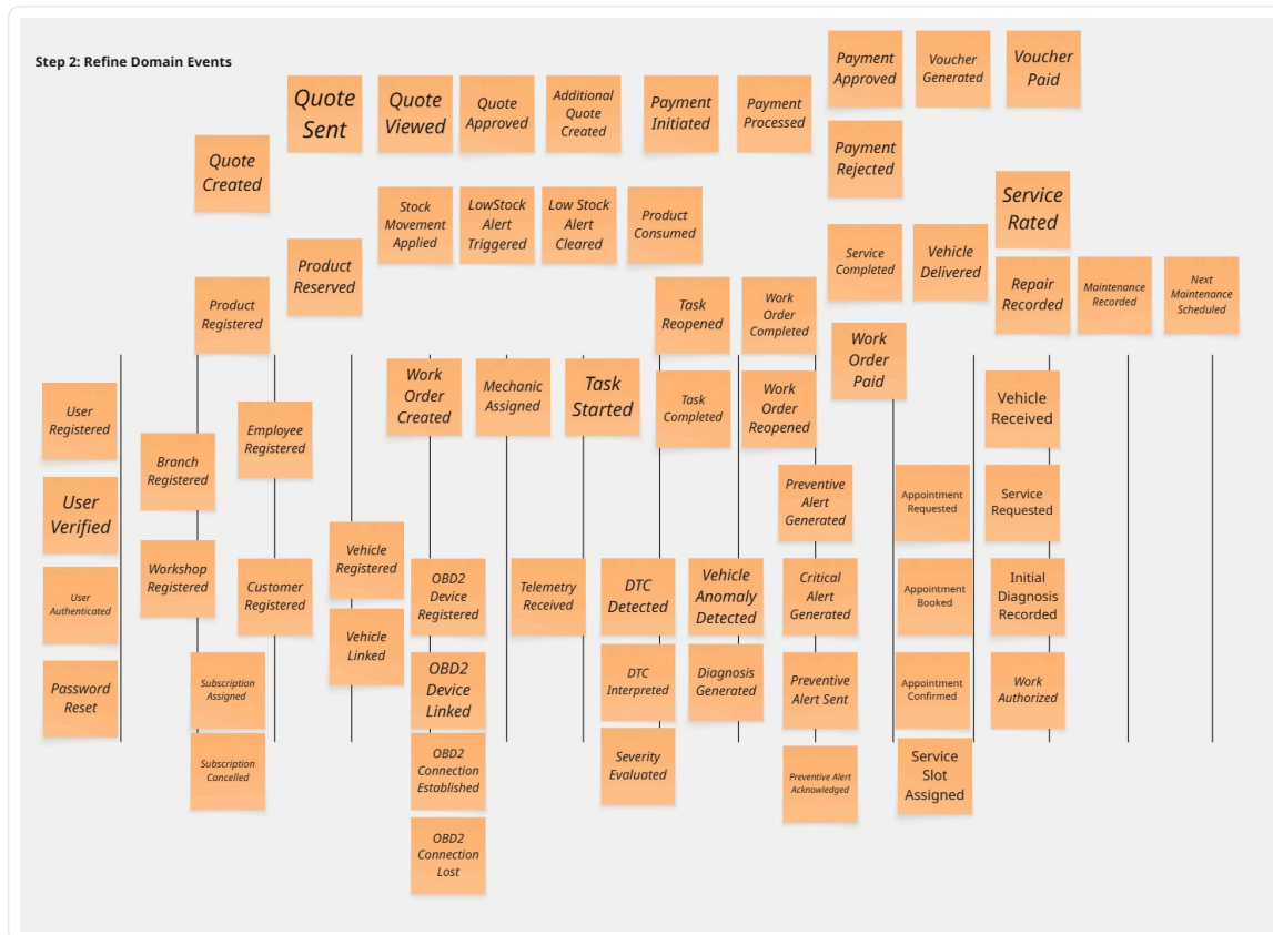
Figura 8: Refine Domain – Refinamiento y organización de los eventos del dominio.
