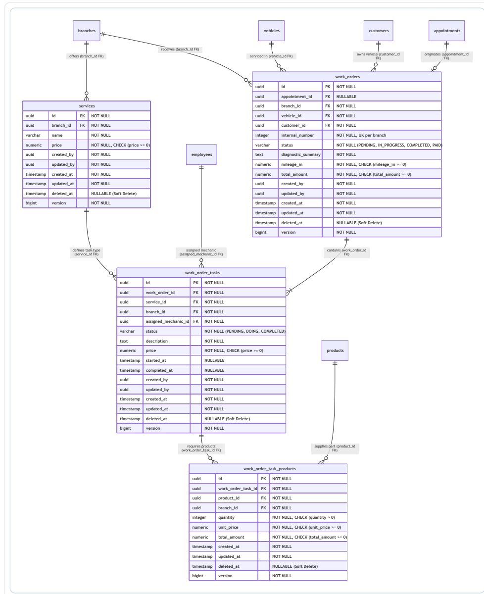
Figura 55: Diagrama de Base de Datos Relacional ER – Operations
