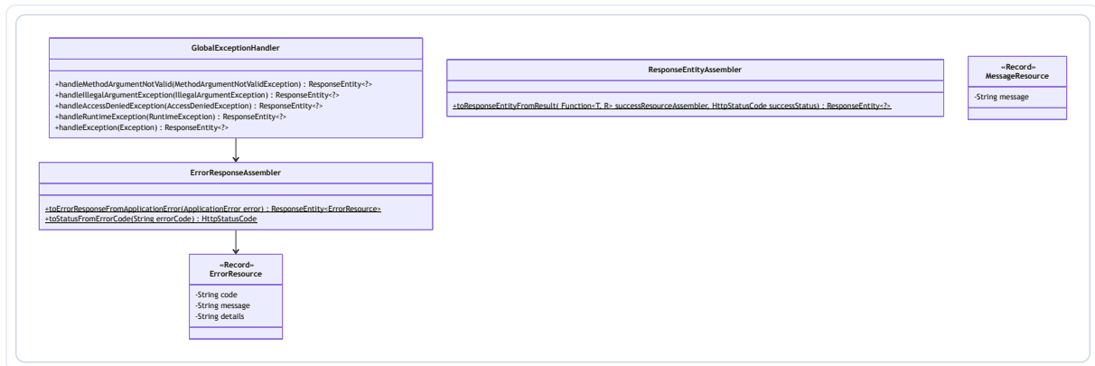
Figura 37: Diagrama de la Capa de Interfaz – Shared Kernel
