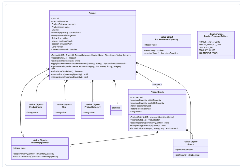
Figura 56: Diagrama de la Capa de Dominio – Inventory
