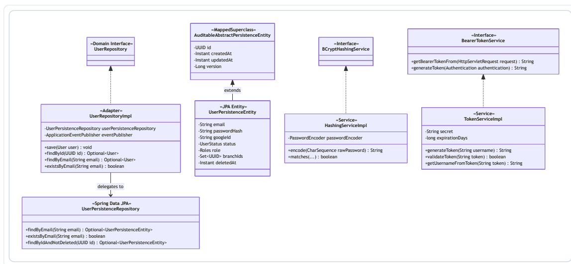
Figura 45: Diagrama de la Capa de Infraestructura – IAM
