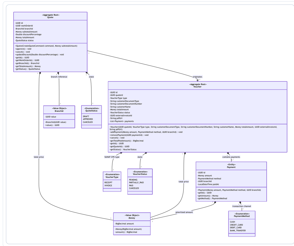
Figura 89: Diagrama de Clases del Dominio UML – Billing
