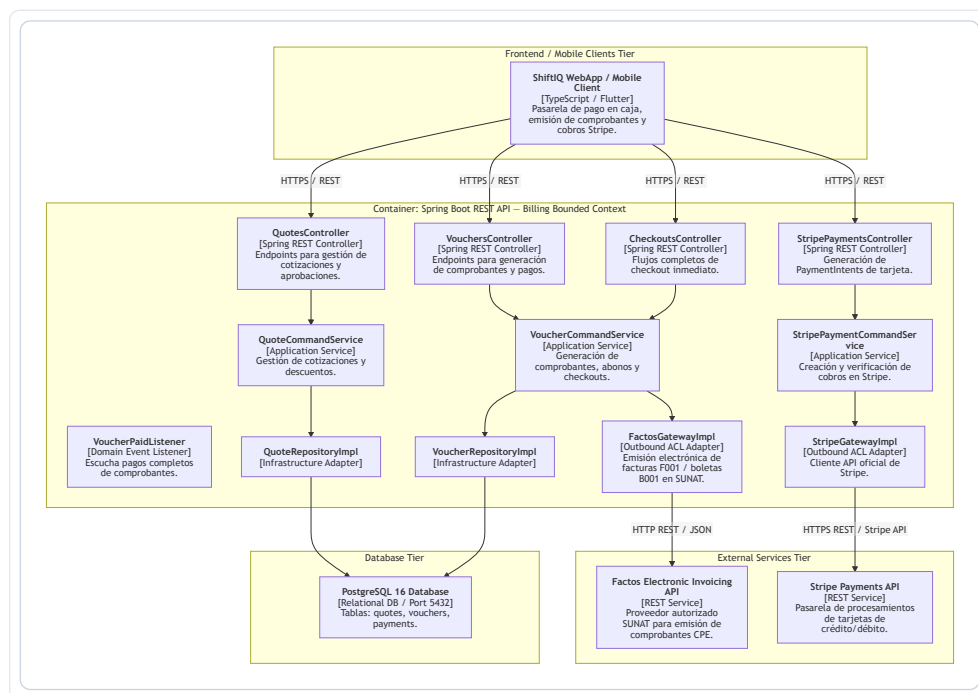
Figura 88: Diagrama de Componentes C4 Nivel 3 – Billing
