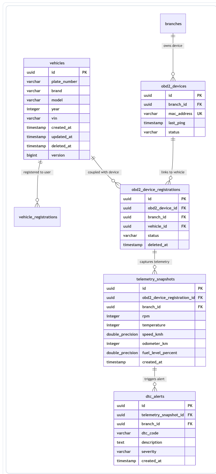
Figura 69: Diagrama de Base de Datos Relacional ER – IoT
