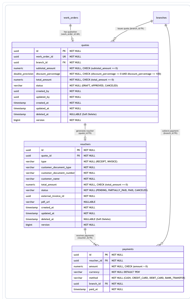
Figura 90: Diagrama de Base de Datos Relacional ER – Billing
