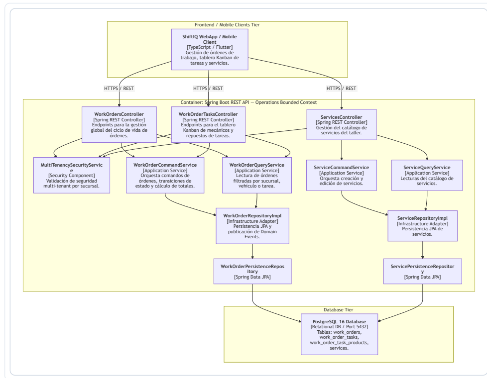
Figura 53: Diagrama de Componentes C4 Nivel 3 – Operations
