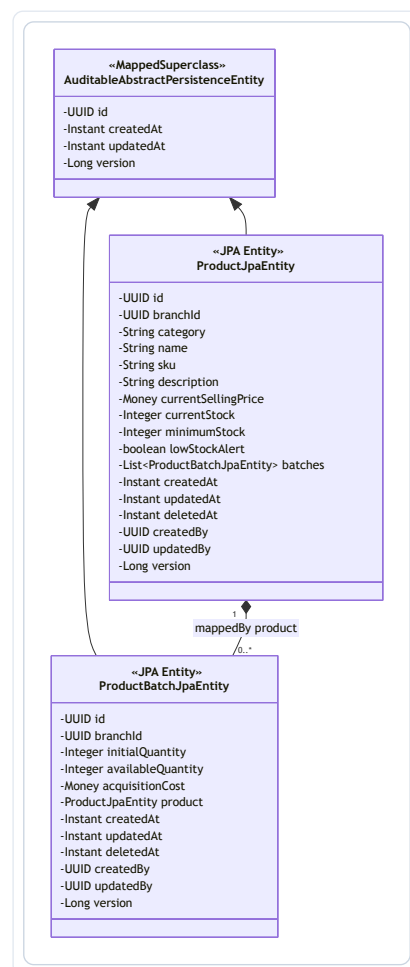
Figura 59: Diagrama de la Capa de Infraestructura – Inventory
