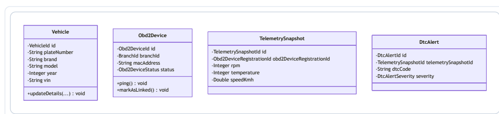
Figura 66: Diagrama de Clases del Dominio UML – IoT
