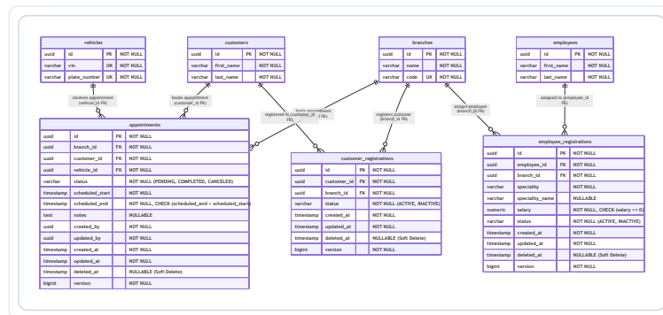
Figura 81: Diagrama de Base de Datos Relacional ER – Fleet
