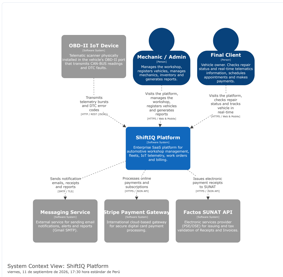
Figura 31: Diagrama de Contexto del Sistema – ShiftIQ Platform.
