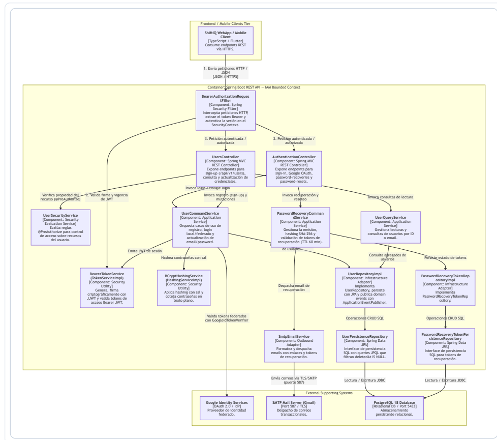
Figura 44: Diagrama de Componentes C4 Nivel 3 – IAM
