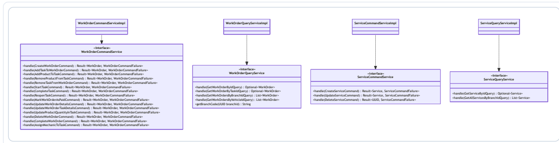
Figura 48: Diagrama de la Capa de Aplicación – Operations
