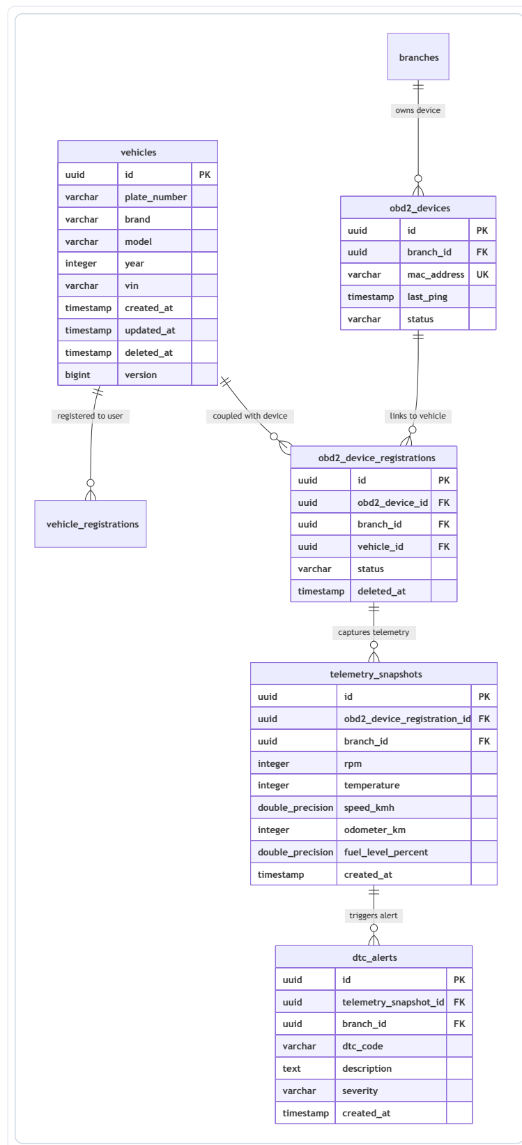
Figura 67: Diagrama de Base de Datos Relacional ER – IoT
