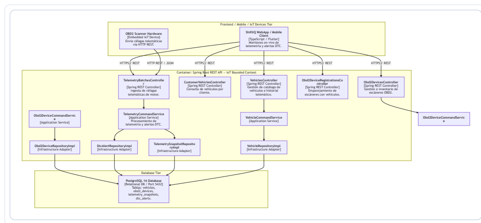
Figura 65: Diagrama de Componentes C4 Nivel 3 – IoT
