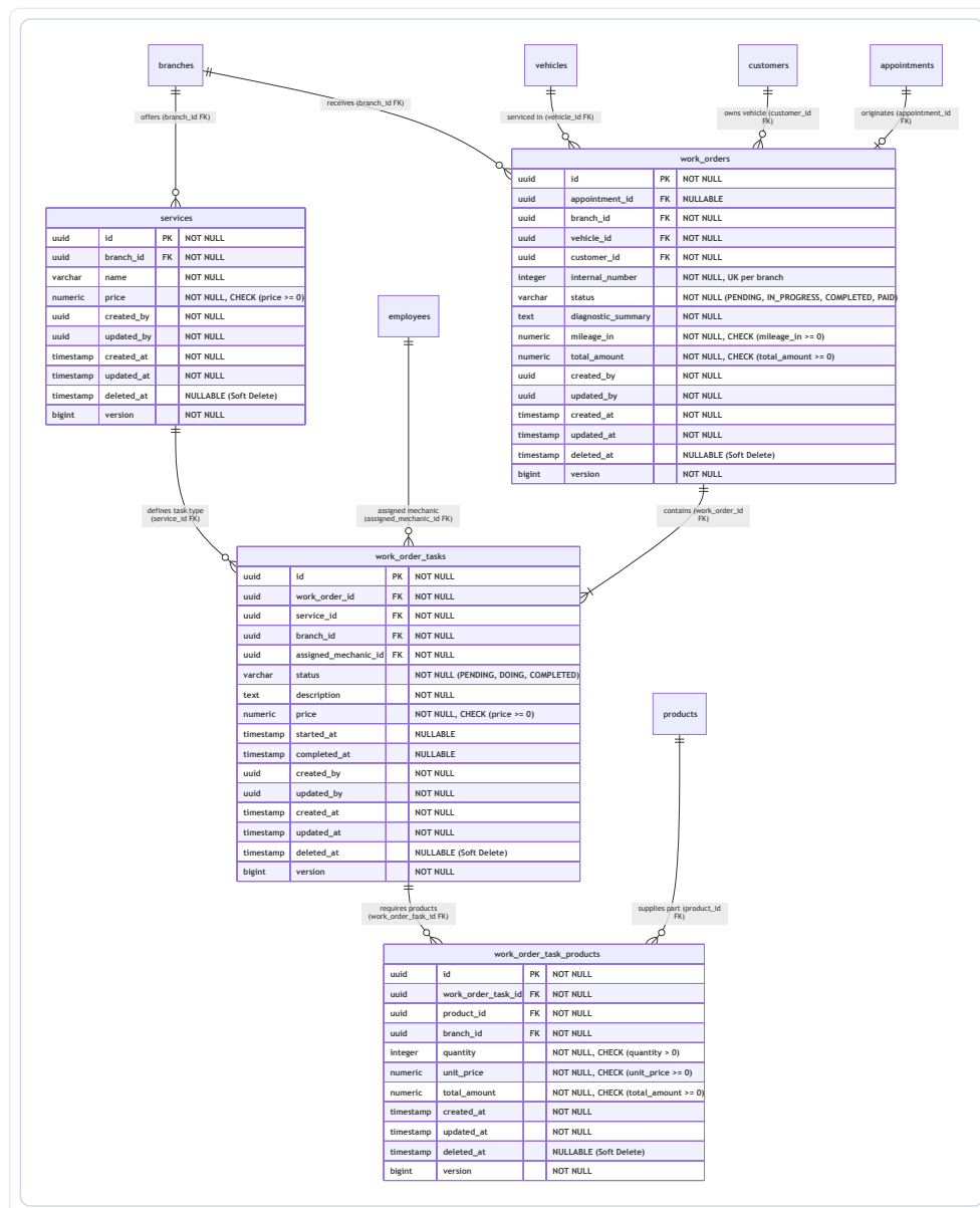
Figura 53: Diagrama de Base de Datos Relacional ER – Operations
