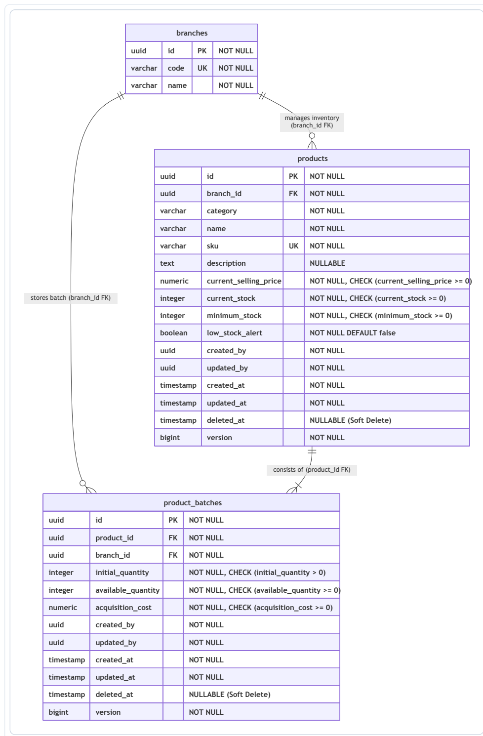
Figura 60: Diagrama de Base de Datos Relacional ER – Inventory
