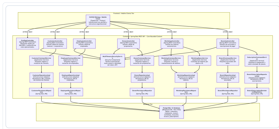
Figura 72: Diagrama de Componentes C4 Nivel 3 – Core
