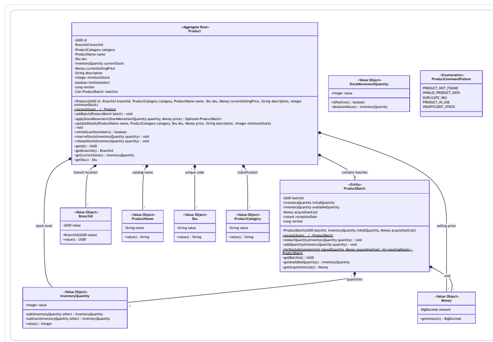
Figura 59: Diagrama de Clases del Dominio UML – Inventory
