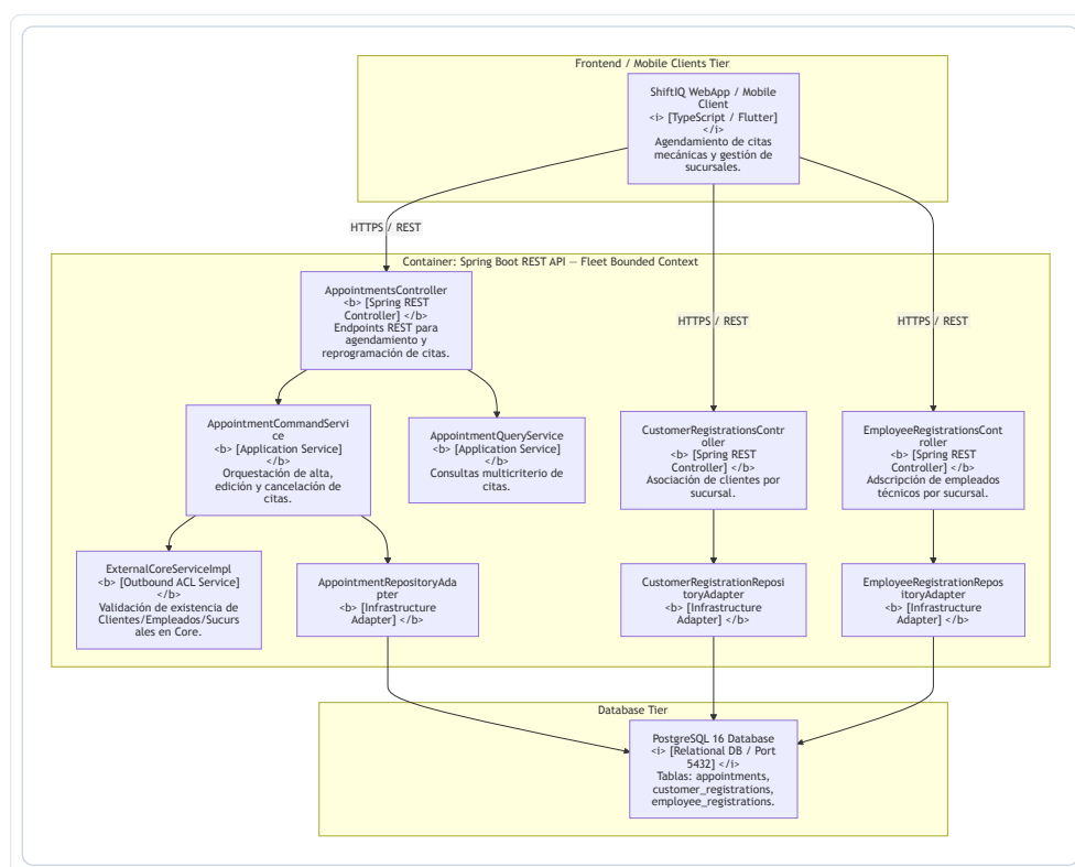
Figura 74: Diagrama de Componentes C4 Nivel 3 – Fleet
