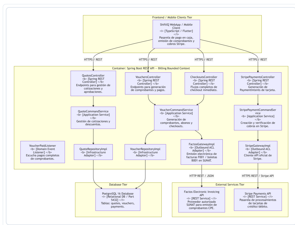
Figura 81: Diagrama de Componentes C4 Nivel 3 – Billing
