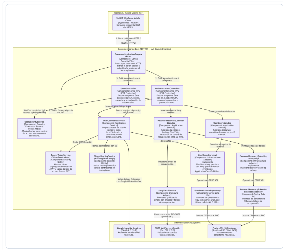
Figura 45: Diagrama de Componentes C4 Nivel 3 – IAM
