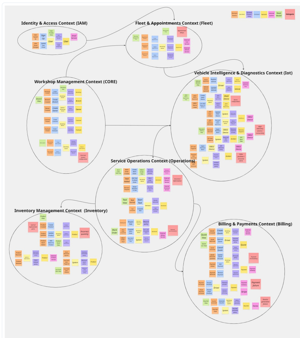
Figura 9: Candidate Context Discovery – Reconocimiento de los Candidate Bounded Contexts de ShiftIQ.
