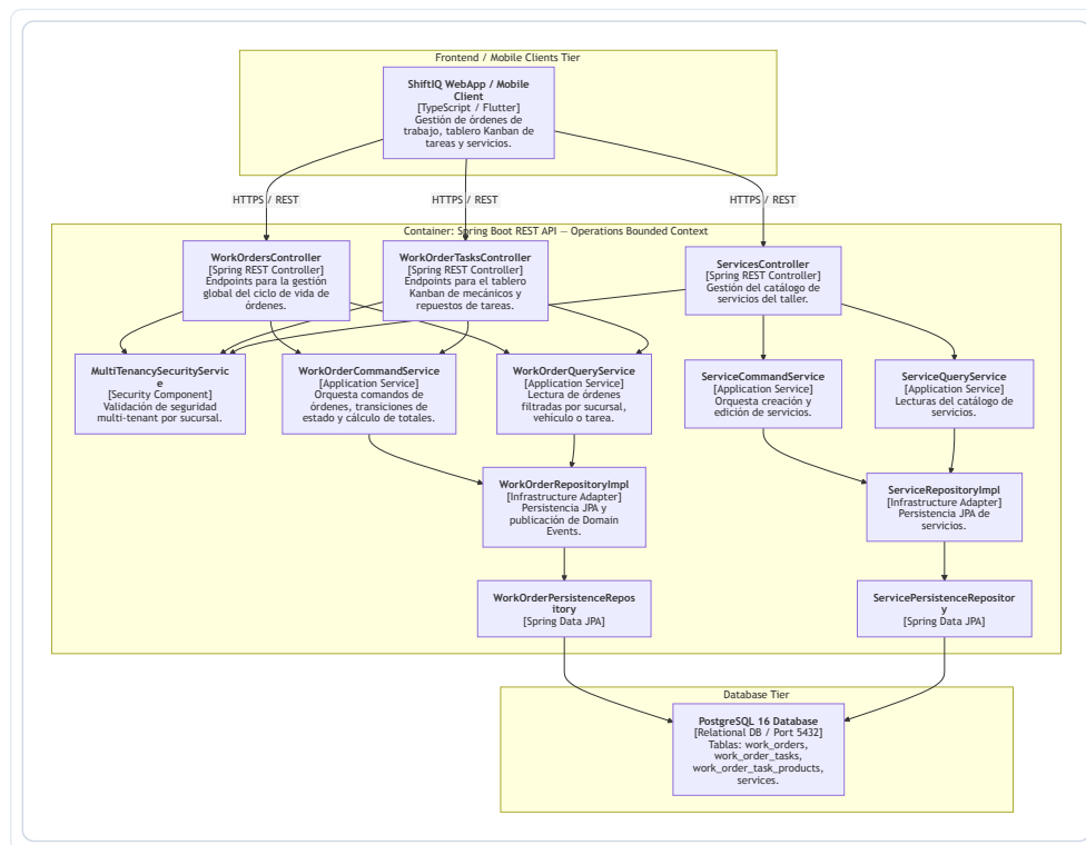
Figura 52: Diagrama de Componentes C4 Nivel 3 – Operations
