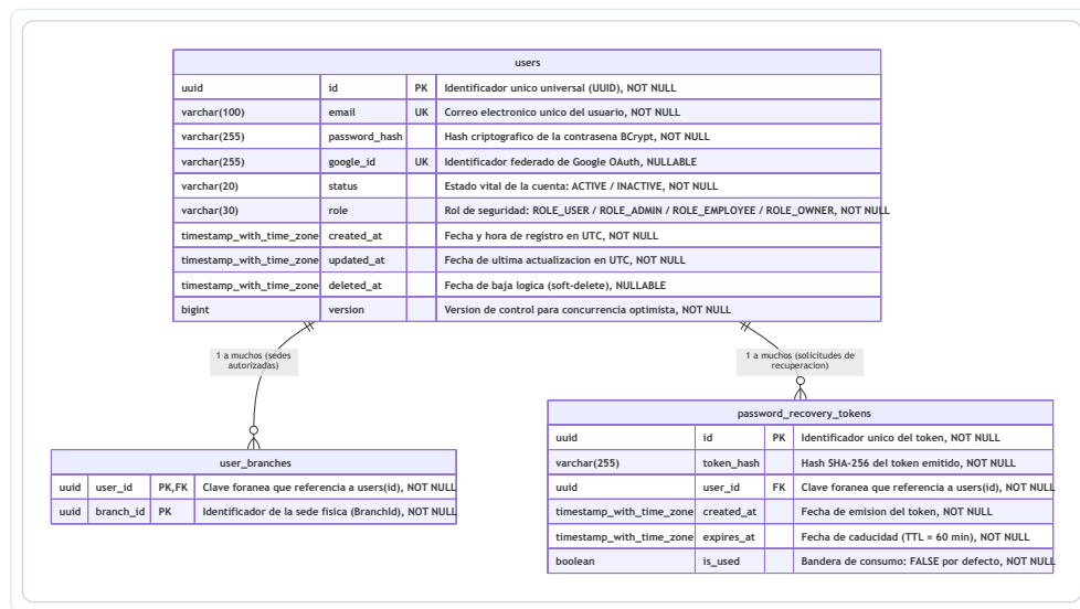
Figura 47: Diagrama de Base de Datos Relacional ER – IAM
