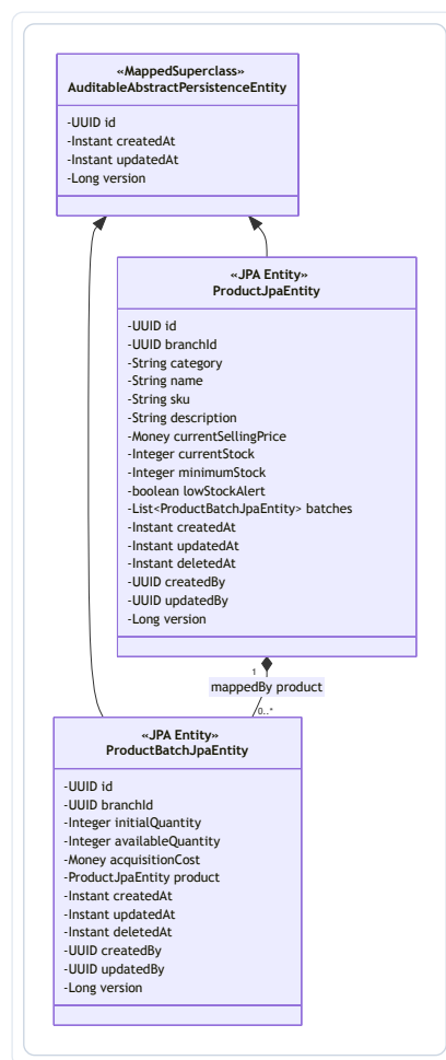
Figura 58: Diagrama de la Capa de Infraestructura – Inventory
