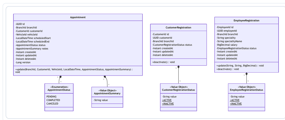
Figura 76: Diagrama de la Capa de Dominio – Fleet
