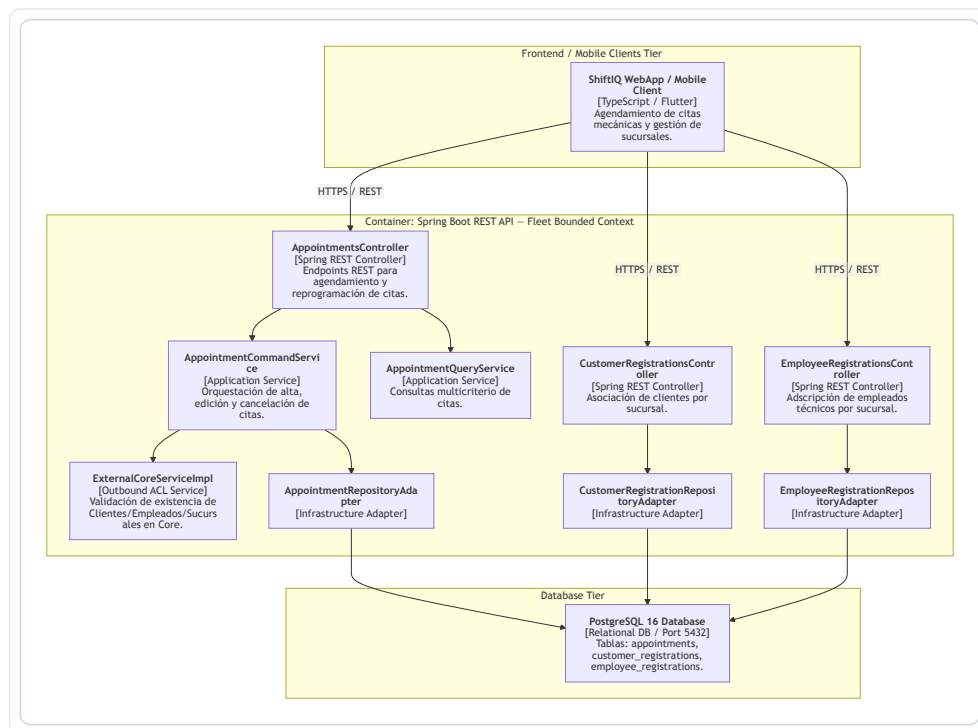
Figura 80: Diagrama de Componentes C4 Nivel 3 – Fleet
