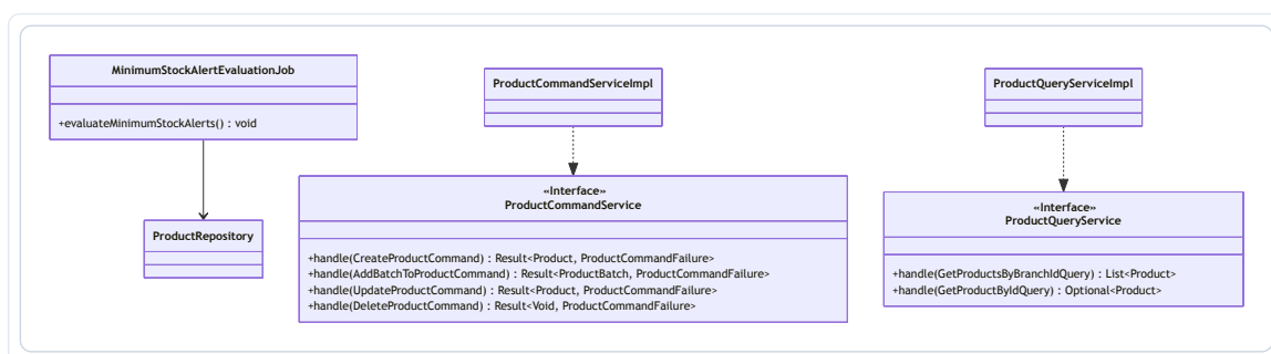
Figura 56: Diagrama de la Capa de Aplicación – Inventory
