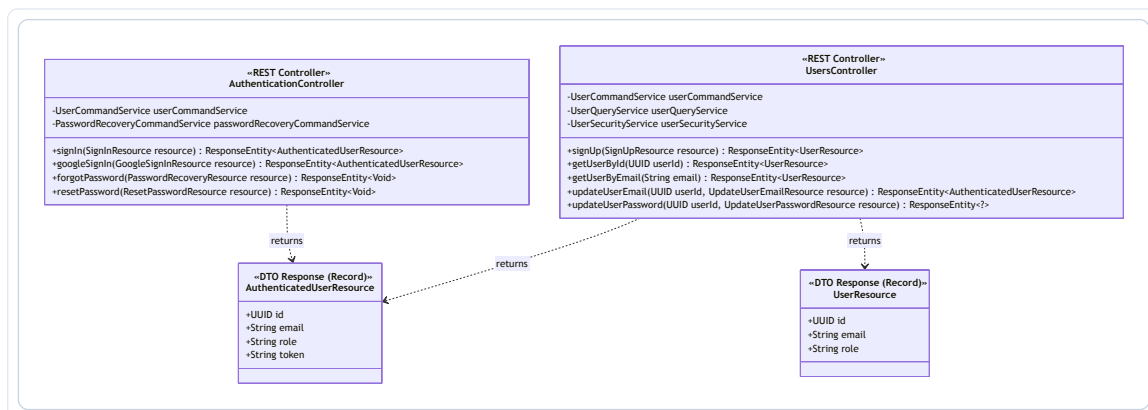
Figura 43: Diagrama de la Capa de Interfaces – IAM
