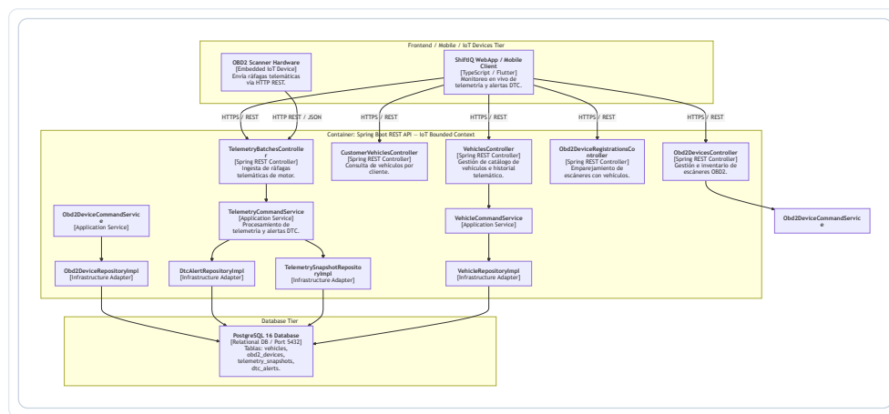
Figura 66: Diagrama de Componentes C4 Nivel 3 – IoT
