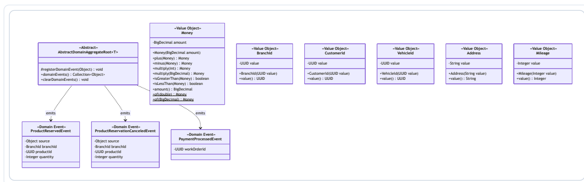
Figura 35: Diagrama de la Capa de Dominio – Shared Kernel
