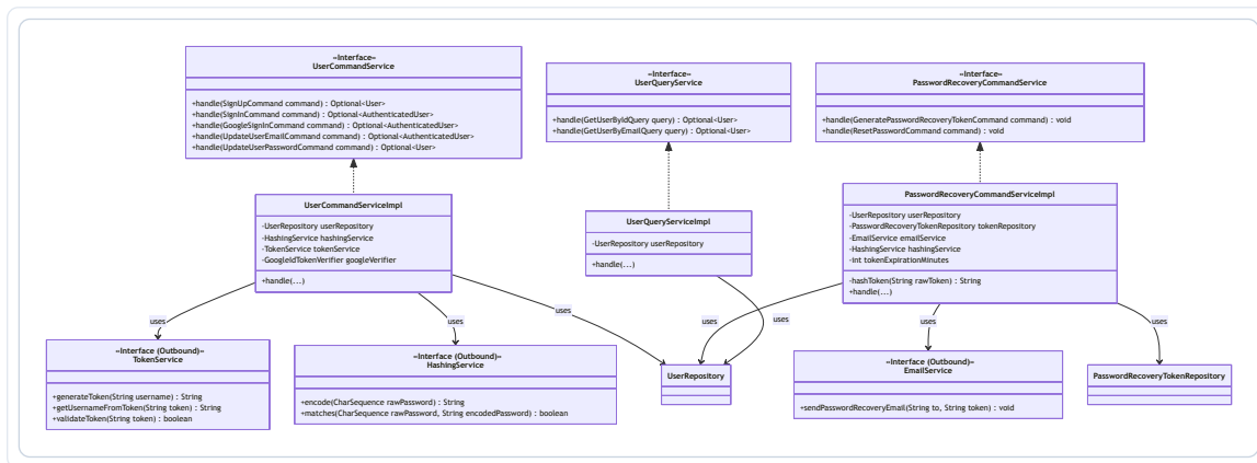
Figura 42: Diagrama de la Capa de Aplicación – IAM
