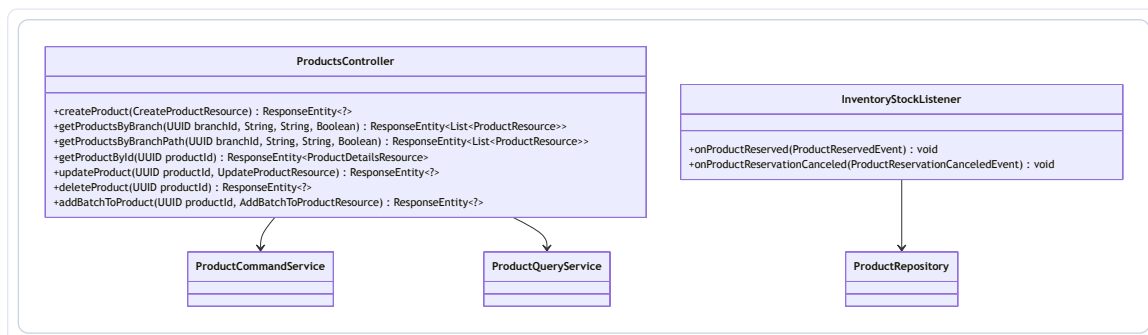
Figura 57: Diagrama de la Capa de Interfaz – Inventory
