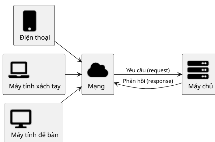
Hình 4.1: Mô hình kiến trúc khách–chủ
