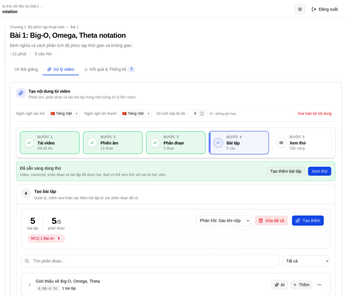
Hình 5.6: Giao diện quản lý bài giảng: tiến trình xử lý và danh sách hoạt động tương tác theo phân đoạn
