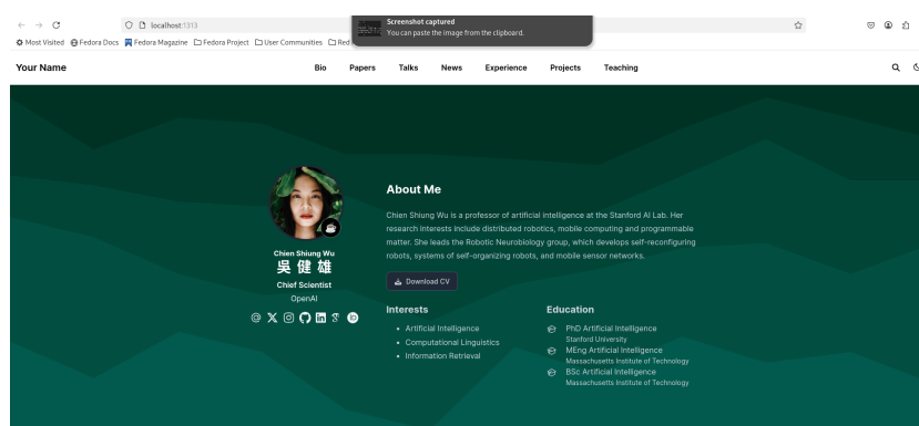
Рис. 3.9: Страница сайта
