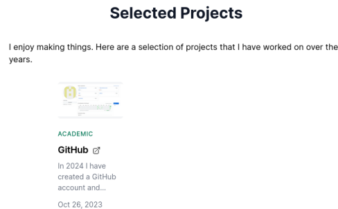
Рис. 3.2: Страница сайта
