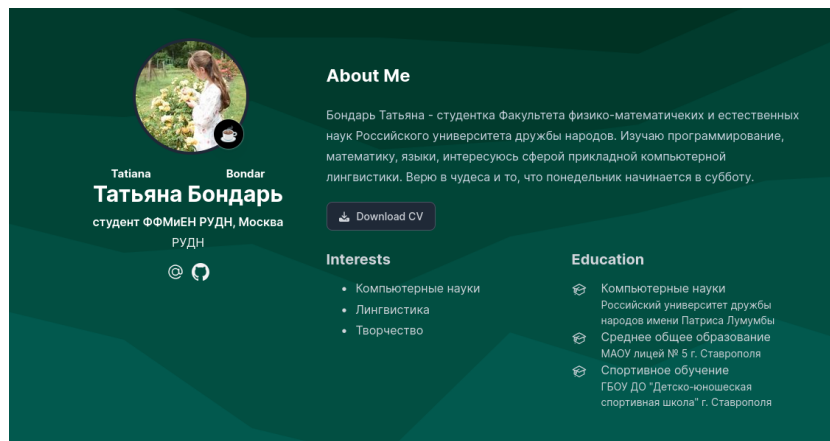
Рис. 3.4: Страница сайта
