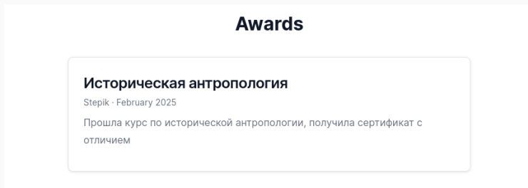
Рис. 5: Страница сайта
