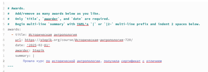
Рис. 3.4: Информация о достижениях
