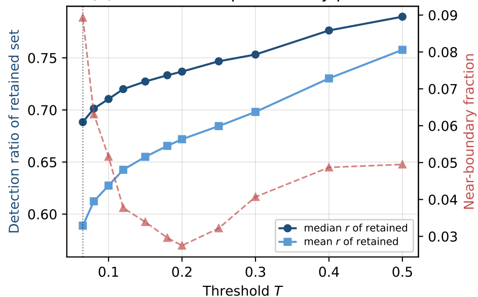
(d) Retained-sample difficulty proxies
