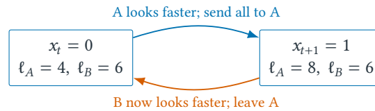
圖 H.3 Endogenous routing feedback。每次 observation 都正確，震盪仍會發生，因為 decision 改變了下一輪被量測的 latency。
