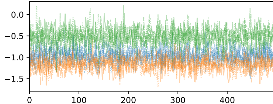
kappa_model
