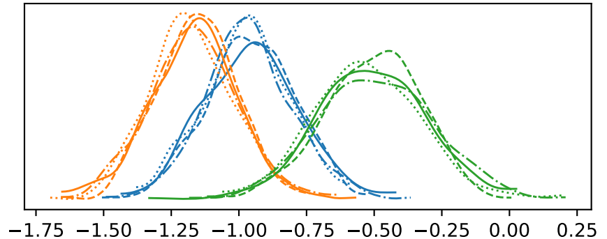
kappa_model
