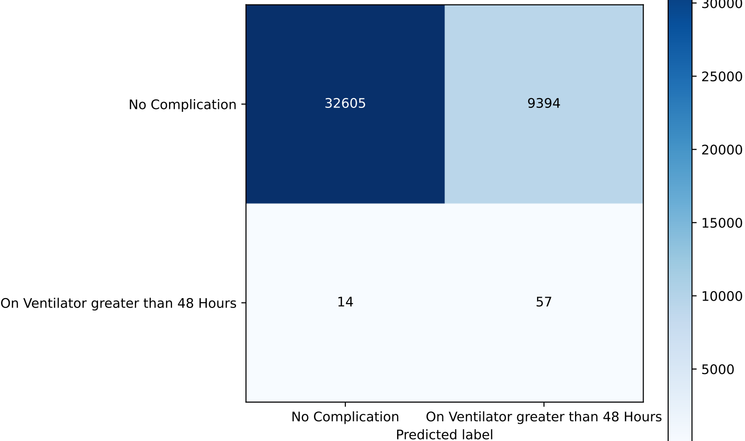
Confusion Matrix - FAILWEAN - Best AUC Model: lr (AUC = 0.84)
