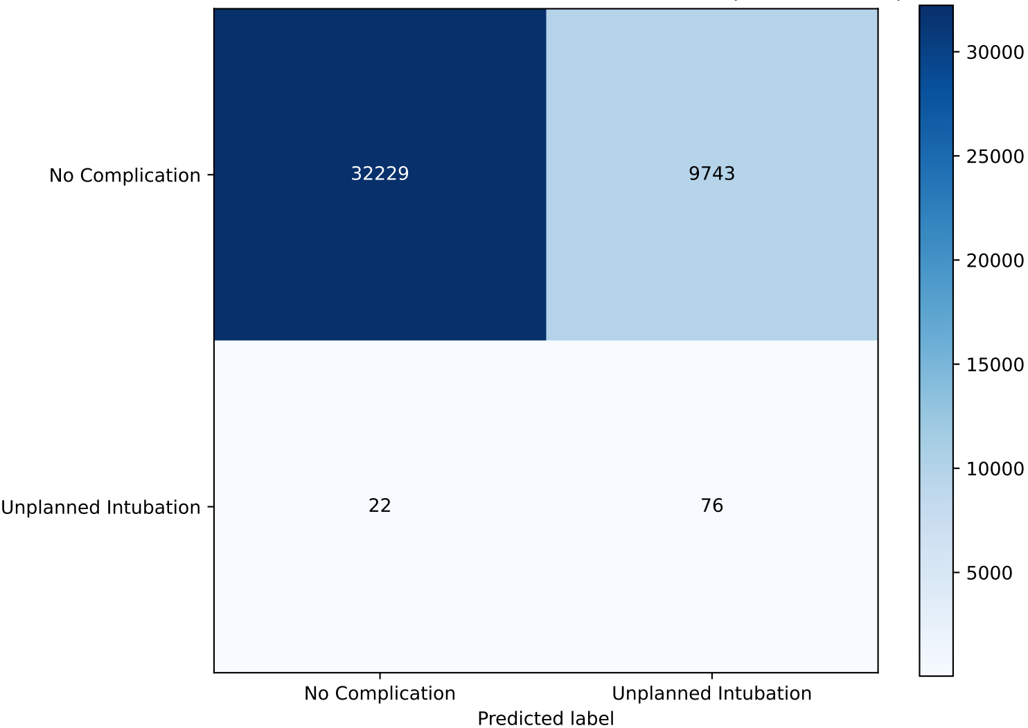
Confusion Matrix - REINTUB - Best AUC Model: Ir (AUC = 0.8377)
