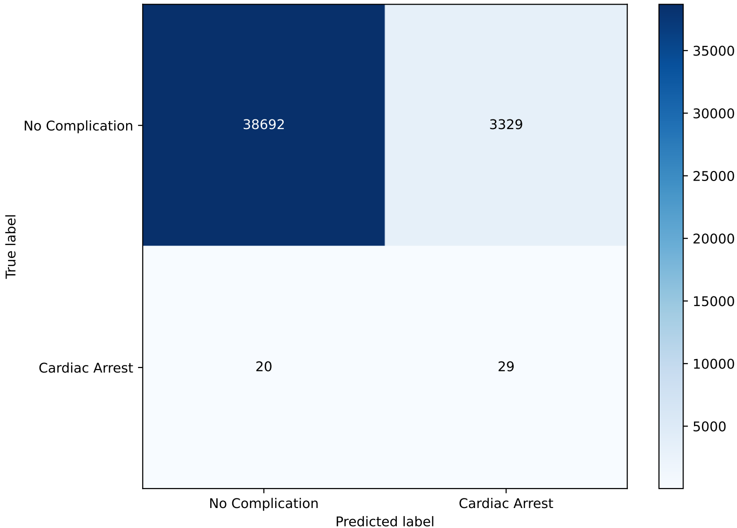
Confusion Matrix - CDARREST - Best AUC Model: nb (AUC = 0.8675)
