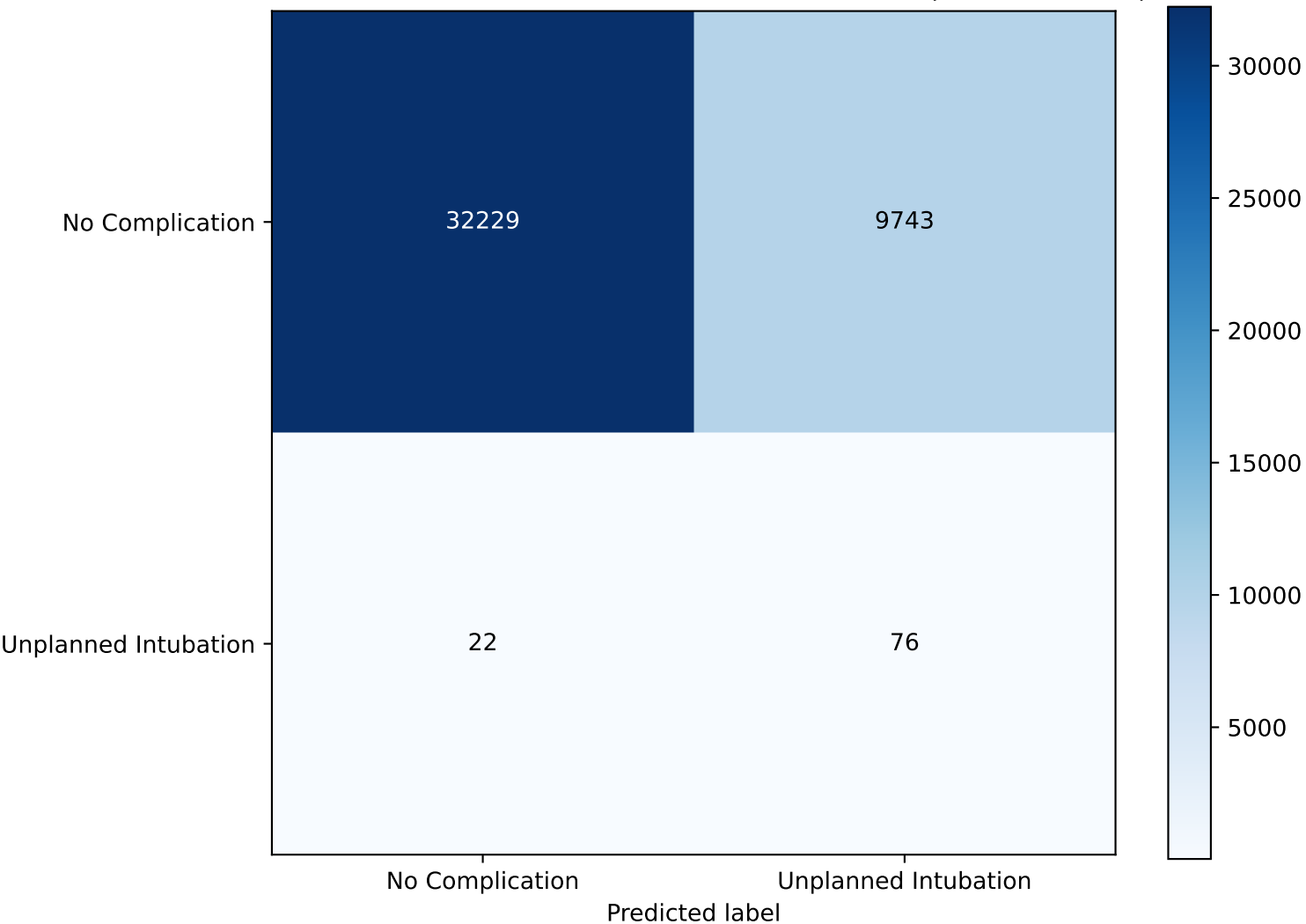
Confusion Matrix - REINTUB - Best AUC Model: lr (AUC = 0.8377)
