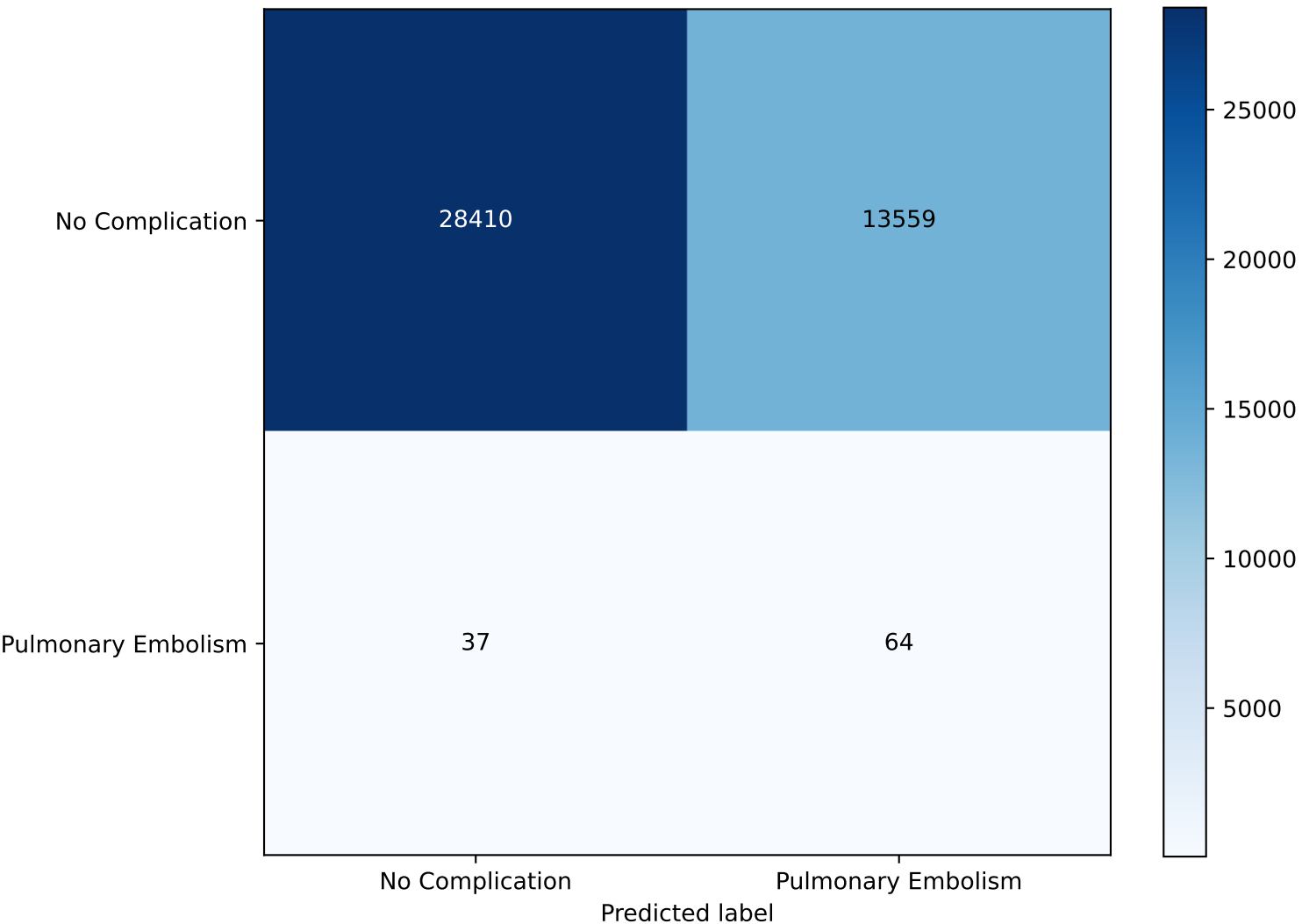
Confusion Matrix - PULEMBOL - Best AUC Model: lr (AUC = 0.7131)
