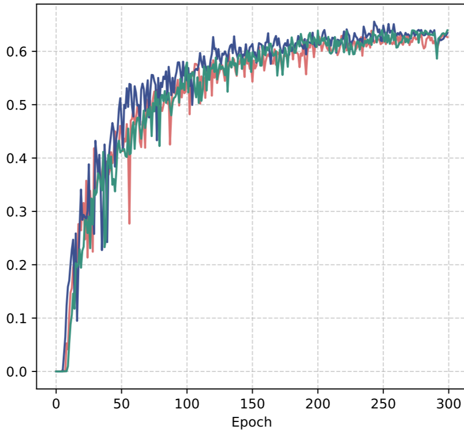
mAP50-95
