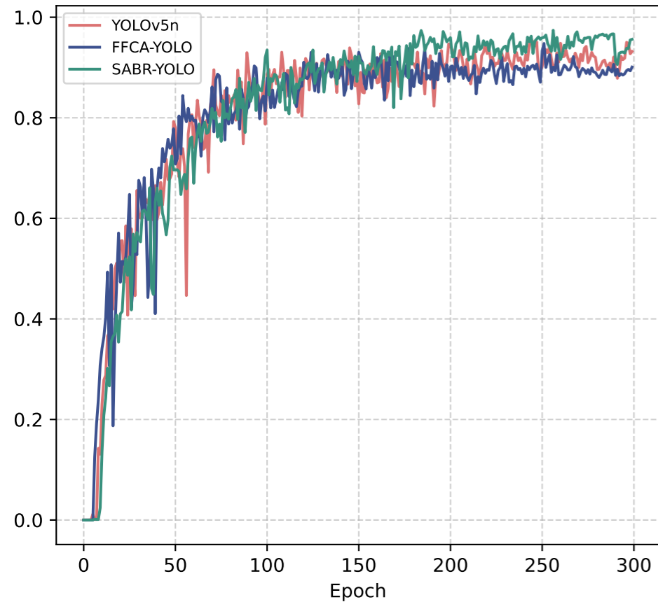
mAP50
