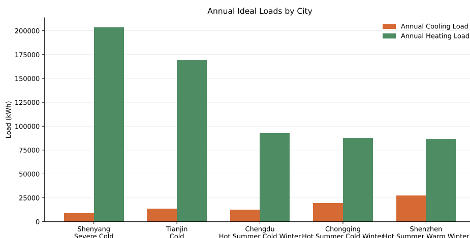
图 5: 五城市年冷负荷与年热负荷比较
