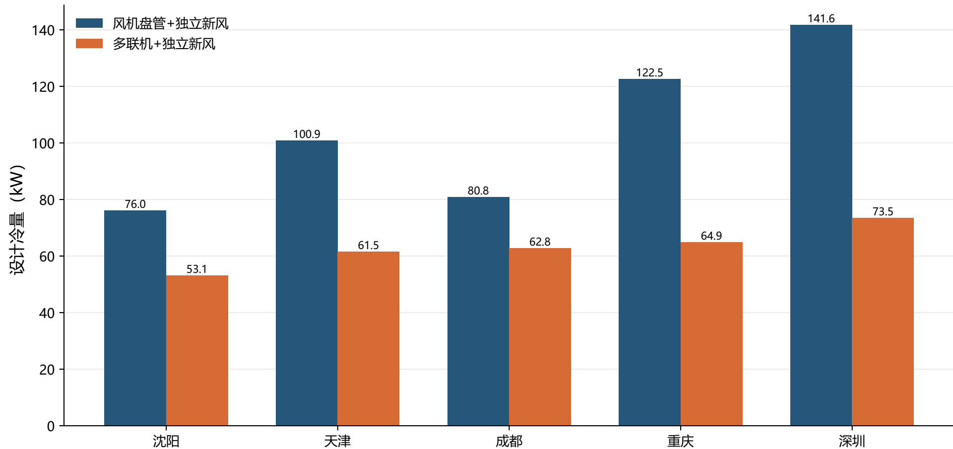
五城市两类系统设计冷量
