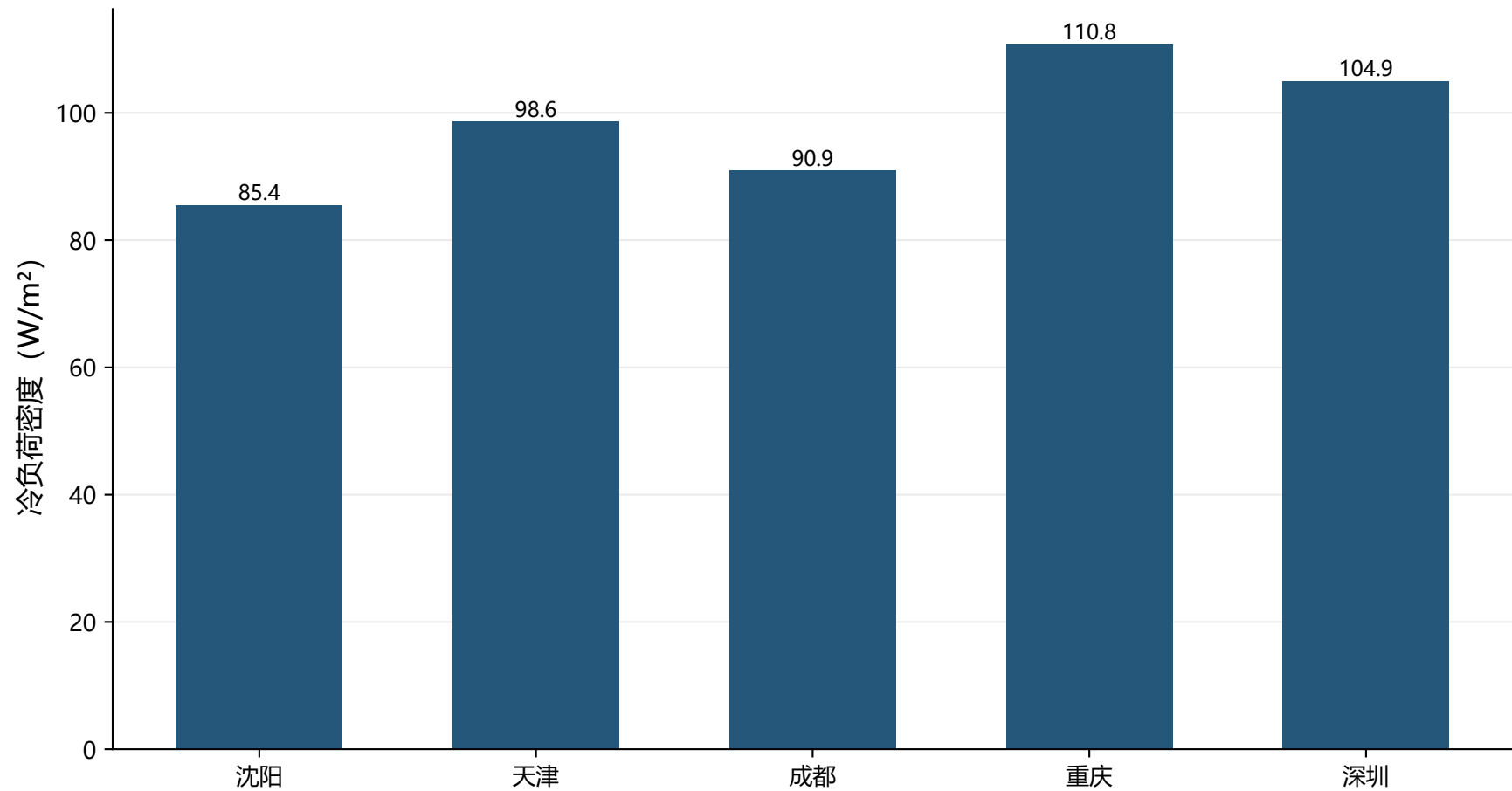
五城市设计峰值冷负荷密度
