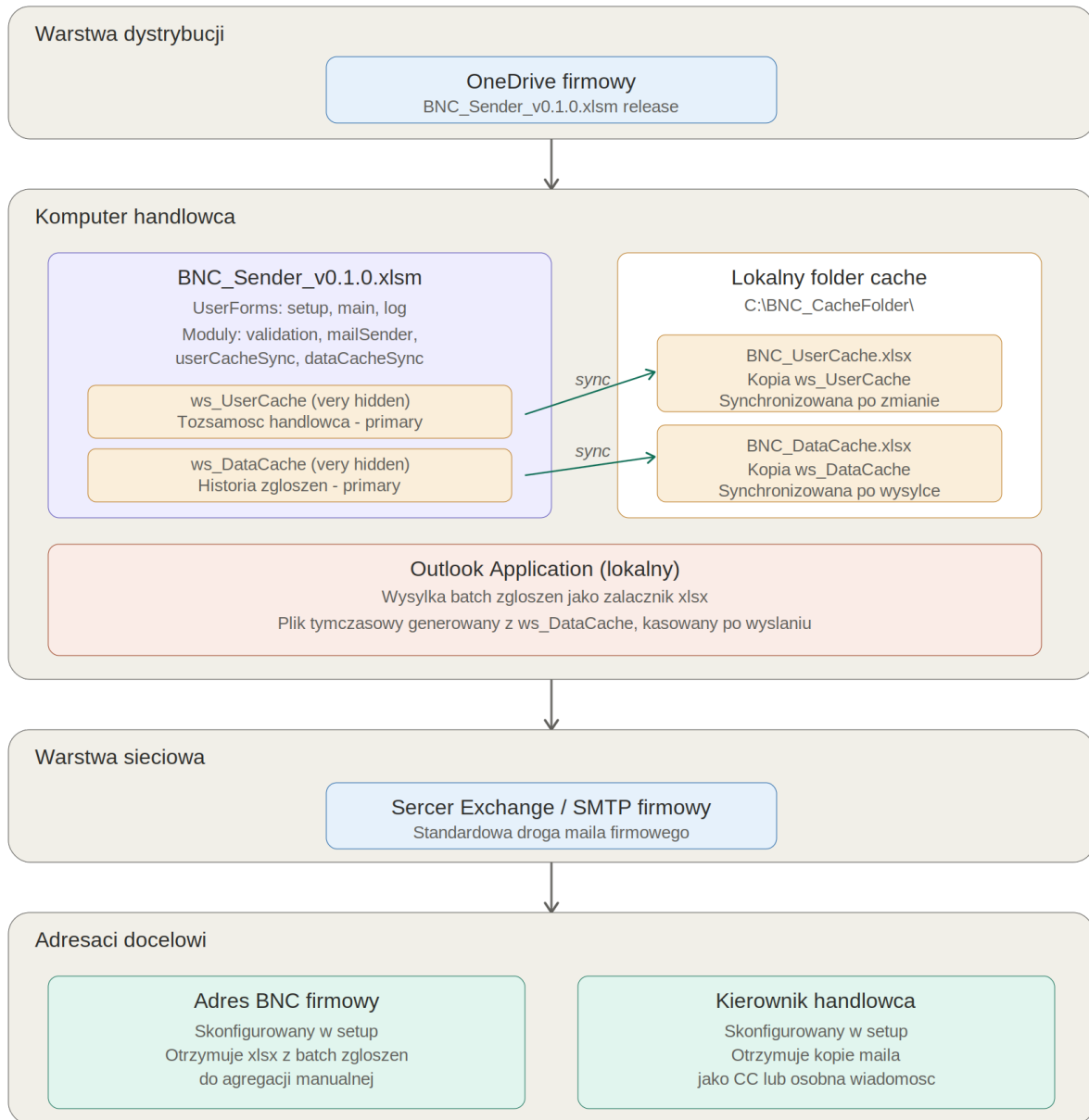
Diagram: Architektura systemu
